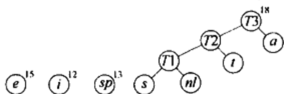
图 10-16 第三次合并后的哈夫曼算法
