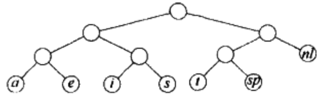
图 10-10 稍微好一些的树
