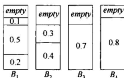
图 10-24 对 0.2, 0.5, 0.4, 0.7, 0.1, 0.3, 0.8 的首次适合装箱
