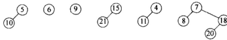
图 11-16 在删除最小元素(3)后的懒惰二项队列
