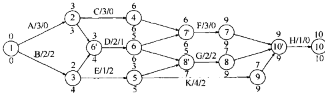
图 9-37 最早完成时间、最晚完成时间和松弛时间
