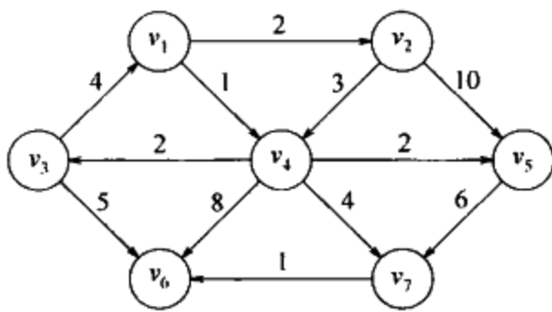
图 9-20 有向图 G
