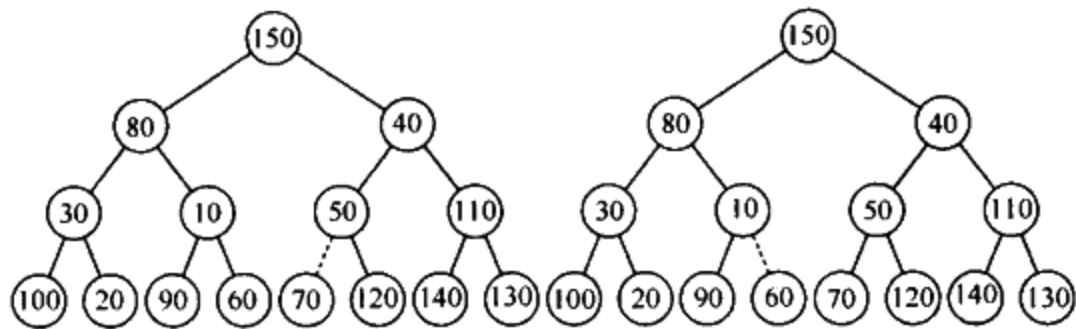
图 6-16 左: 在 percolateDown(6)后; 右: 在 percolateDown(5)后
