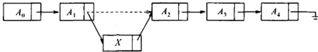
图 3-3 向链表插入
