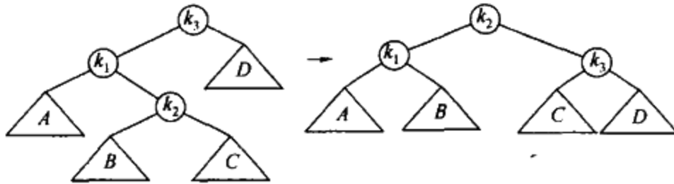
图 4-42 双旋转
