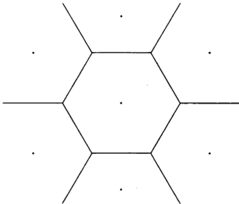
图 10-77 Voronoi 图
