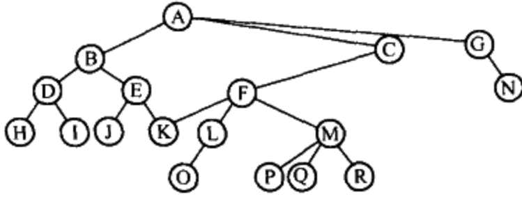
图 4-72 练习 4.44 中的树
