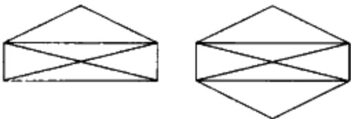
图 9-68 三幅图形
