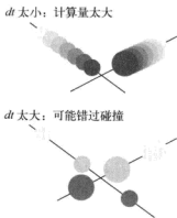
图 6.0.2 驱动模拟的主要问题
