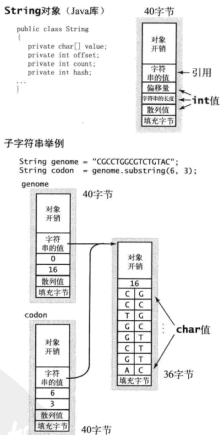
图 1.4.10 一个 String 对象和一个子字符串
