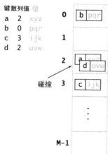
图 3.4.1 散列表的核心问题
