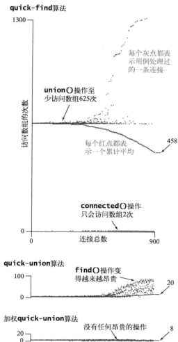
图 1.5.10 所有操作的总成本（625 个触点，另见彩插）
