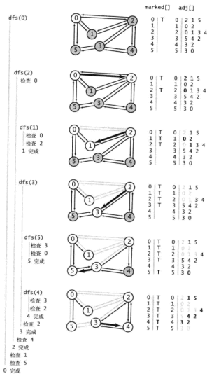
图 4.1.14 使用深度优先搜索的轨迹，寻找所有和顶点 0 连通的顶点（另见彩插）
