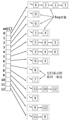
图 4.1.9 邻接表数组示意（无向图）
