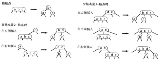
图 3.3.8 在一棵 2-3 树中分解一个 4- 结点的情况汇总
