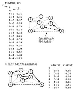
图 4.4.19 含有负权重的边的加权有向图
