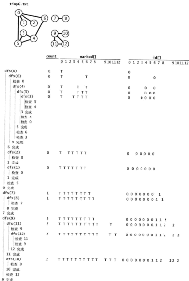
图 4.1.21 使用深度优先搜索的轨迹，寻找所有连通分量
