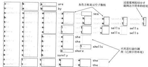
图 5.1.7 三向字符串快速排序的递归调用轨迹（不在子数组较小时切换排序方法）
