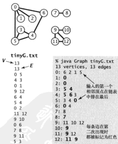
图 4.1.10 由边得到的邻接表（另见彩插）
