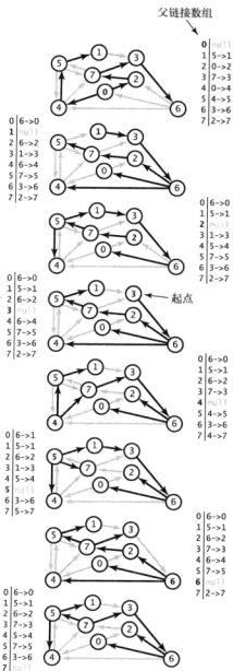
图 4.4.2 最短路径树（另见彩插）
