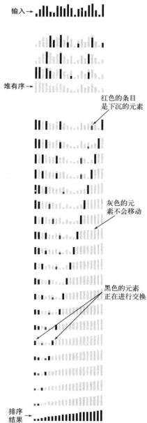
图 2.4.8 堆排序的可视轨迹 (另见彩插)
