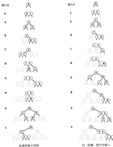
图 3.3.10 2-3 树的构造轨迹
