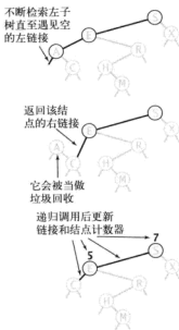
图 3.2.12 删除二叉查找树中的最小结点
