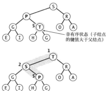
图 2.4.3 由下至上的堆有序化 (上浮)
