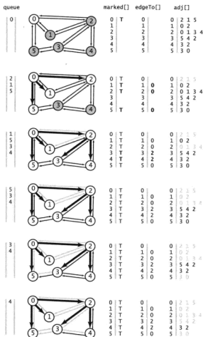
图 4.1.18 使用广度优先搜索的轨迹，寻找所有起点为 0 的路径（另见彩插）
