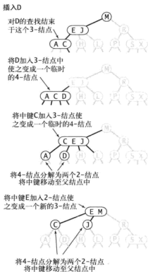
427 图 3.3.6 向一个父结点为3-结点的3-结点中插入新键
