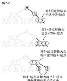
图 3.3.5 向一个父结点为2-结点的3-结点中插入新键
