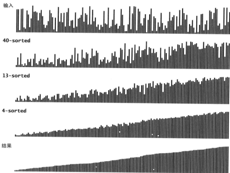
图 2.1.4 希尔排序的可视轨迹
