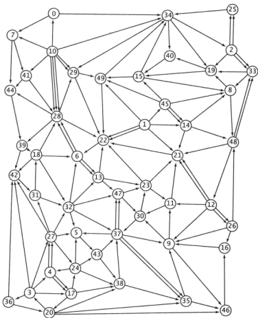
图 4.2.17 这幅有向图中含有多少个强连通分量
