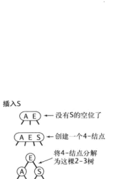
图 3.3.4 向一棵只含有一个3-结点的树中插入新键
