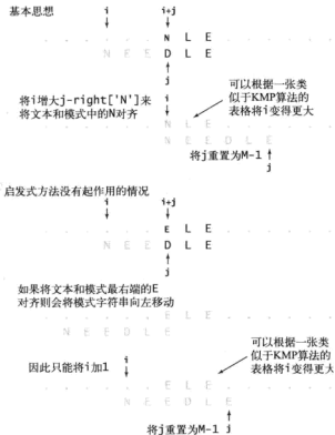
图 5.3.13 启发式的处理不匹配的字符 (不匹配的字符包含在模式字符串中)
