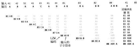
图 5.15.19 LZW 算法对 41 42 52 41 43 41 44 81 83 82 88 41 80 的展开
