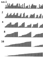
图 2.2.5 自底向上的归并排序的可视轨迹
