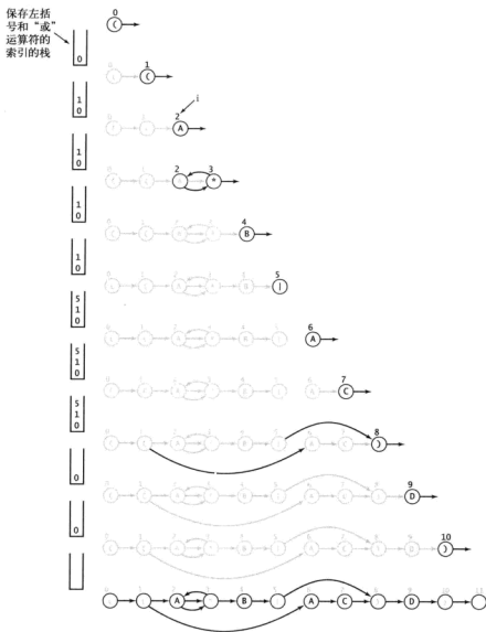
图 5.4.7 构造正则表达式 (A^*B|AC)D 所对应的 NFA
