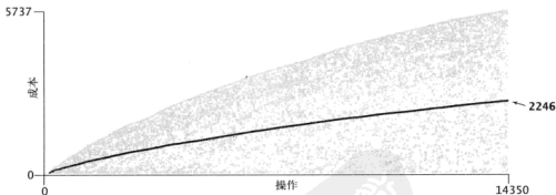
图 3.1.3 使用 SequentialSearchST ，运行 java FrequencyCounter 8 < tale.txt 的成本
