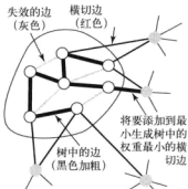
图 4.3.9 最小生成树的 Prim 算法 (另见彩插)
