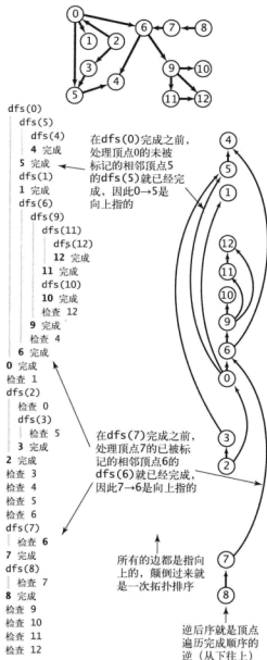
图 4.2.11 有向无环图的逆后序是拓扑排序
