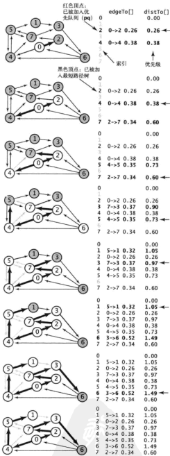
图 4.4.10 Dijkstra 算法的轨迹 (另见彩插)
