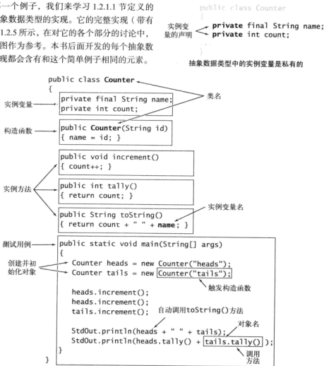
图 1.2.5 详解数据类型的定义类
