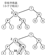
图 2.4.4 由上至下的堆有序化 (下沉)
