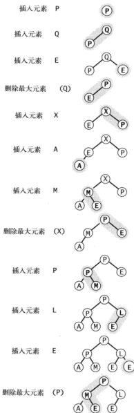
图 2.4.6 在堆上的优先队列操作
