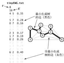
图 4.3.1 一幅加权无向图和它的最小生成树
