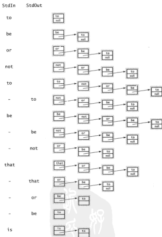
图 1.3.9 stack 的开发用例的轨迹
