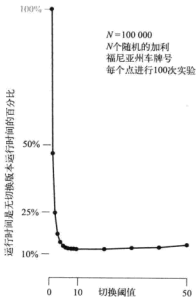
图 5.1.13 高位优先的字符串排序算法中切换小型子数组的排序方法的实际效果
