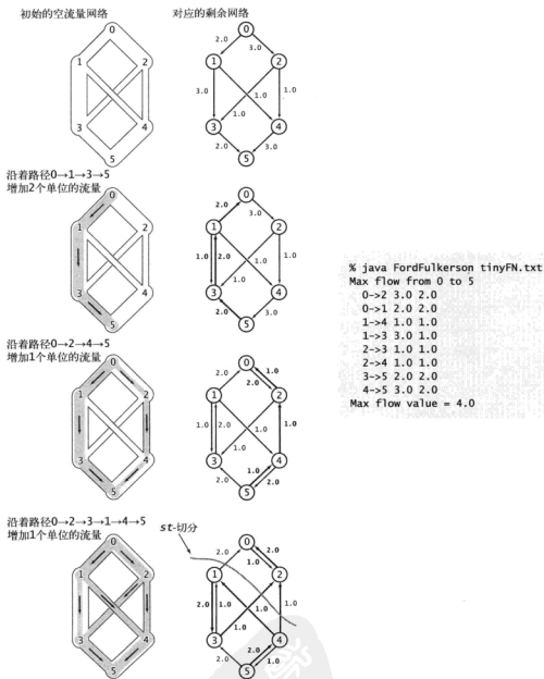
899 图 6.0.23 最短增广路径的 FordFulkerson 算法的轨迹
