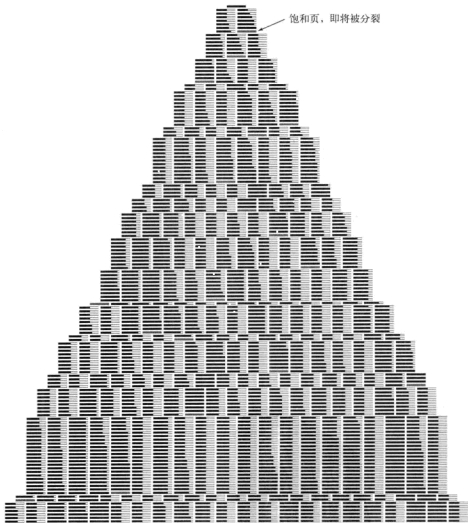
图 6.0.11 构造一棵庞大的 B-树
