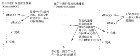
图 4.2.15 Kosaraju 算法的正确性证明
