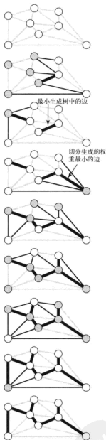
图 4.3.6 贪心最小生成树算法 (另见彩插)
