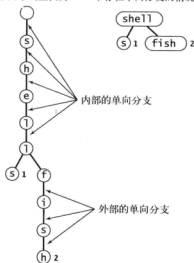
图 5.2.9 消除单词查找树中的单向分支
