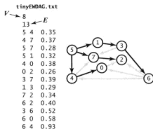
图 4.4.12 一幅无环加权有向图 and 它的一棵最短路径树
