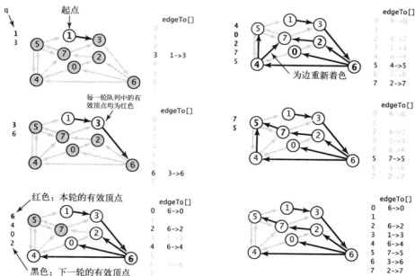
图 4.4.22 Bellman-Ford 算法的轨迹 (另见彩插)
