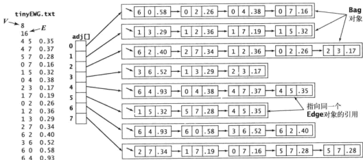
图 4.3.7 加权无向图的表示
