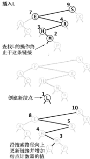
图 3.2.5 二叉查找树的插入操作
