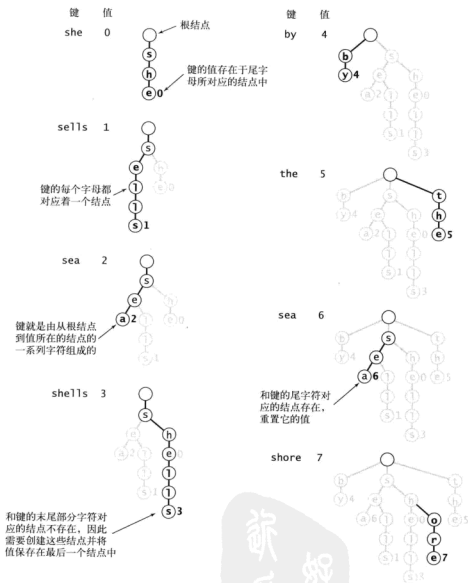
图 5.2.3 标准索引用例中单词查找树的构造轨迹
