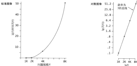
图 1.4.2 实验数据 (ThreeSum.count() 的运行时间) 的分析
