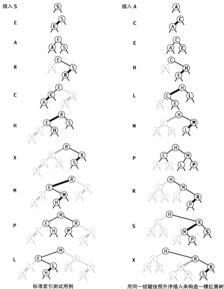
图 3.3.24 红黑树的构造轨迹 (另见彩插)
