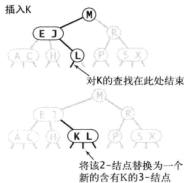
图 3.3.3 向 2- 结点中插入新的键
