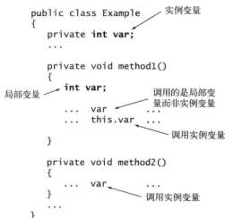
实例方法中的实例变量和局部变量的作用范围
