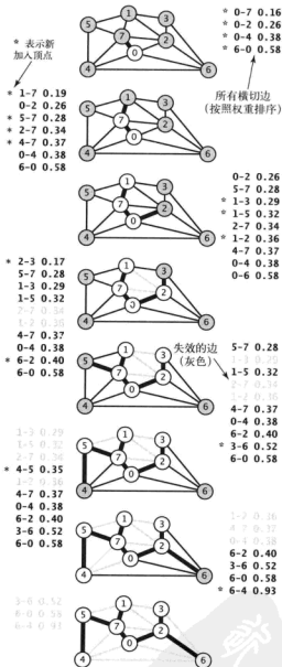
图 4.3.10 Prim 算法的轨迹（延时实现，另见彩插）
