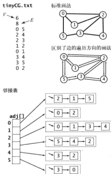
图 4.1.13 一幅连通的无向图
