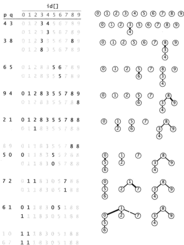
图 1.5.5 quick-union 算法的轨迹 (以及相应的森林)
