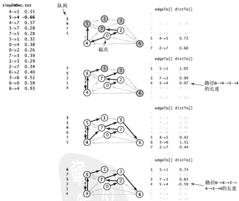
图 4.4.25 Bellman-Ford 算法的轨迹 (含有负权重环的图, 另见彩插)
