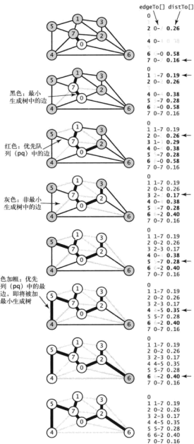
4.3.12 Prim 算法的轨迹（即时版本，另见彩插）
