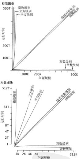
图 1.4.5 典型的生长数量级函数
