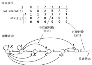
图 5.3.6 和模式字符串 A B A B A C 对应的确定有限状态自动机
