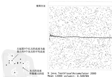
图 1.2.8 可视化累加器图像（另见彩插）
