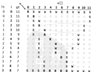
三向切分的轨迹（每次迭代循环之后的数组内容）
