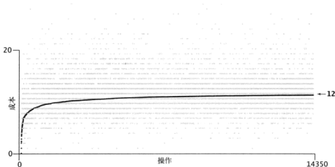
图 3.3.29 使用 RedBlackBST，运行 java FrequencyCounter 8 &lt; tale.txt 的成本
