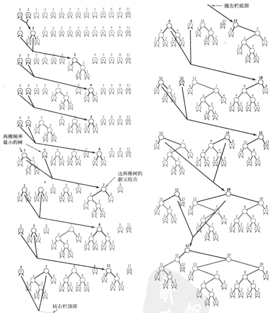
图 5.5.12 构造一棵霍夫曼编码单词查找树
