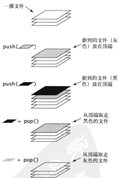
图 1.3.3 下压栈的操作
