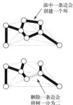
图 4.3.3 树的基本性质
