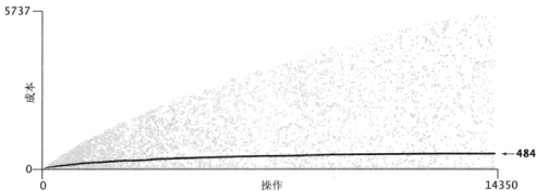
图 3.1.4 使用 BinarySearchST, 运行 java FrequencyCounter 8 &lt; tale.txt 的成本
