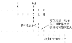
图 5.3.12 启发式的处理不匹配的字符（不匹配的字符不包含在模式字符串中）
