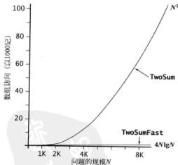
图 1.4.6 解决 2-sum 和 3-sum 问题的各种算法的成本
