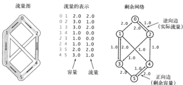
图 6.0.22 网络流问题详解
