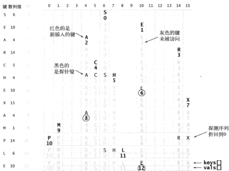
图 3.4.6 标准索引用例使用的基于线性探测的符号表的轨迹（另见彩插）
