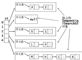
图 3.4.3 标准索引用例使用基于拉链法的散列表
