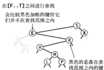
二叉查找树的范围查找
