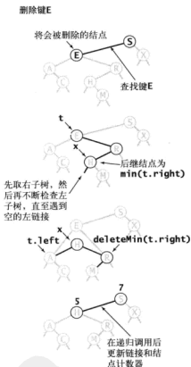
图 3.2.13 二叉查找树中的删除操作
