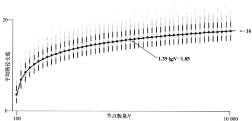
图 3.2.14 一棵随机构造的二叉查找树中由根到达任意结点的平均路径长度（另见彩插）
