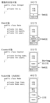
图 1.4.8 典型对象的内存需求
