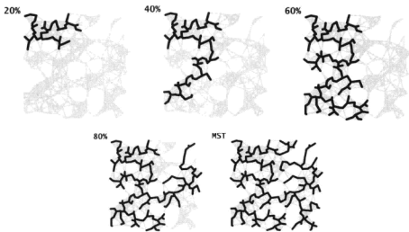
图 4.3.13 Prim 算法（250 个顶点）
