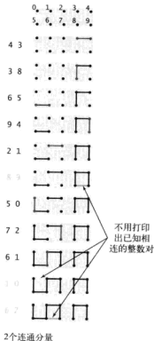
图 1.5.1 动态连通性问题 (另见彩插)
