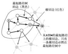
图 4.4.9 Dijkstra 的最短路径算法 (另见彩插)
