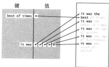
图 6.0.14 理想化的一张文本字符串索引表
