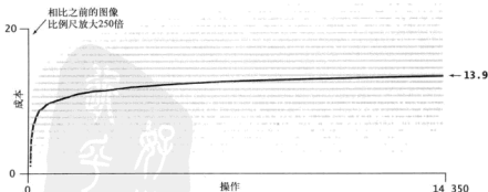
图 3.2.9 使用二叉查找树，运行 java FrequencyCounter 8 < tale.txt 的成本
