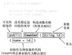
图 1.2.6 详解构造函数
