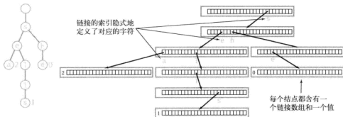
图 5.2.4 单词查找树的表示 ( R=26 )
