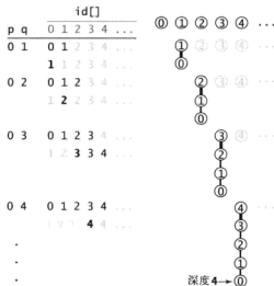
图 1.5.6 quick-union 算法的最坏情况
