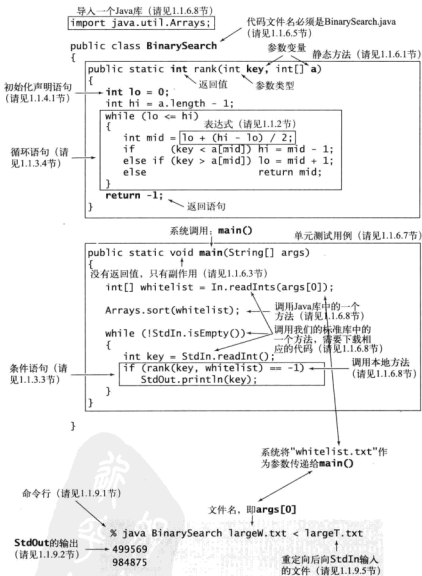
图 1.1.1 Java 程序及其命令行的调用
