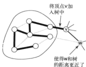
图 4.3.11 Prim 算法的即时实现
