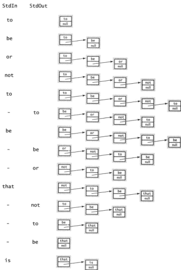
图 1.3.10 Queue 的开发用例的轨迹
