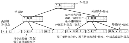
图 6.0.8 详解用一棵 B-树表示的键集 ( M=6 )
