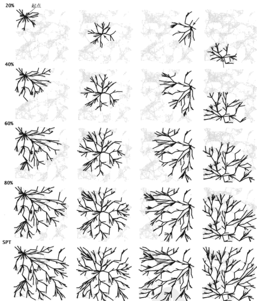
图 4.4.11 Dijkstra 算法 (250 个顶点, 不同的起点)
