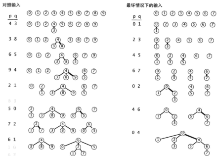
图 1.5.8 加权 quick-union 算法的轨迹 (森林)
