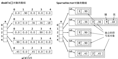
图 3.5.4 稀疏矩阵的表示
