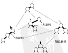
图 3.3.23 红黑树中红链接向上传递 (另见彩插)
