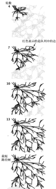
图 4.4.23 Bellman-Ford 算法（250 个顶点）（另见彩插）
