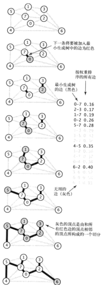
图 4.3.14 Kruskal 算法的轨迹 (另见彩插)
