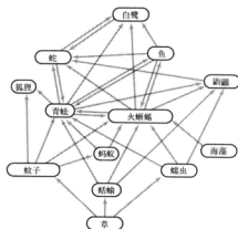
图 4.2.14 一幅表示食物链的有向图的一小部分
