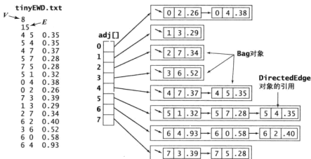
图 4.4.4 加权有向图表示
