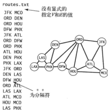
图 4.1.22 符号图示例（边的列表）
