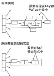
图 3.5.1 拉链法的内存使用情况
