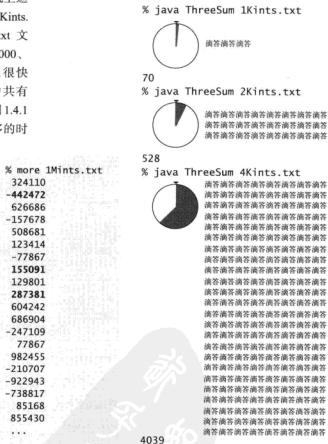
图 1.4.1 记录一个程序的运行时间
