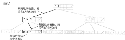
图 6.0.9 在由 B-树表示的键集中进行查找 ( M=6 )
