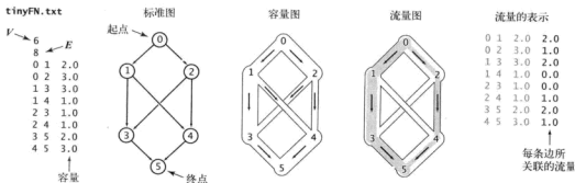
图 6.0.19 网络流问题详解
