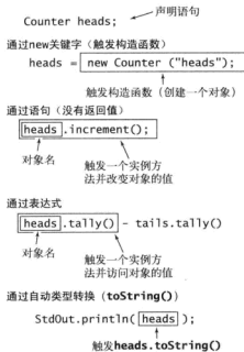
图 1.2.3 触发实例方法的各种方式
