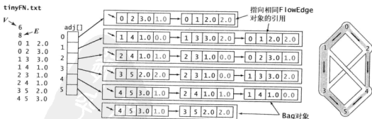
图 6.0.20 流量网络的表示
