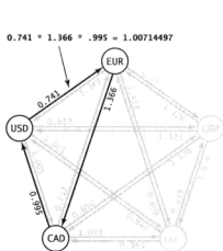
图 4.4.26 一次套汇机会
