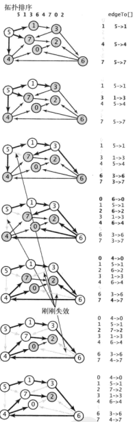
图 4.4.14 无环图中的最长路径算法（另见彩插）
