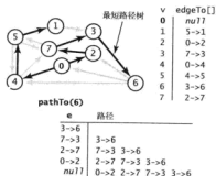
图 4.4.8 pathTo() 方法的计算轨迹
