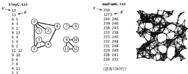
图 4.1.8 Graph 的构造函数的输入格式 (两个示例)
