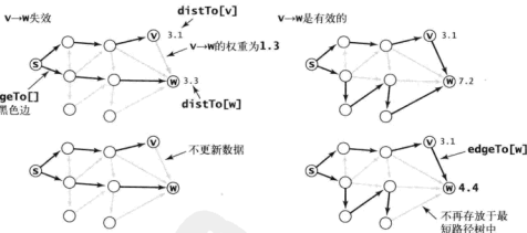
图 4.4.6 边的松弛的两种情况 (另见彩插)
