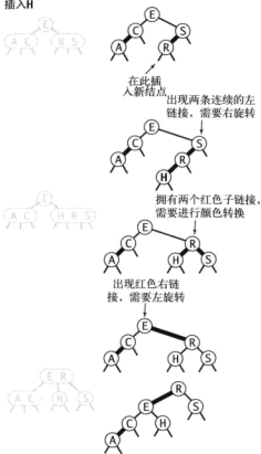
图 3.3.22 向树底部的 3- 结点插入一个新键 (另见彩插)
