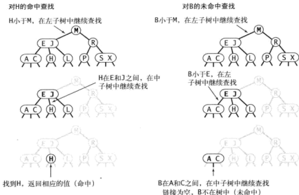
图 3.3.2 2-3 树中的查找命中（左）和未命中（右）
