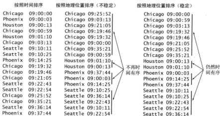
图 2.5.1 从另一个键上排序的稳定性
