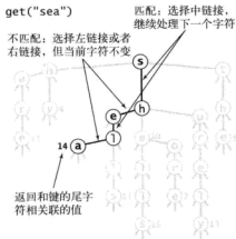
图 5.2.11 三向单词查找树中的查找示例
