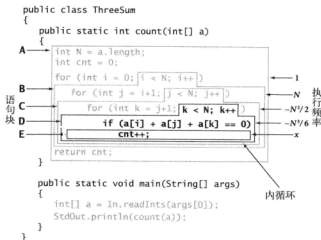
图 1.4.4 程序语句执行频率的分析
