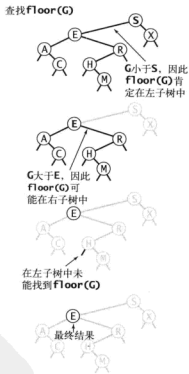
图 3.2.10 计算 floor() 函数
