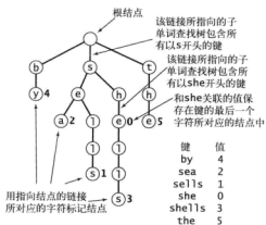
图 5.2.1 单词查找树详解
