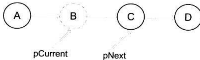
图 3-5 链表示意图
