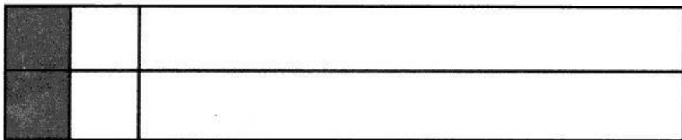
图 4-1 第一块瓷砖竖着放，如图中阴影部分所示
