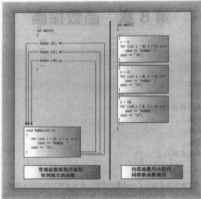
图 8.1 内联函数与常规函数
