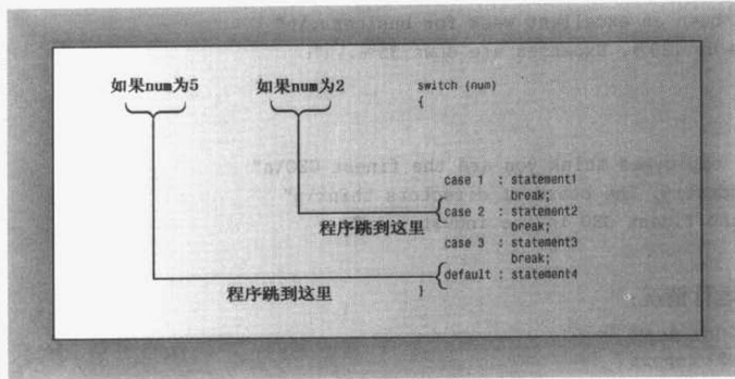
图 6.3 switch 语句的结构
