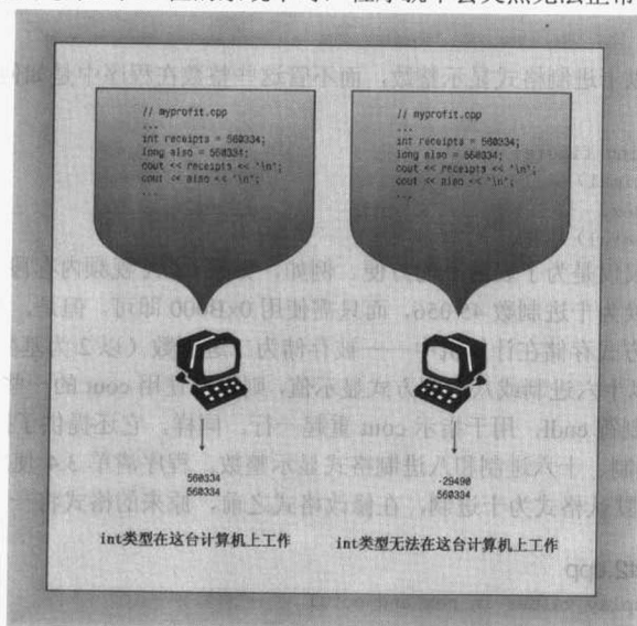
图 3.2 为提高可移植性，请使用 long
