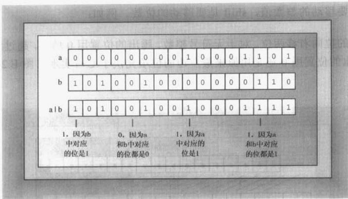
图 E.4 位操作符 OR
