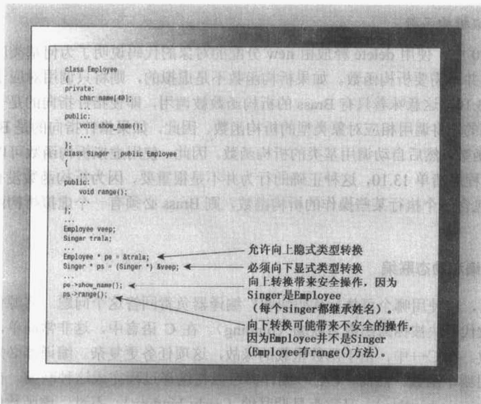
图 13.4 向上强制转换和向下强制转换
