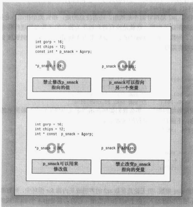
图 7.5 指向 const 的指针和 const 指针
