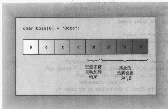
图 4.2 将数组初始化为字符串
