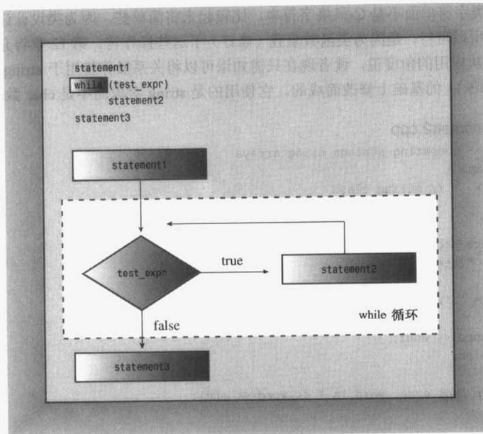
图 5.3 while 循环的结构
