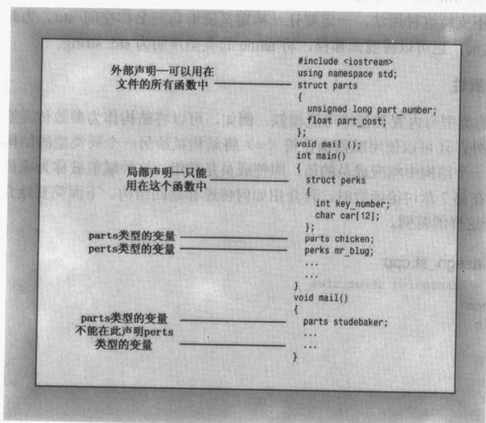
图 4.7 局部结构声明和外部结构声明
