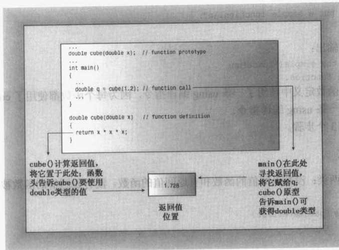
图 7.1 典型的返回值机制
