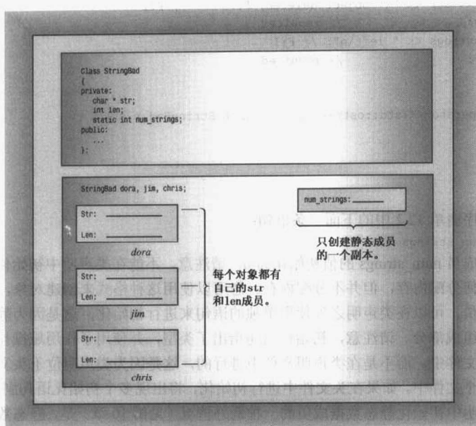
图 12.1 静态数据成员
