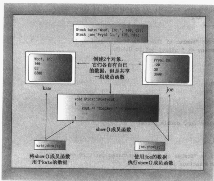
图 10.2 对象、数据和成员函数
