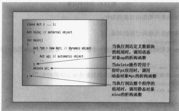
图 12.4 调用析构函数
