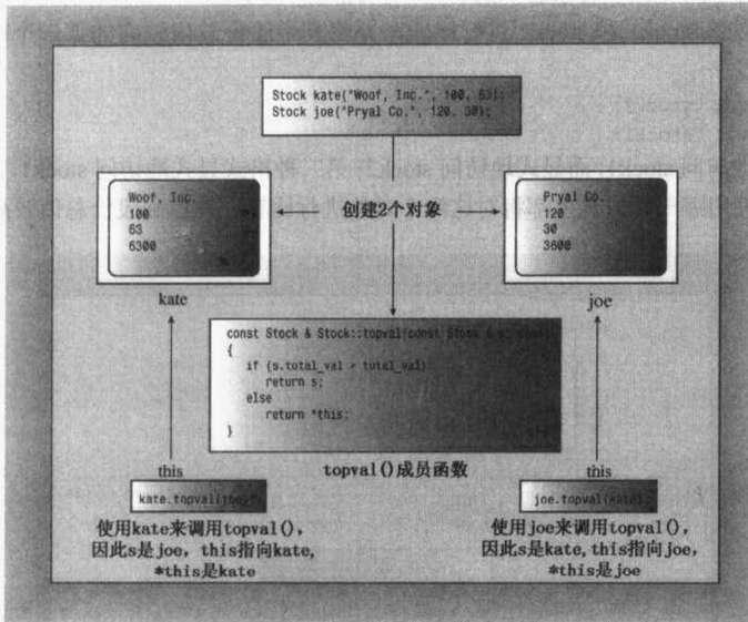
图 10.4 this 指向调用对象
