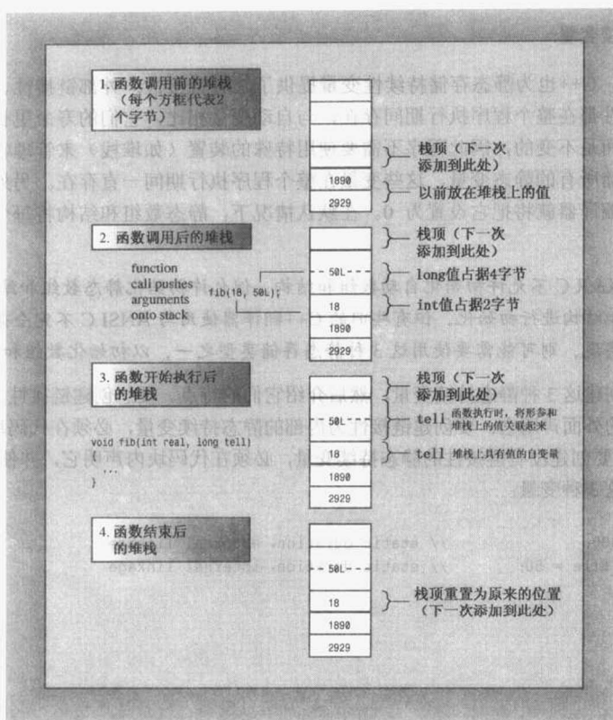
图 9.3 使用堆栈传递参数
