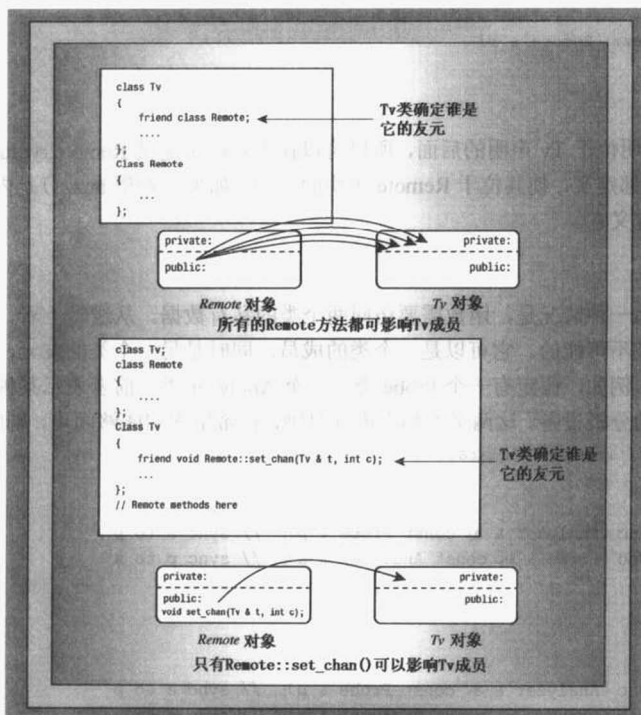
图 15.1 类友元与类成员友元
