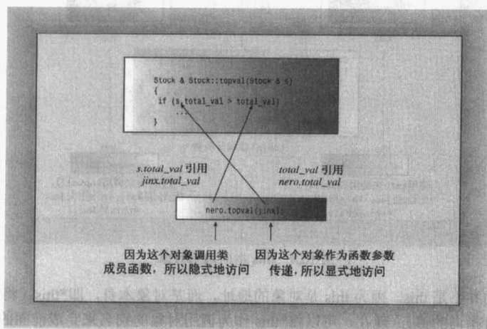
图 10.3 使用成员函数访问两个对象
