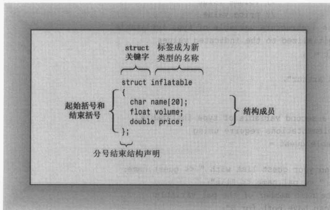
图 4.6 结构描述的组成部分
