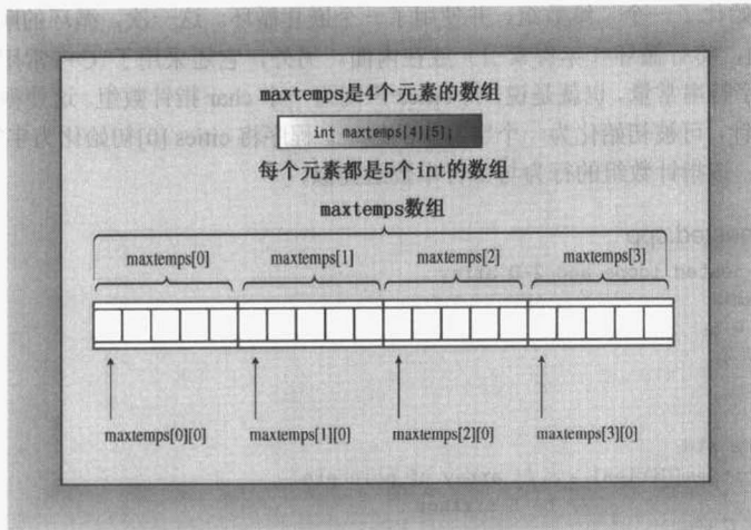
图 5.5 由数组组成的数组
