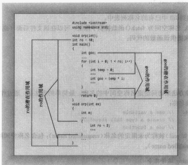
图 9.6 潜在作用域和作用域
