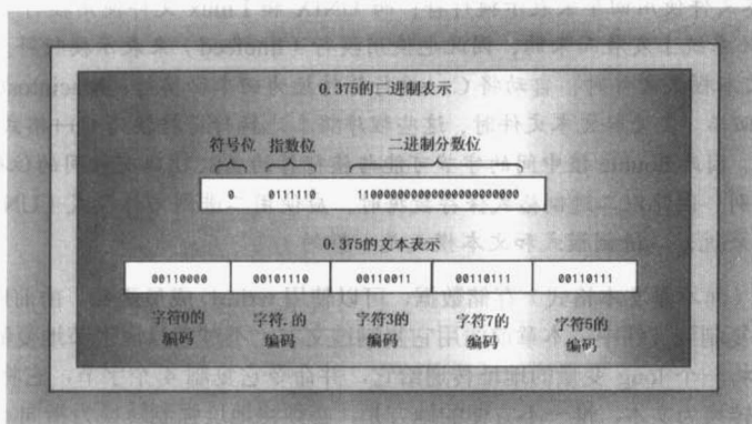
图 17.7 浮点数的二进制表示和文本表示
