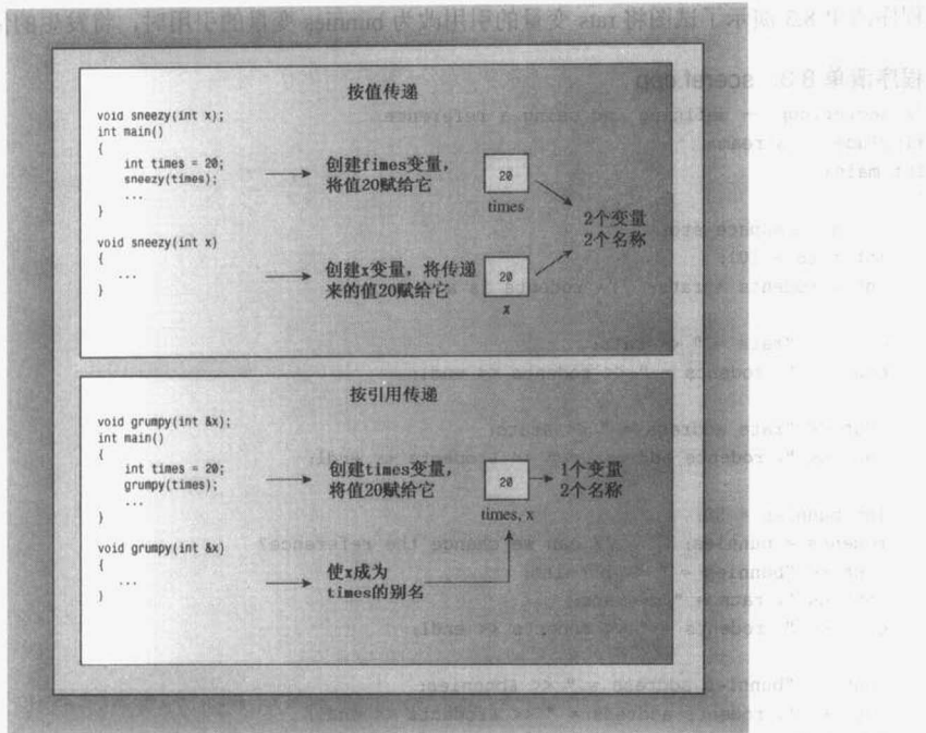
图 8.2 按值传递和按引用传递
