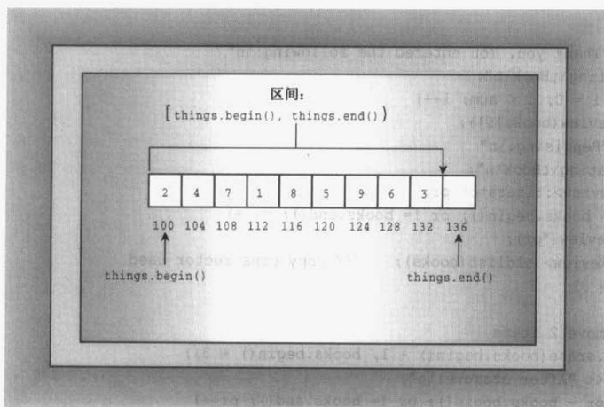
图 16.3 STL 的区间概念
