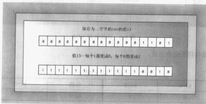
图 E.3 按位非操作符
