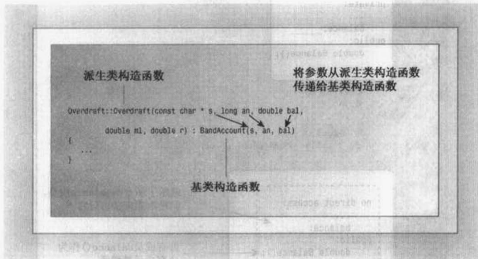
图 13.2 将参数传递给基类构造函数
