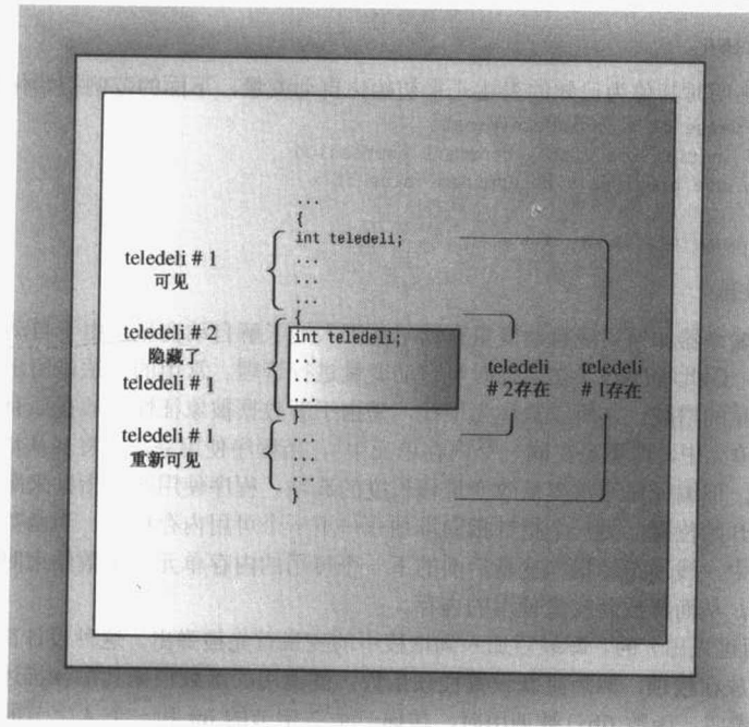
图 9.2 代码块和作用域
