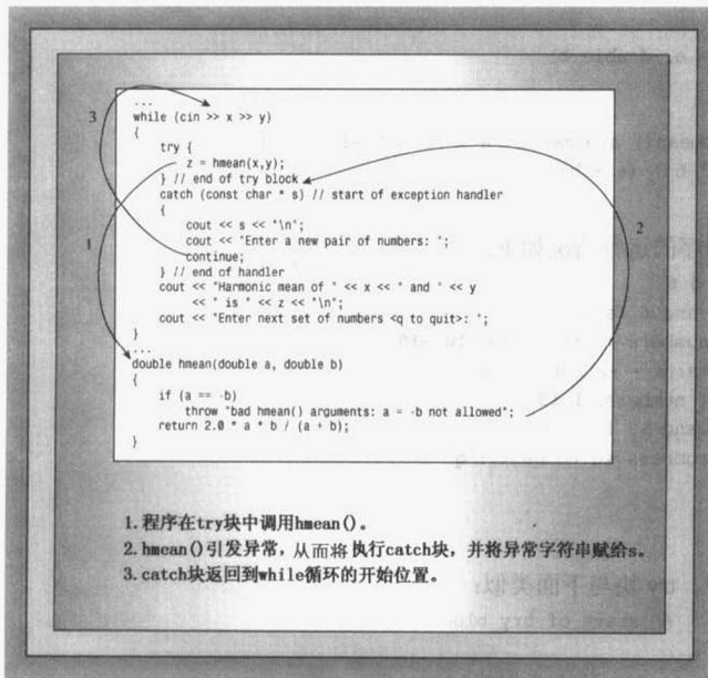
图 15.2 出现异常时的程序流程
