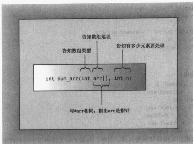
图 7.4 告知函数有关数组的信息
