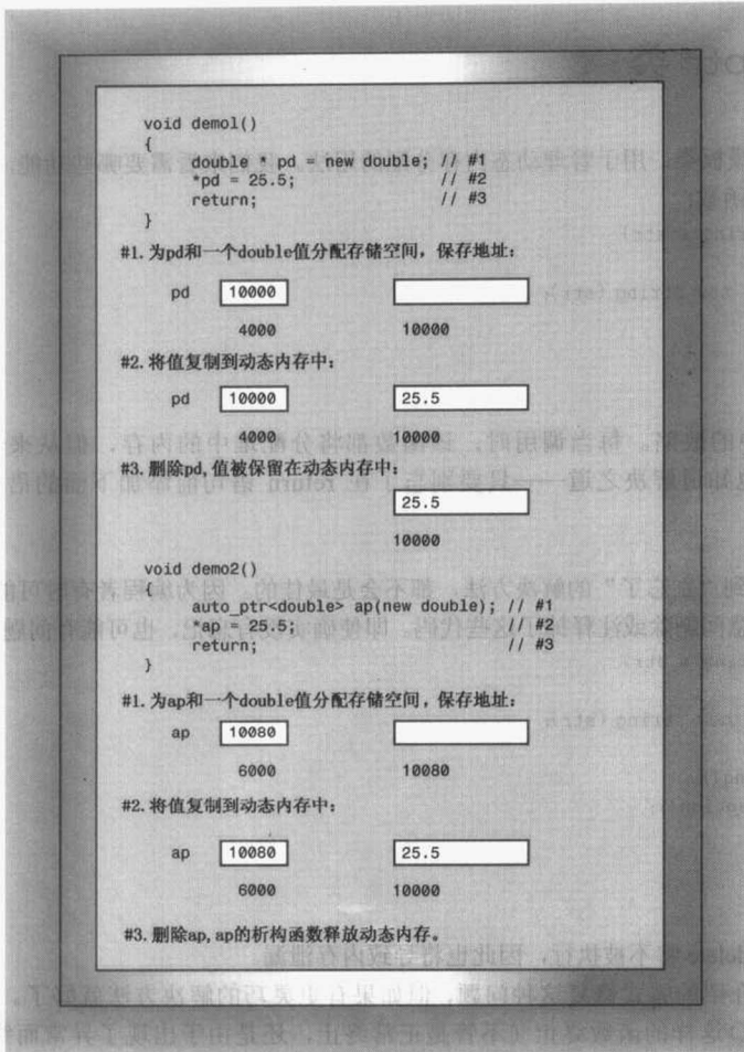
图 16.2 常规指针与 auto_ptr
