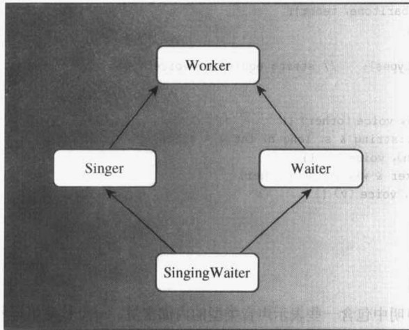
图 14.3 祖先相同的 MI
