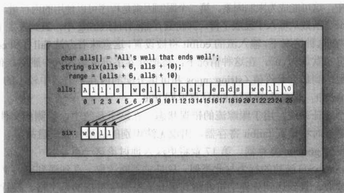
图 16.1 使用区间的 string 构造函数
