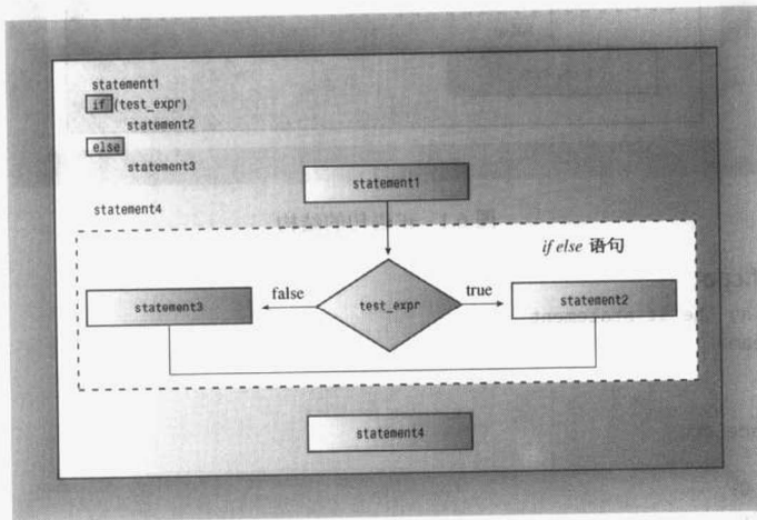
图 6.2 if else 语句的结构
