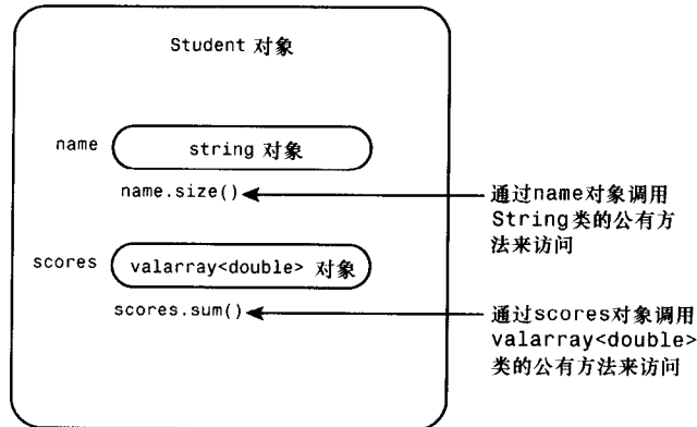
图 14.1 对象中的对象：包含
