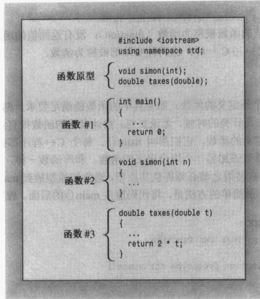
图 2.8 函数定义在文件中依次出现
