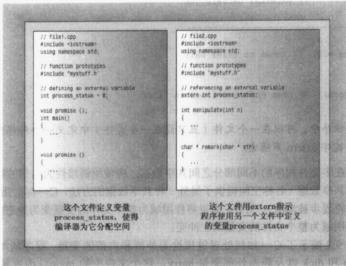
图 9.4 定义声明和引用声明
