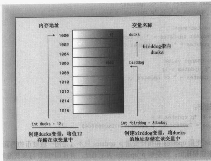
图 4.9 指针存储地址
