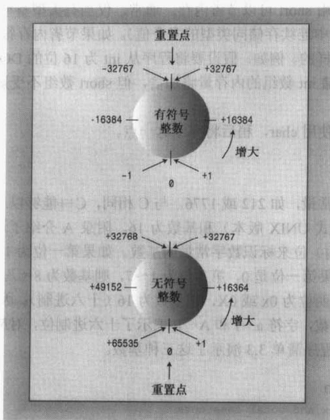
图 3.1 典型的整型溢出行为
