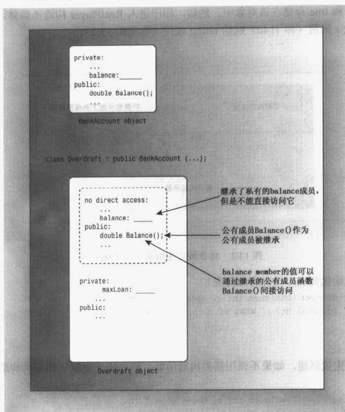
图 13.1 基类对象和派生类对象
