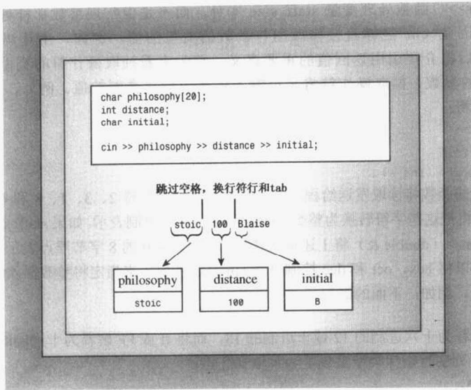
图 17.5 cin&gt;&gt;跳过空白
