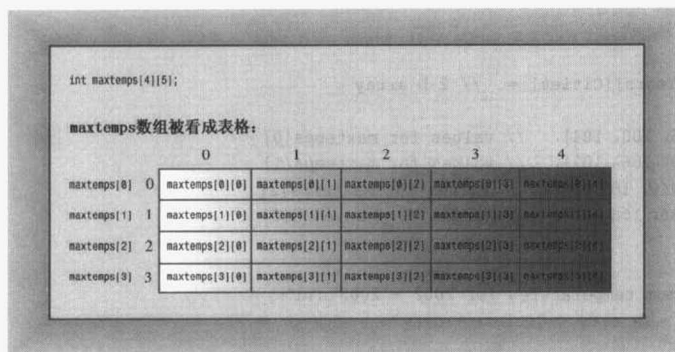
图 5.6 使用下标访问数组元素
