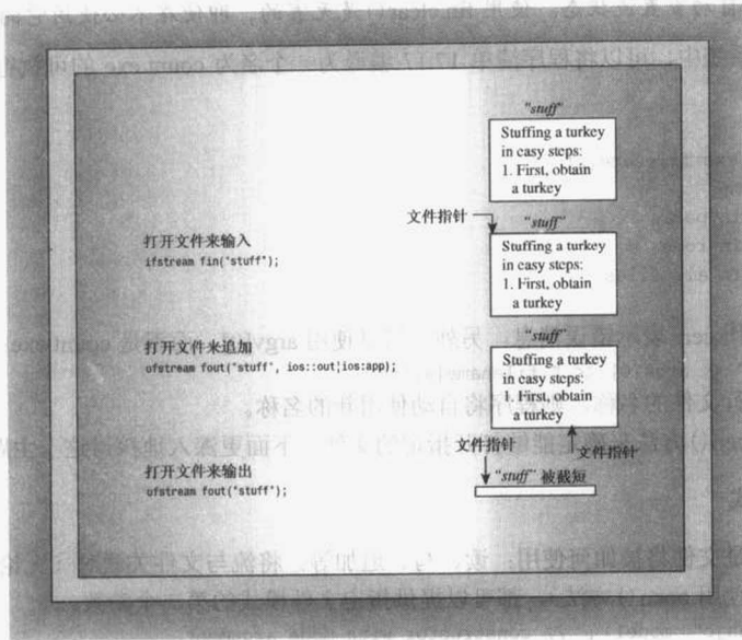
图 17.6 一些文件打开模式
