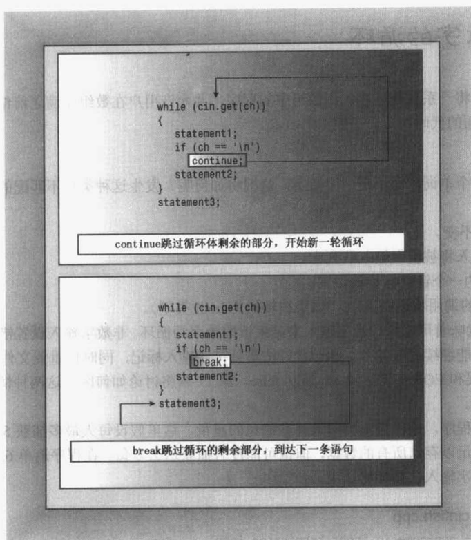
图 6.4 break 和 continue 语句的结构
