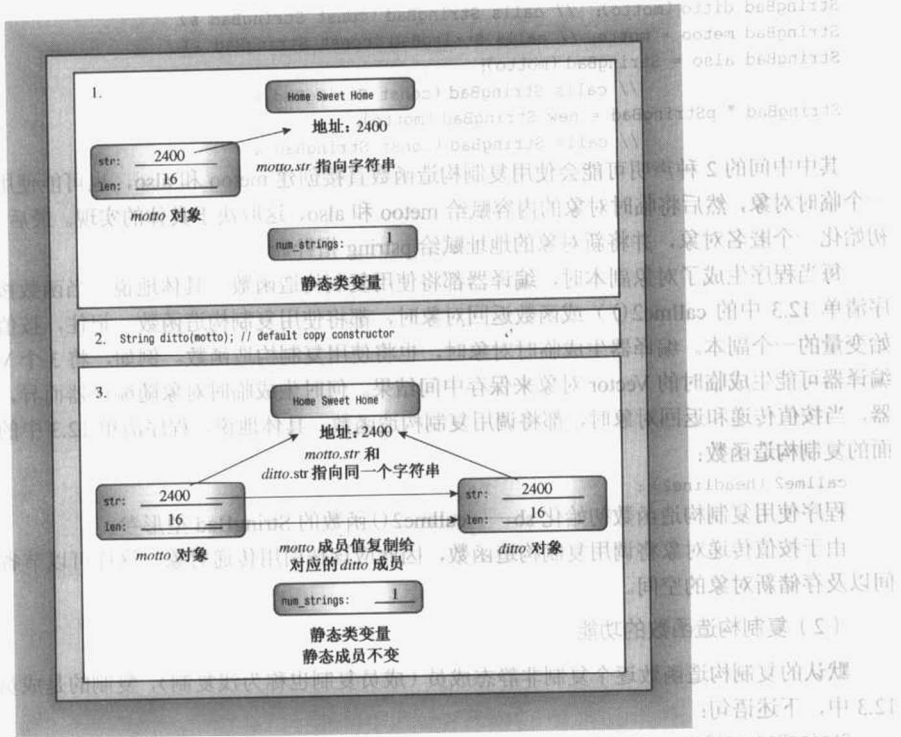
图 12.2 逐个复制成员
