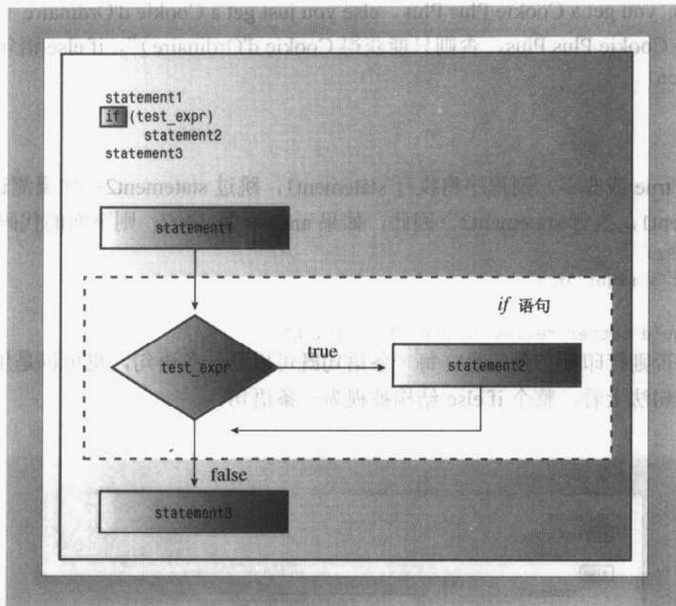
图 6.1 if 语句的结构
