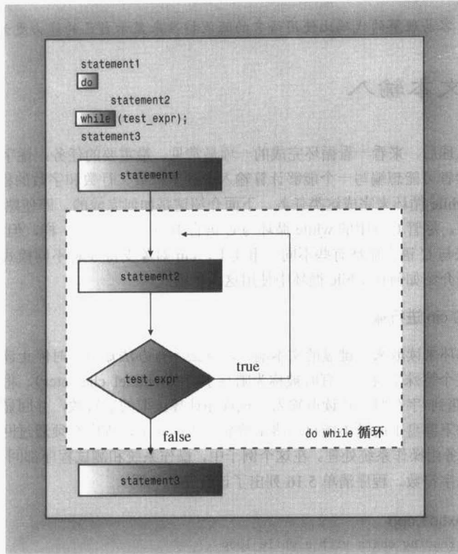
图 5.4 do while 循环的结构
