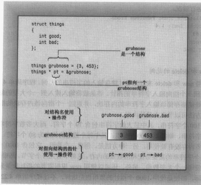
图 4.11 标识结构成员
