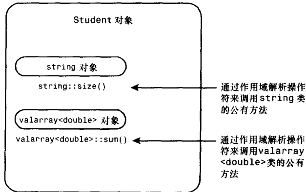
图 14.2 对象中的对象: 私有继承
