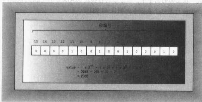
图 A.1 2 字节整数值
