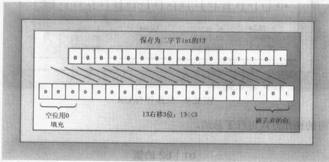
图 E.2 右移操作符
