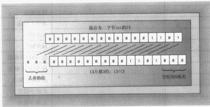
图 E.1 左移操作符
