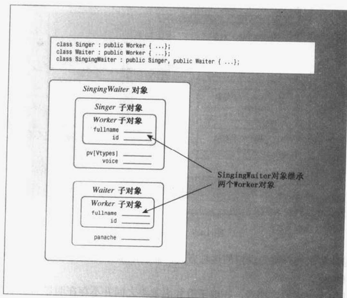
图 14.4 继承两个基类对象
