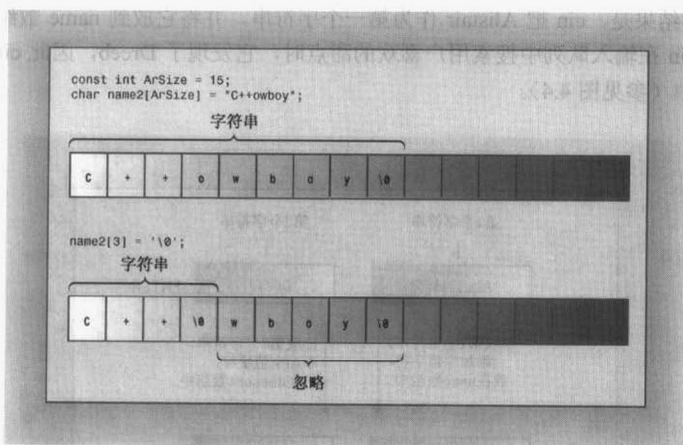
图 4.3 使用 \0 截短字符串
