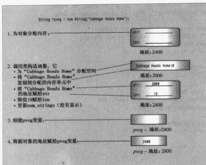
图 12.6 使用 new 创建对象
