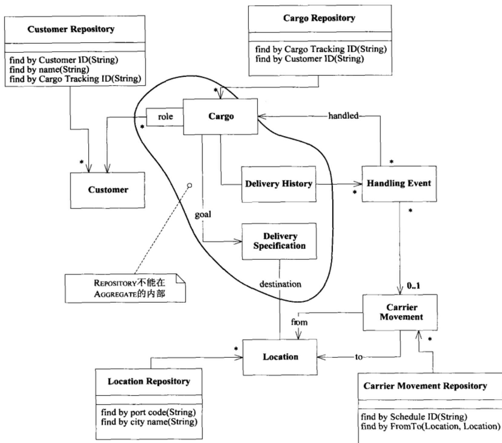
图7-4 REPOSITORY提供了对选中AGGREGATE根访问
