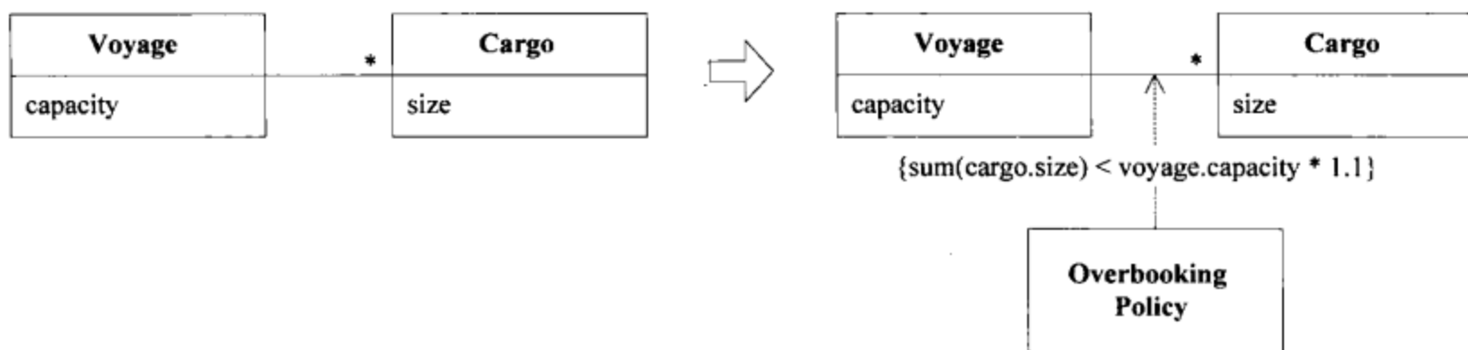
图9-11 为显式表达超订策略而重构的模型
