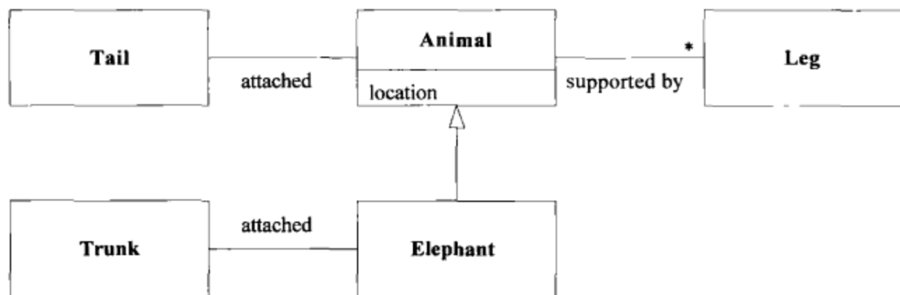
图14-12 一个更深入集成的上下文
