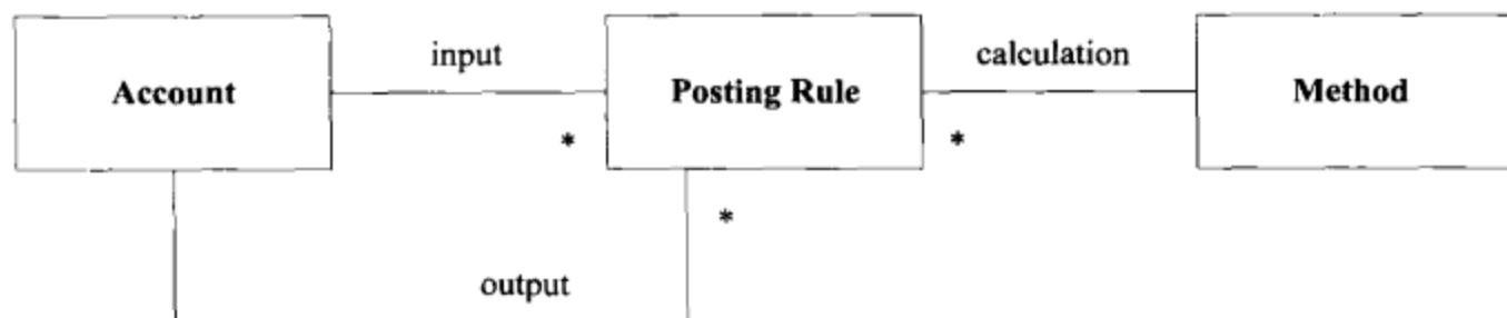
图11-8 基本过账规则的类型图
