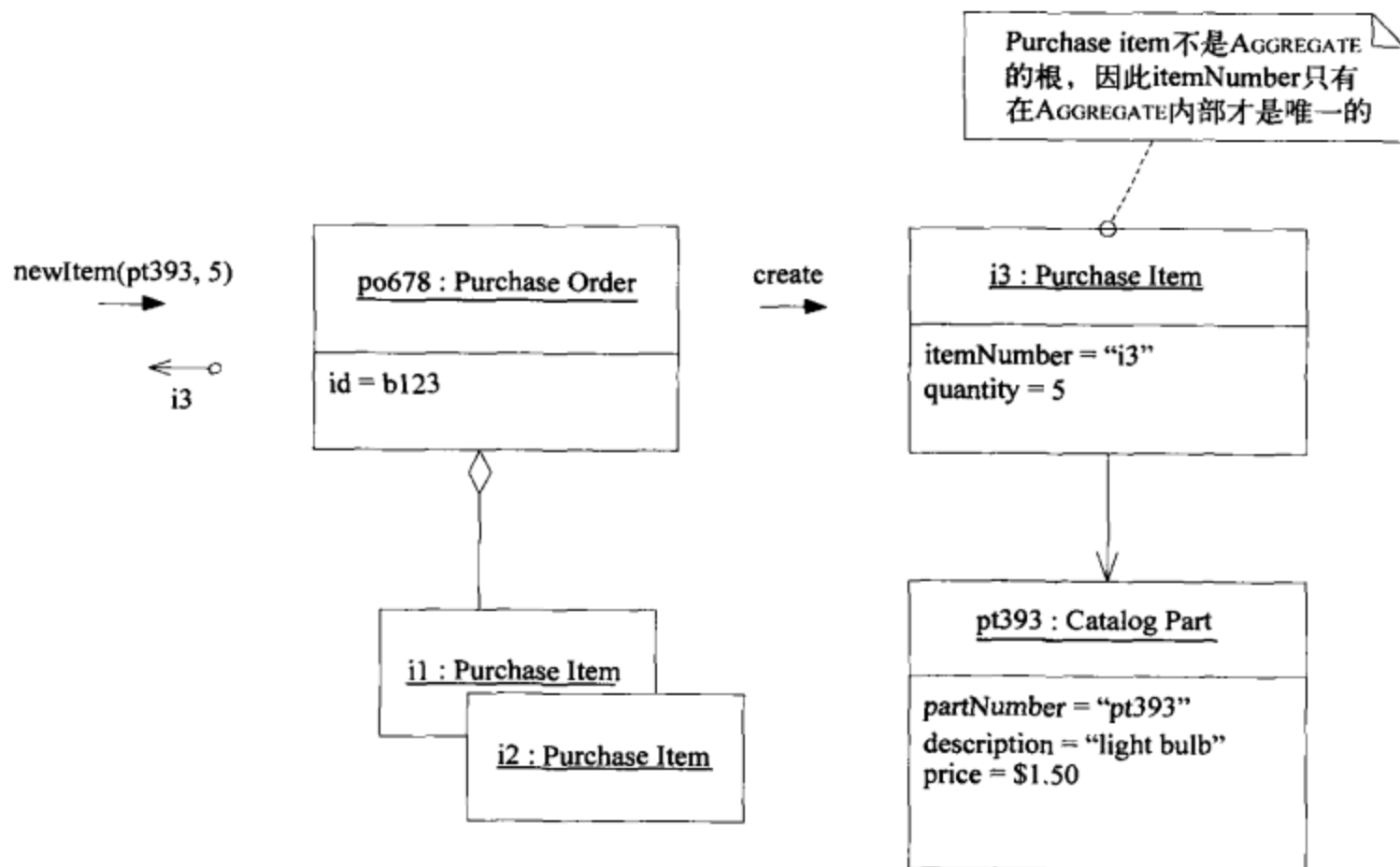
图6-13 一个FACTORY METHOD封装了AGGREGATE的扩展
