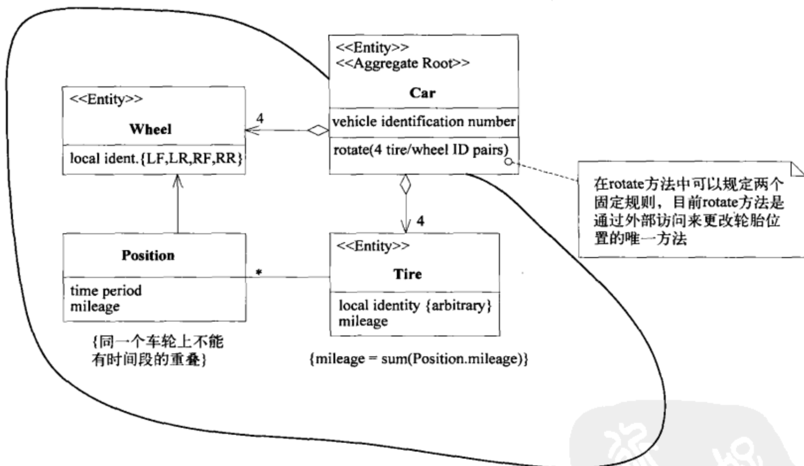
图6-3 AGGREGATE的固定规则
