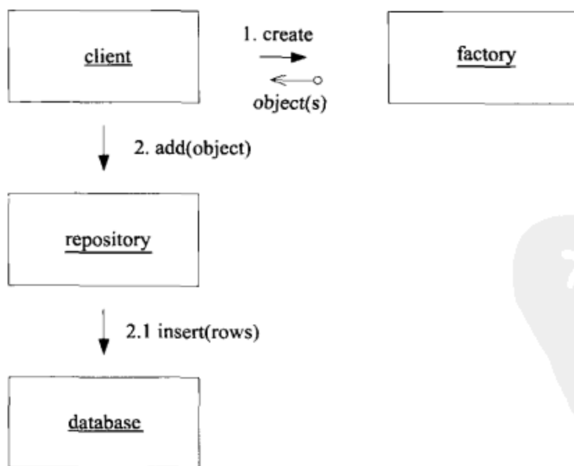
图6-23 客户使用REPOSITORY来存储新对象
