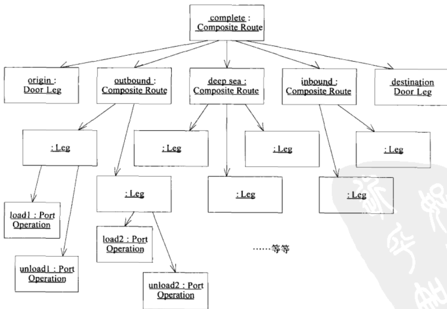
图12-9 表示了一个完整Route的实例
