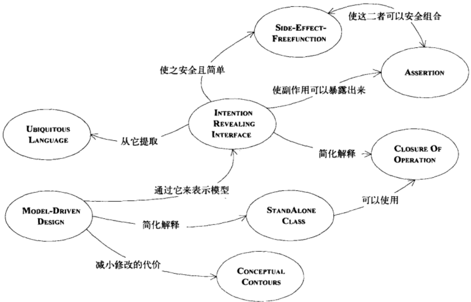
图10-1 一些有助于获得柔性设计的模式
