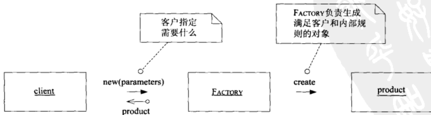
图6-12 与FACTORY的基本交互
