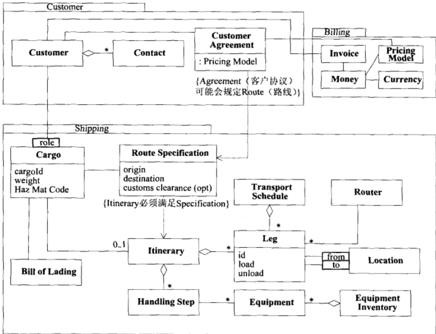
图7-8 基于广泛的领域概念的模块
