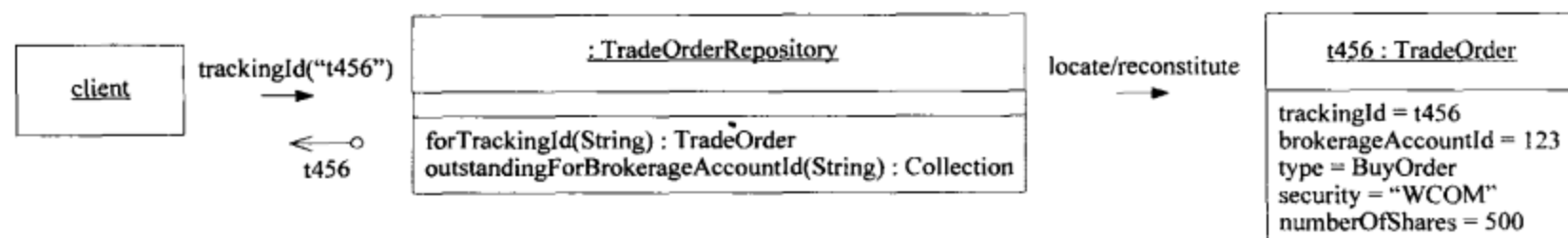
图6-19 在简单REPOSITORY中进行的硬编码查询
