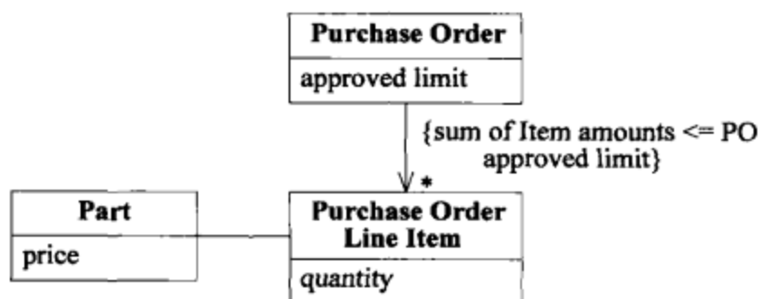
图6-4 一个采购订单系统的模型
