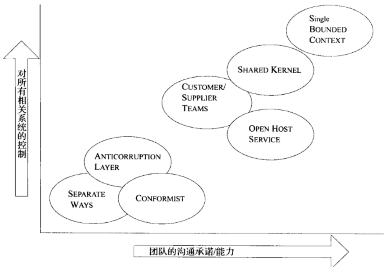
图14-13 CONTEXT关系模式的相对要求
