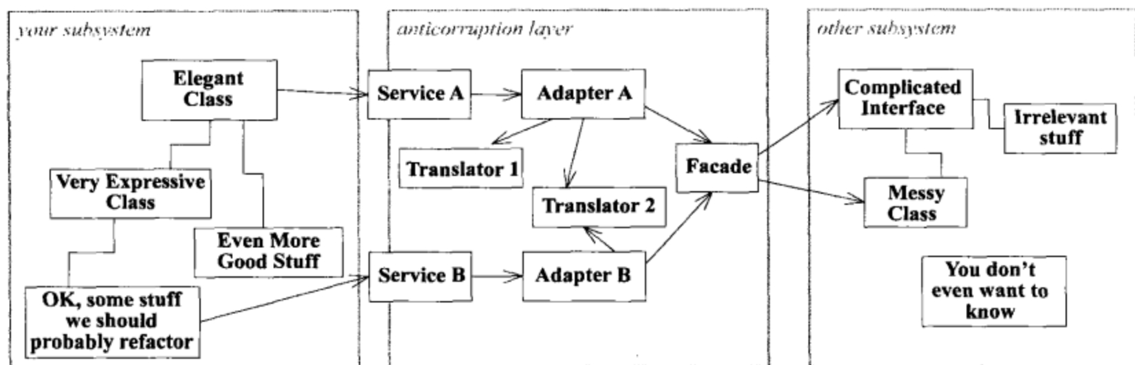
图14-8 ANTICORRUPTION LAYER的结构
