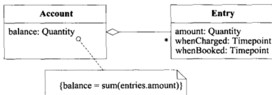
图11-2 一个基本的账户模型
