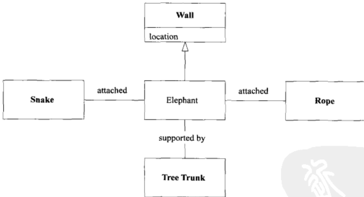
图14-11 一个粗略集成的上下文
