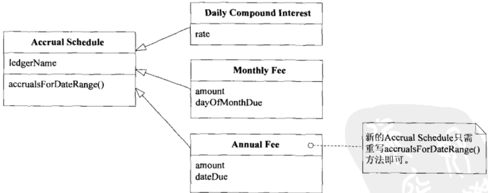
图10-12 这个模型把新的Accrual Schedule添加进来了
