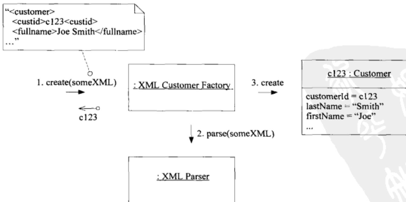
图6-17 重建以XML形式传输的ENTITY
