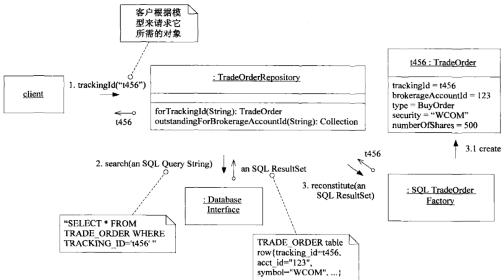
图6-21 REPOSITORY将底层数据存储封装起来
