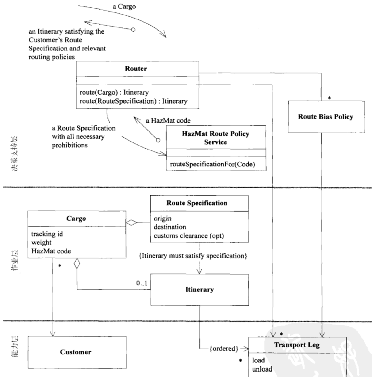
图 16-11 符合分层结构的一种设计
