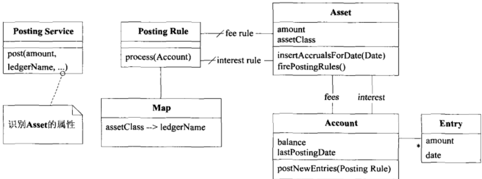
图11-10 含有过账规则的类型
