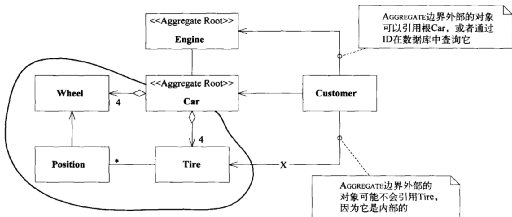
图6-2 本地标识与全局标识及对象引用
