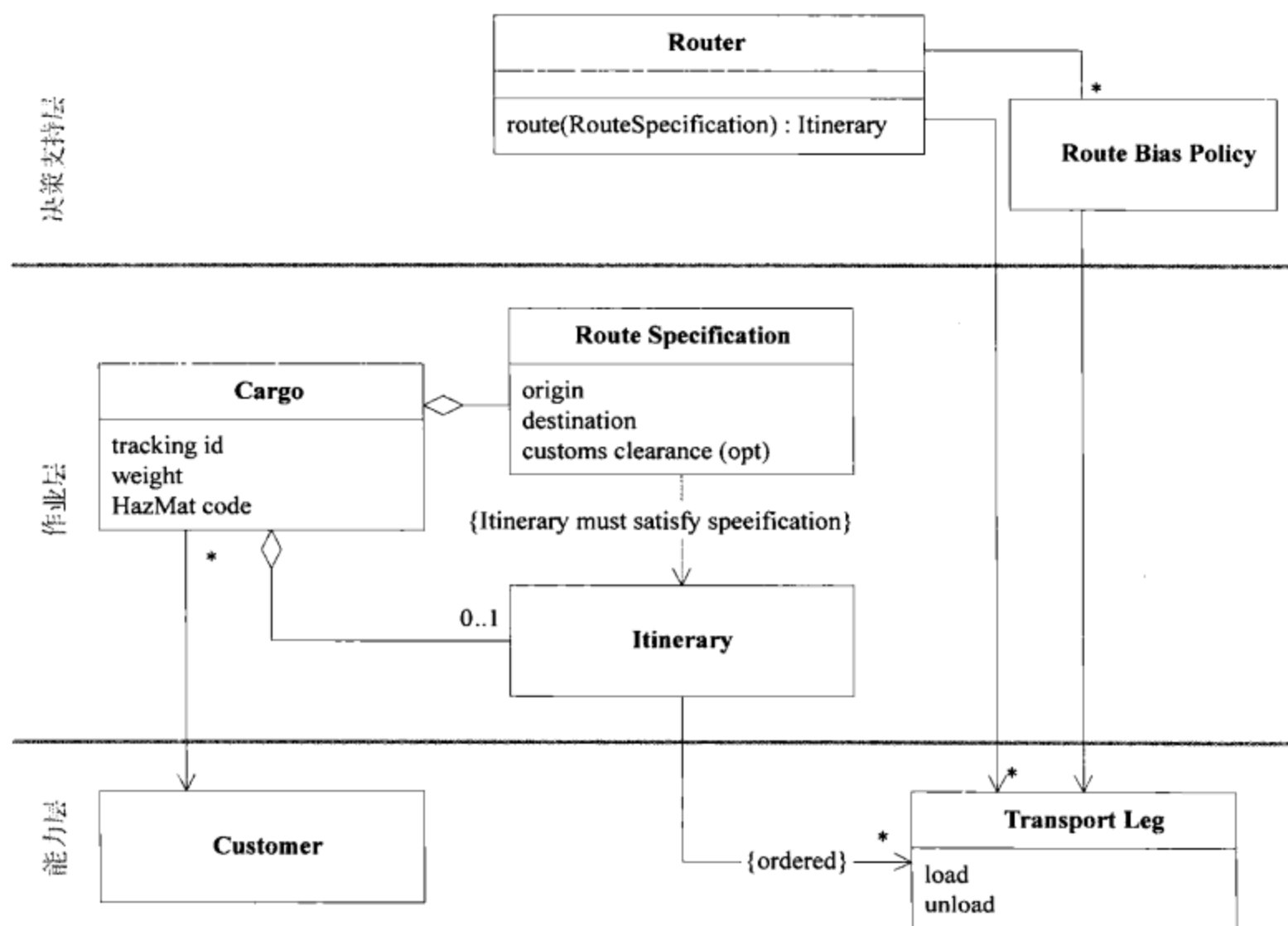
图 16-8 重构后的模型
