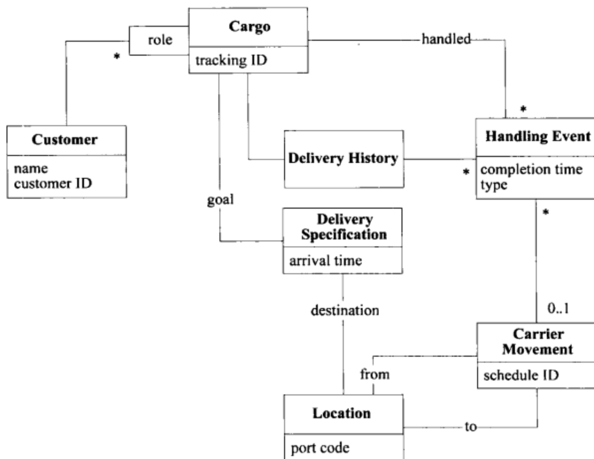
图7-1 表示货运领域模型的类图
