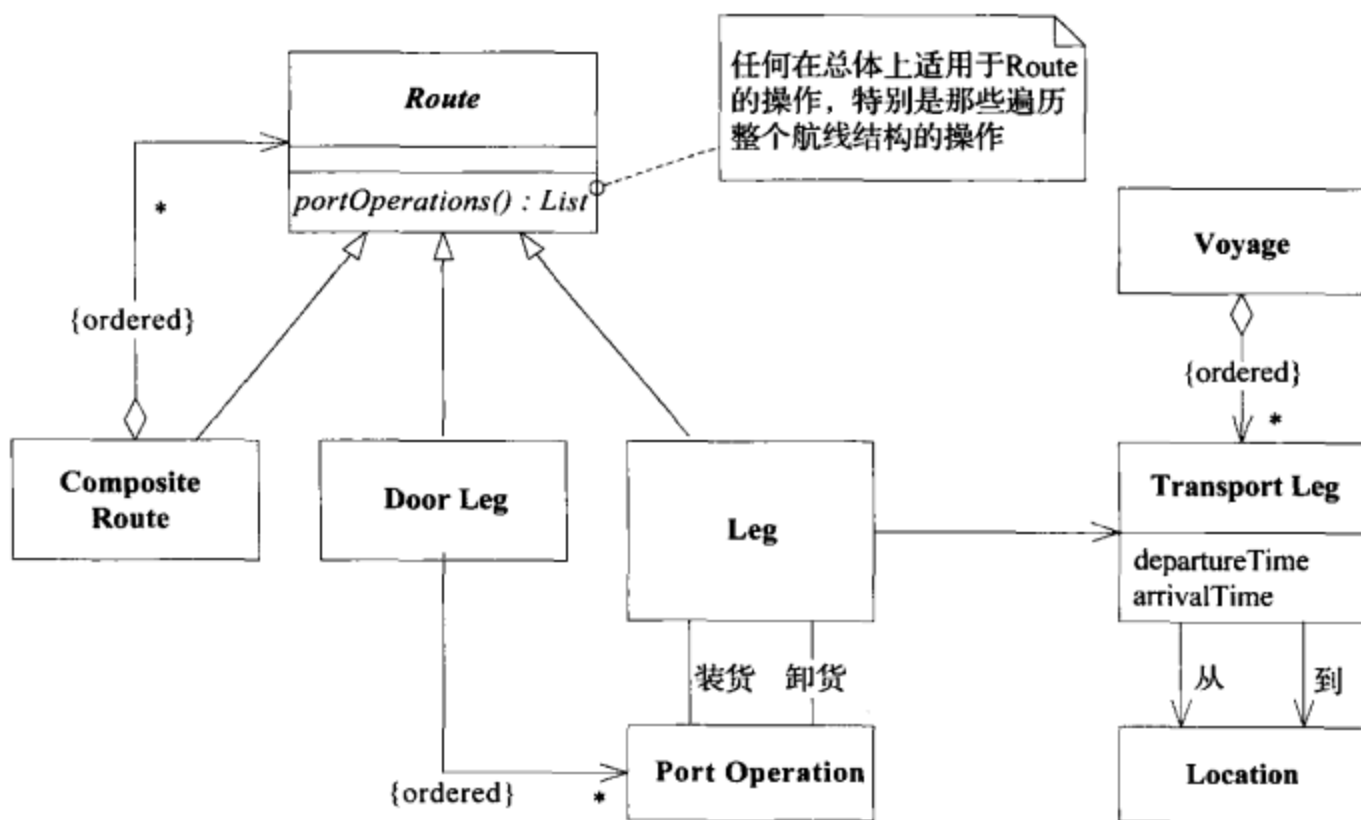
图12-8 使用COMPOSITE之后的类图
