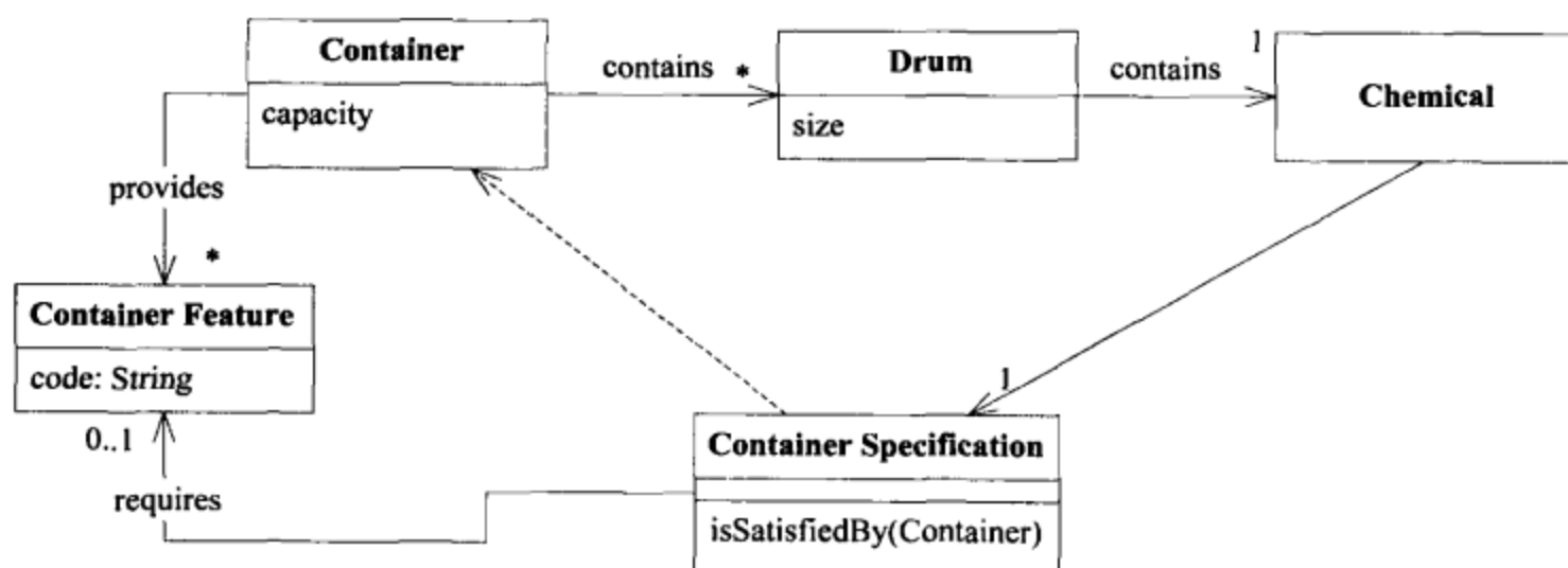
图9-16 仓库存储模型
