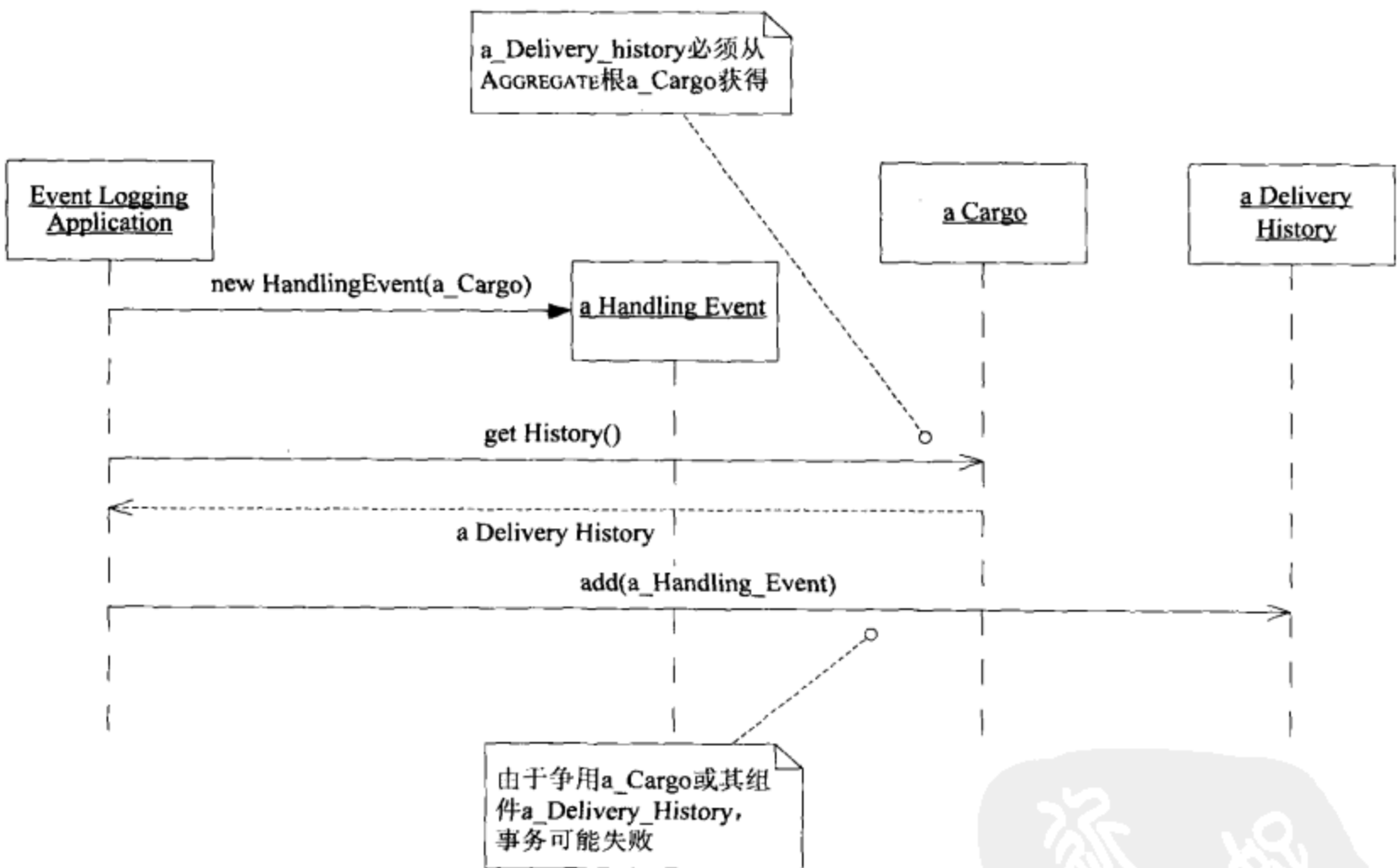
图7-5 添加一个Handling Event需要将它插入到Delivery History中
