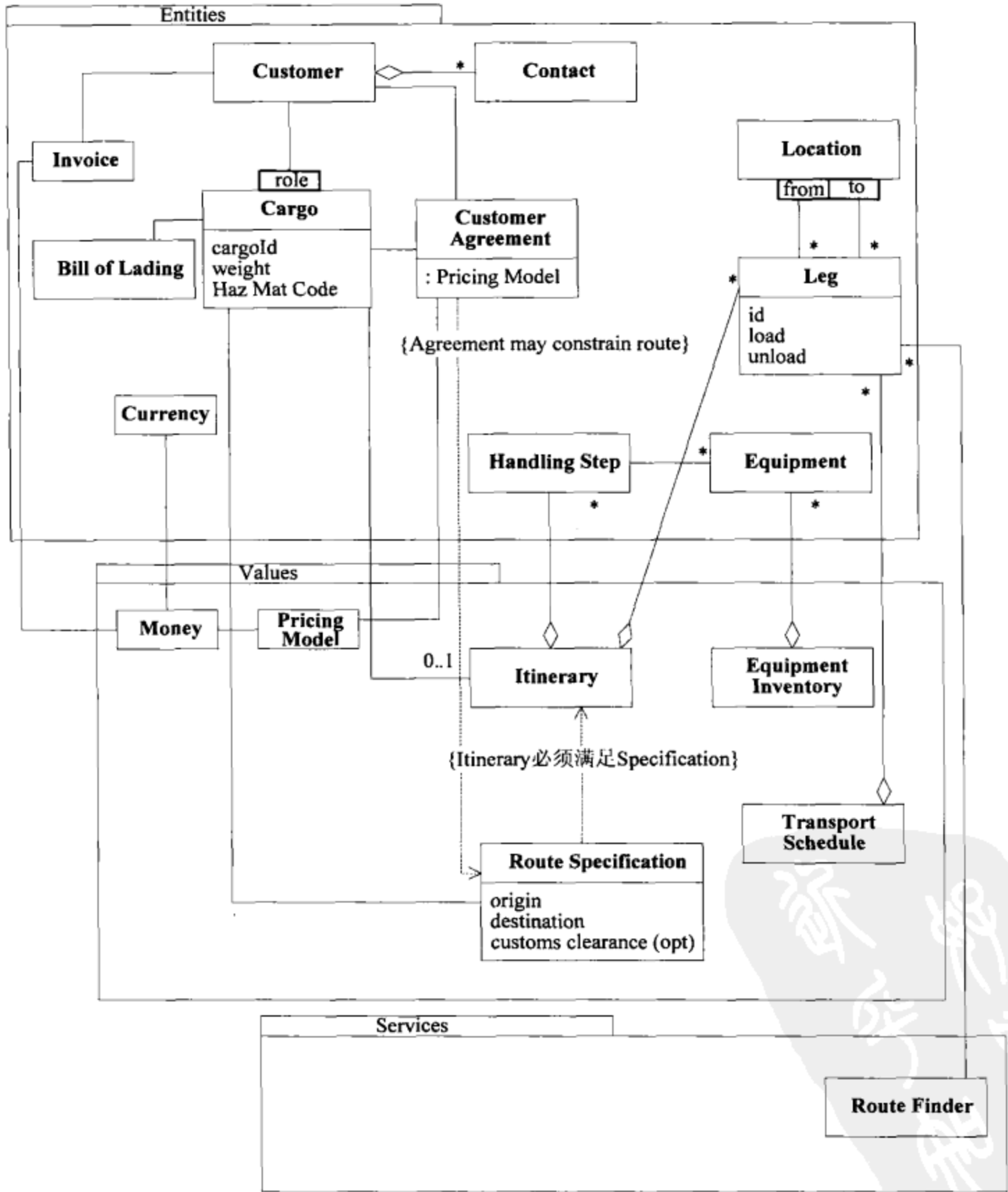
图7-7 这些MODULE并没有传达领域知识
