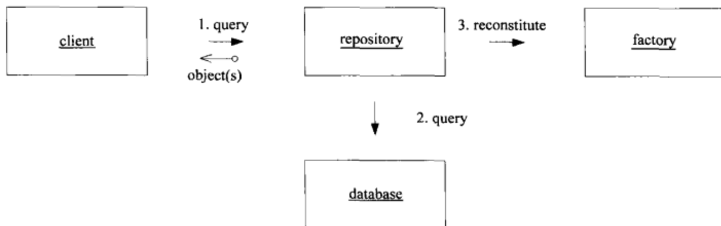
图6-22 REPOSITORY使用FACTORY来重建一个已有对象
