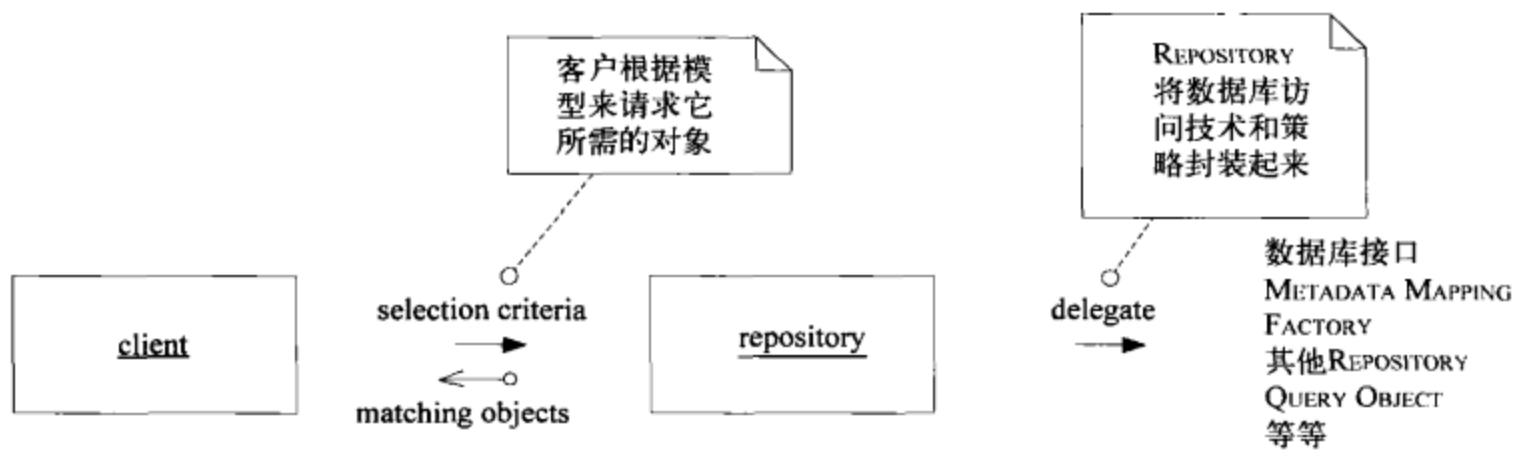
图6-18 REPOSITORY为客户执行一个搜索
