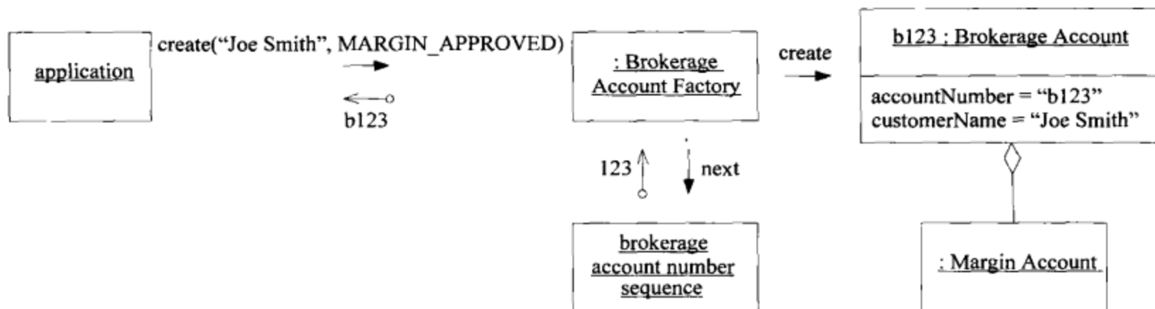
图6-15 由一个独立的FACTORY来构建AGGREGATE
