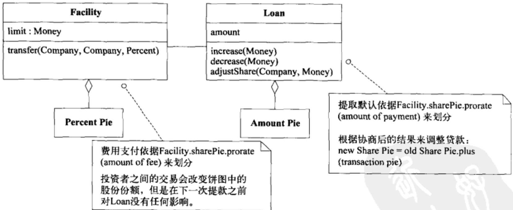
图8-8 使用Share Pie的Loan模型
