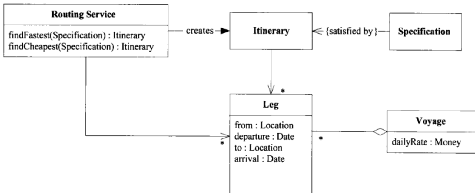
图12-1 带选项的SERVICE接口需要条件逻辑
