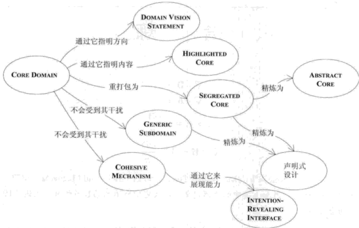
图15-1 战略精炼的导航图
