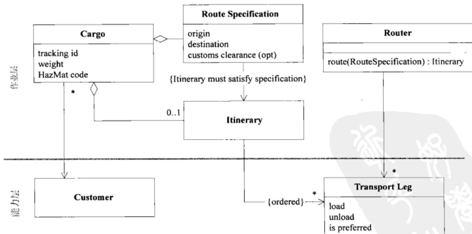
图 16-6 初次通过的分层模型
