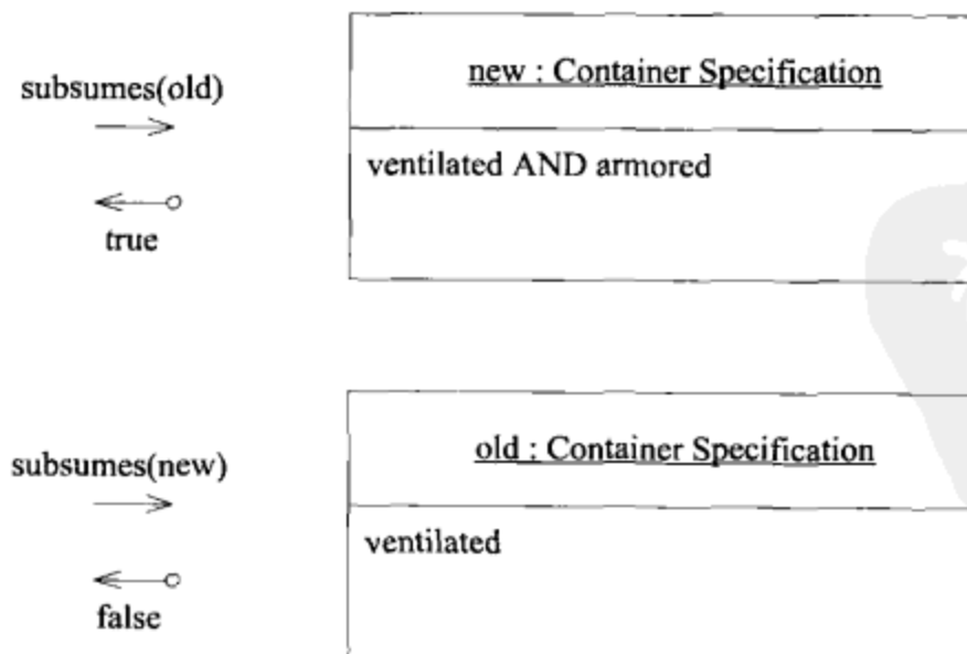
图10-15 汽油容器的SPECIFICATION变严格了
