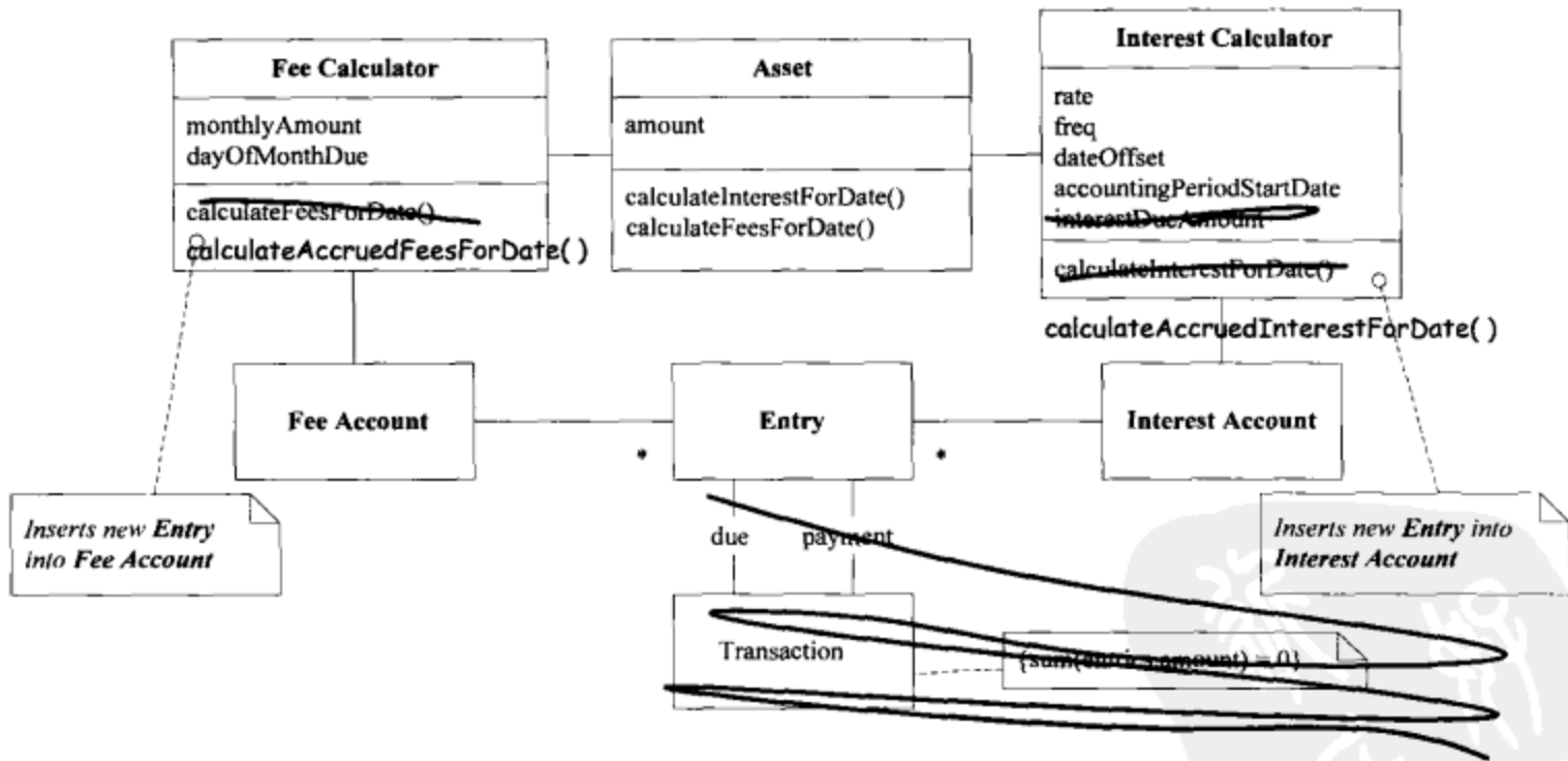
图11-6 基于账户的图, 里面没有Transaction
