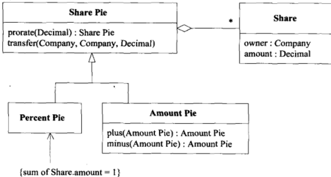
图8-7 股份的抽象模型
