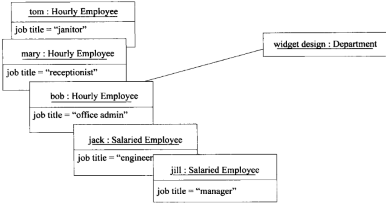
图 16-16 用原来的模型表示出来的一些员工
