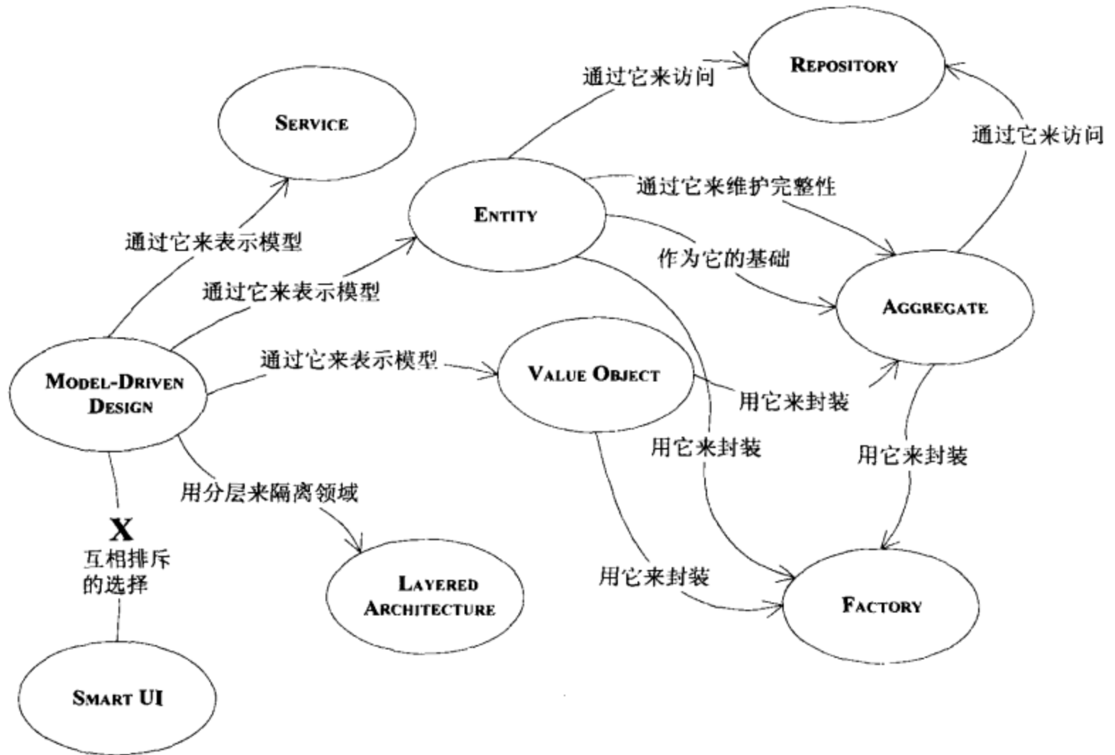
MODEL-DRIVEN DESIGN语言的导航图
