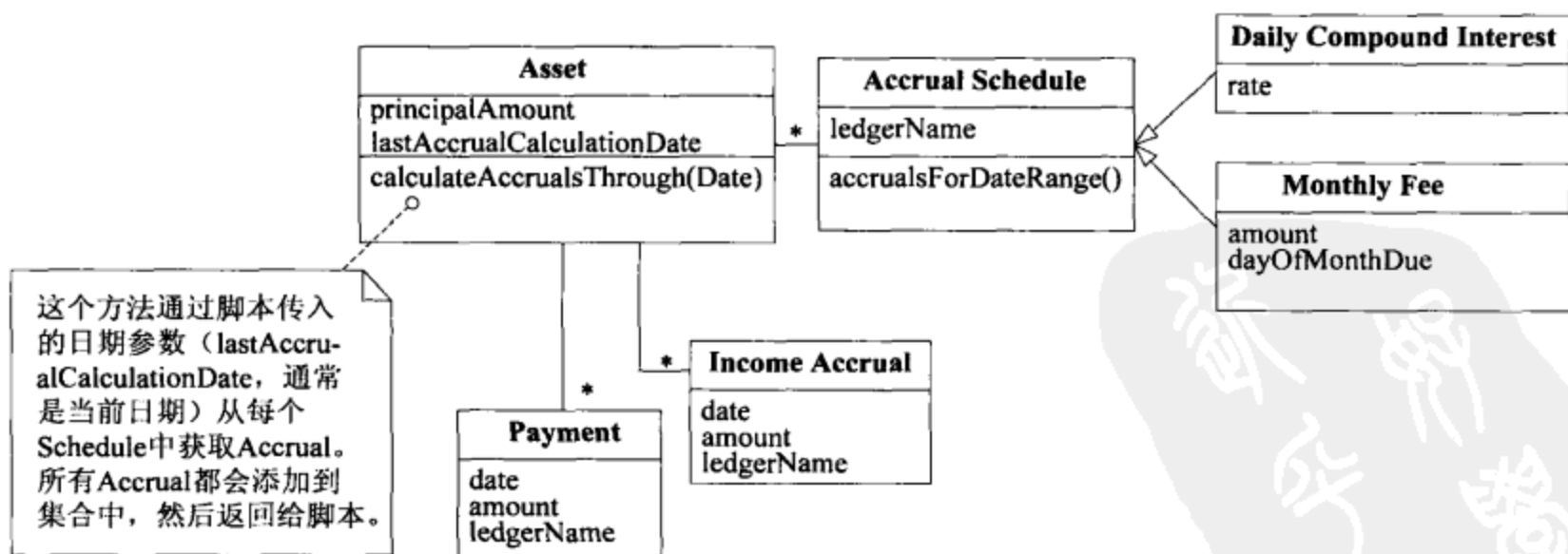
图9-8 重构后的深层模型
