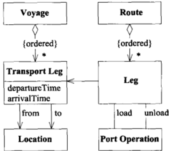
图2-4 航运路线的类图
