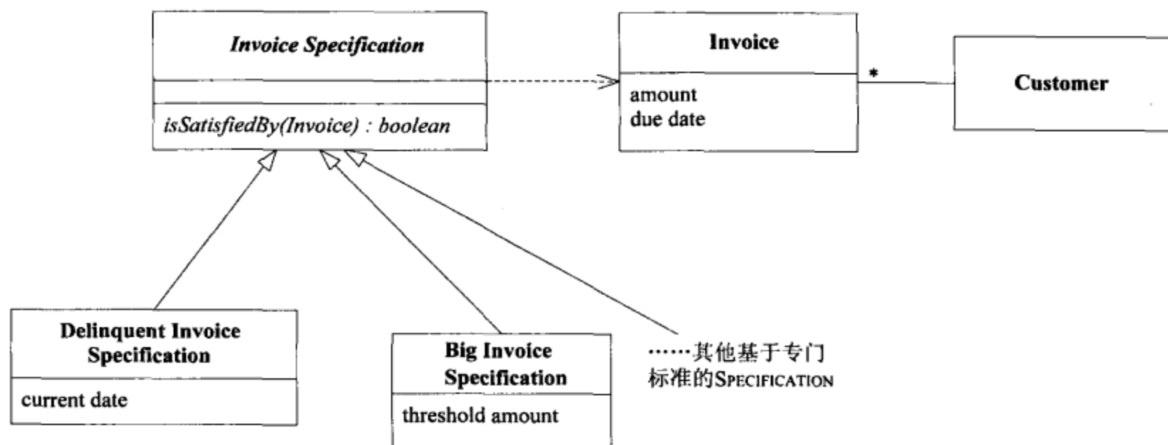
图9-14 应用 SPECIFICATION 进行验证的模型
