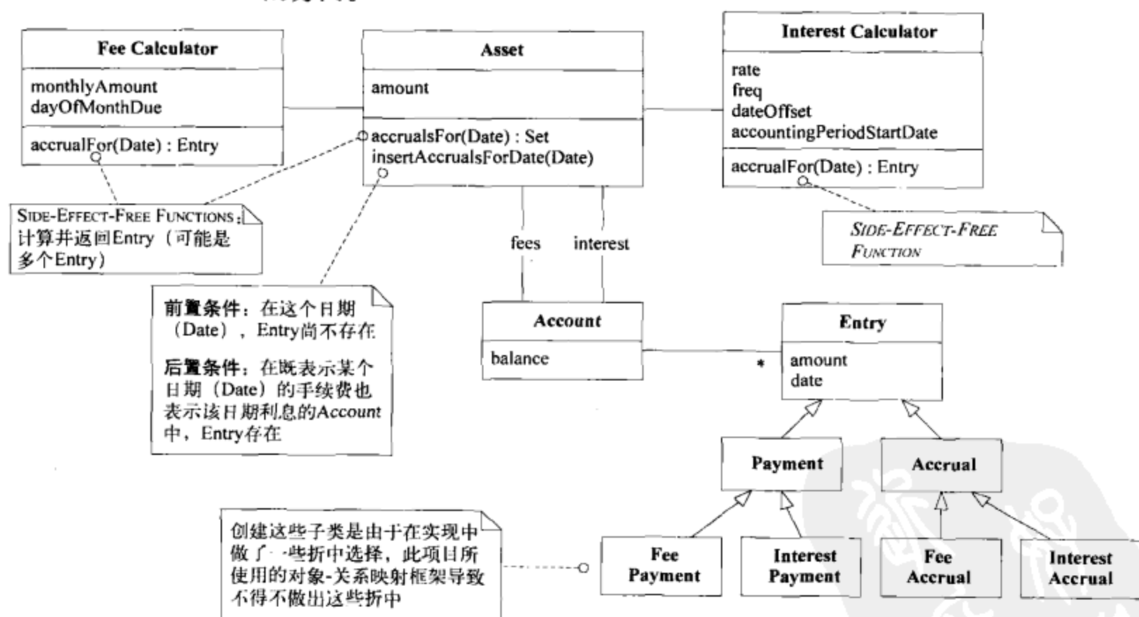
图11-7 实现之后的类图
