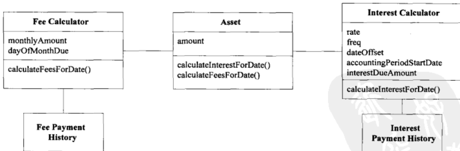
图9-4 笨拙的模型
