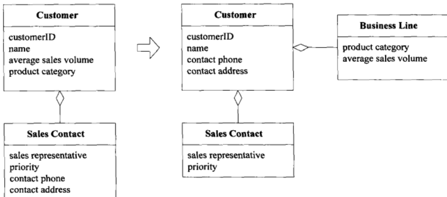
图5-5 与标识有关的属性留在ENTITY内
