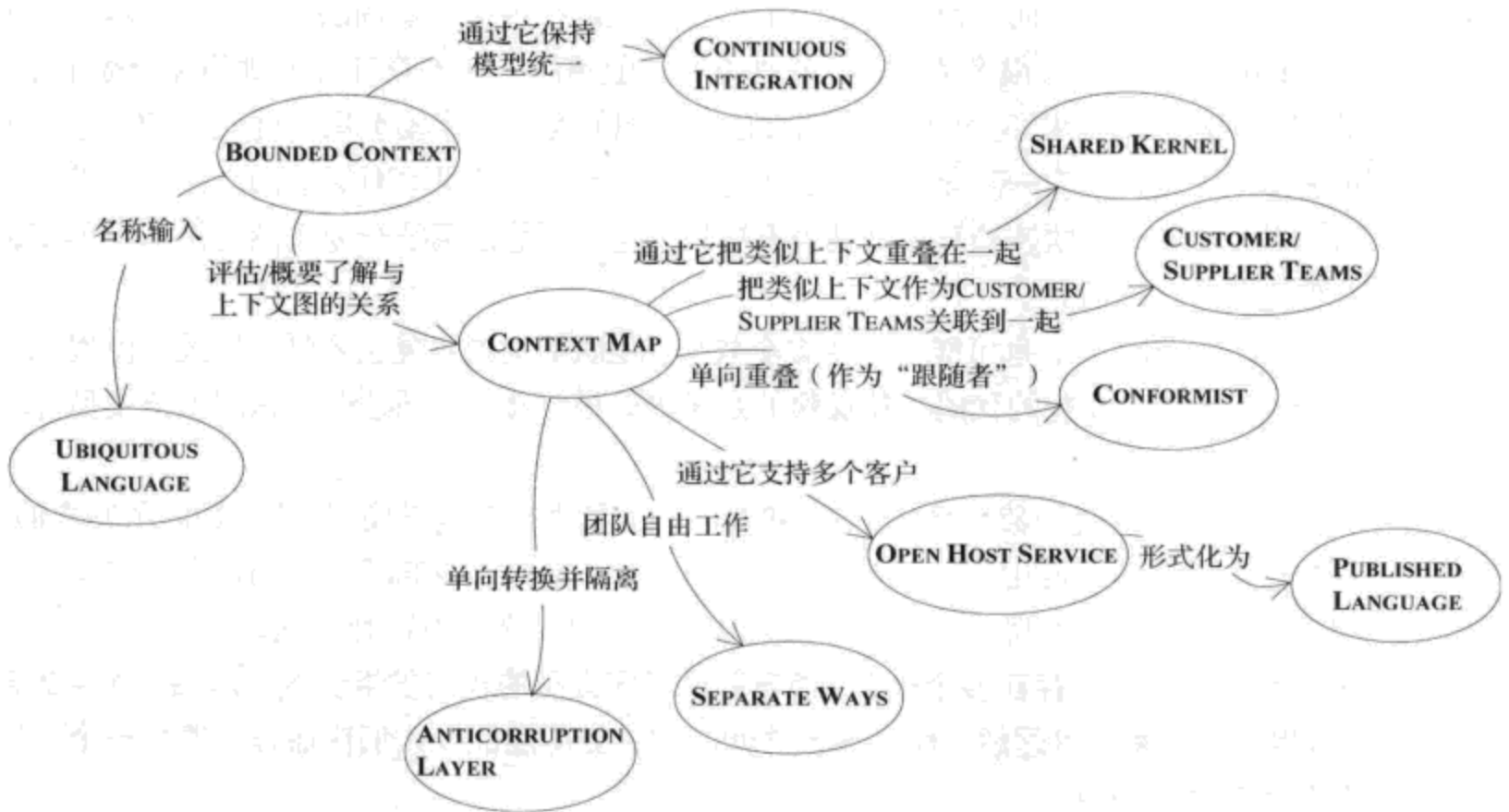
图14-1 模型完整性模式的导航图
