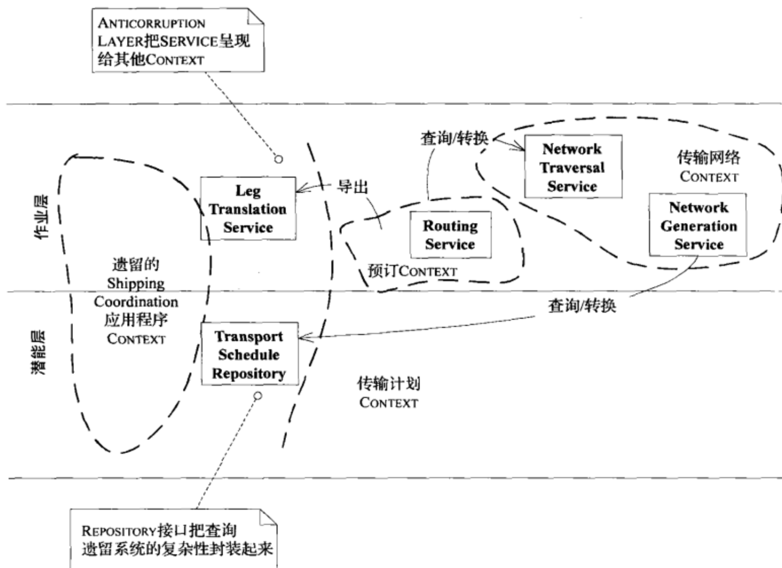
图17-4 允许一些组件跨越多个层的结构
