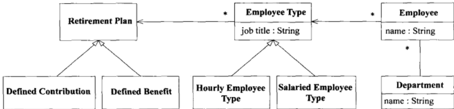
图 16-19 Type 对象能够满足需求
