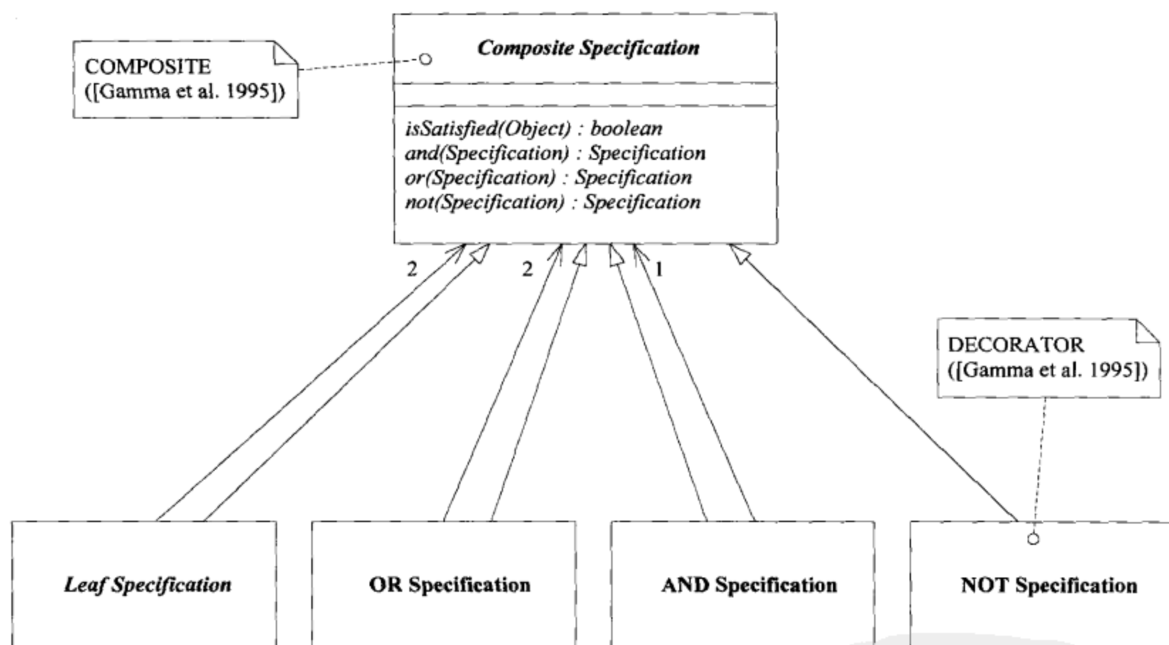
图10-14 SPECIFICATION的COMPOSITE（组合）设计
