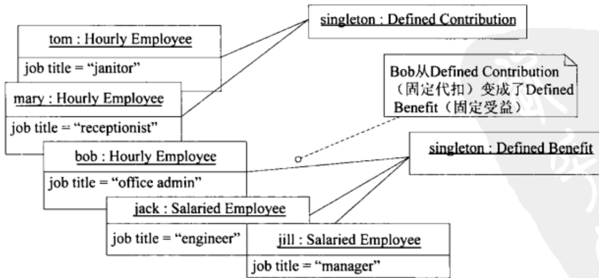
图 16-18 员工可能会与错误的计划关联起来
