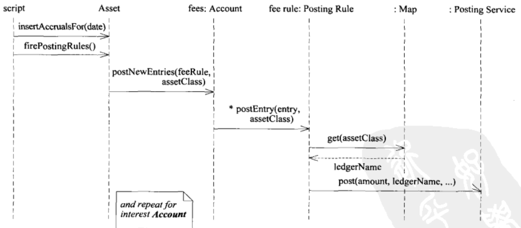
图11-11 显示了规则触发的序列图
