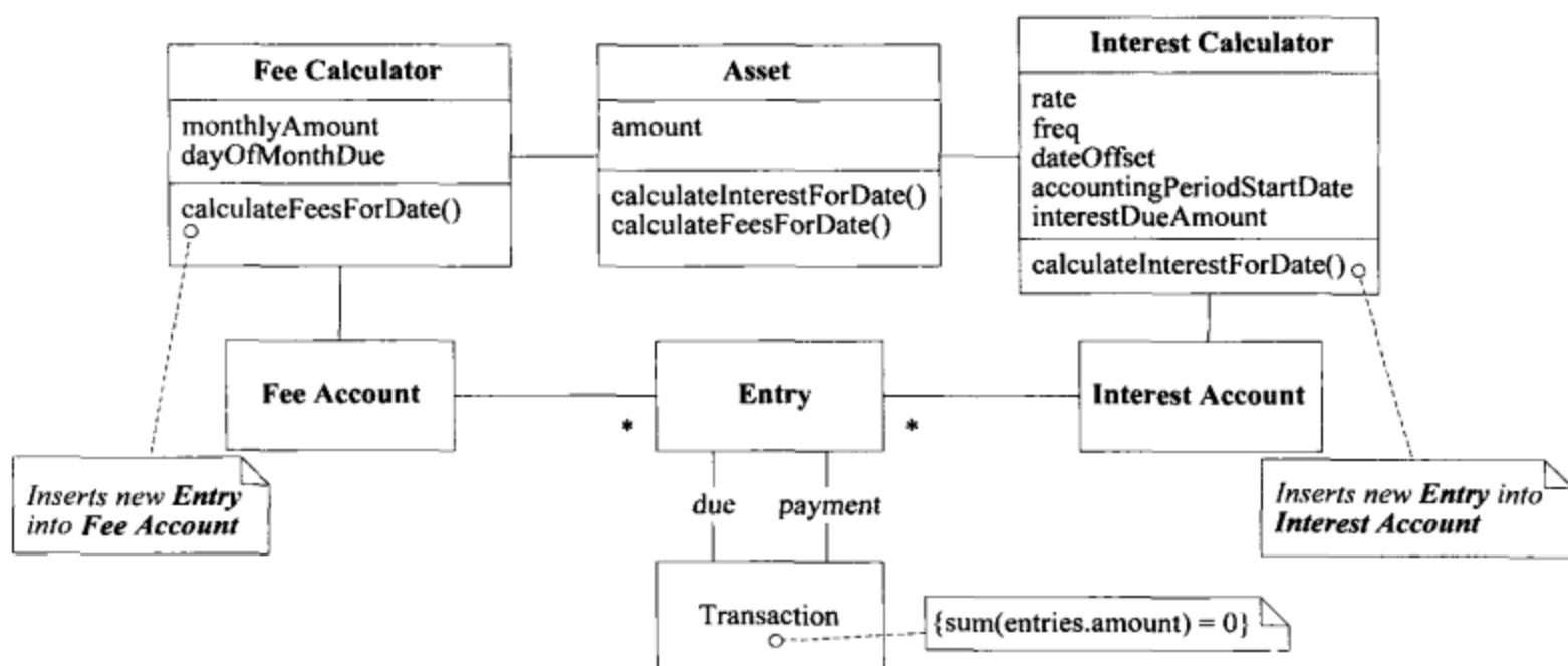
图11-4 新提出的模型
