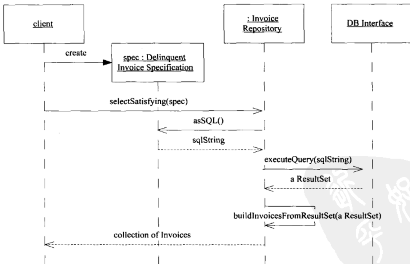
图9-15 REPOSITORY和SPECIFICATION之间的交互
