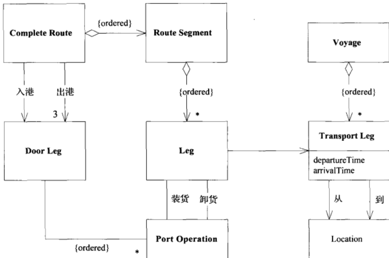
图12-7 详细的Route类图
