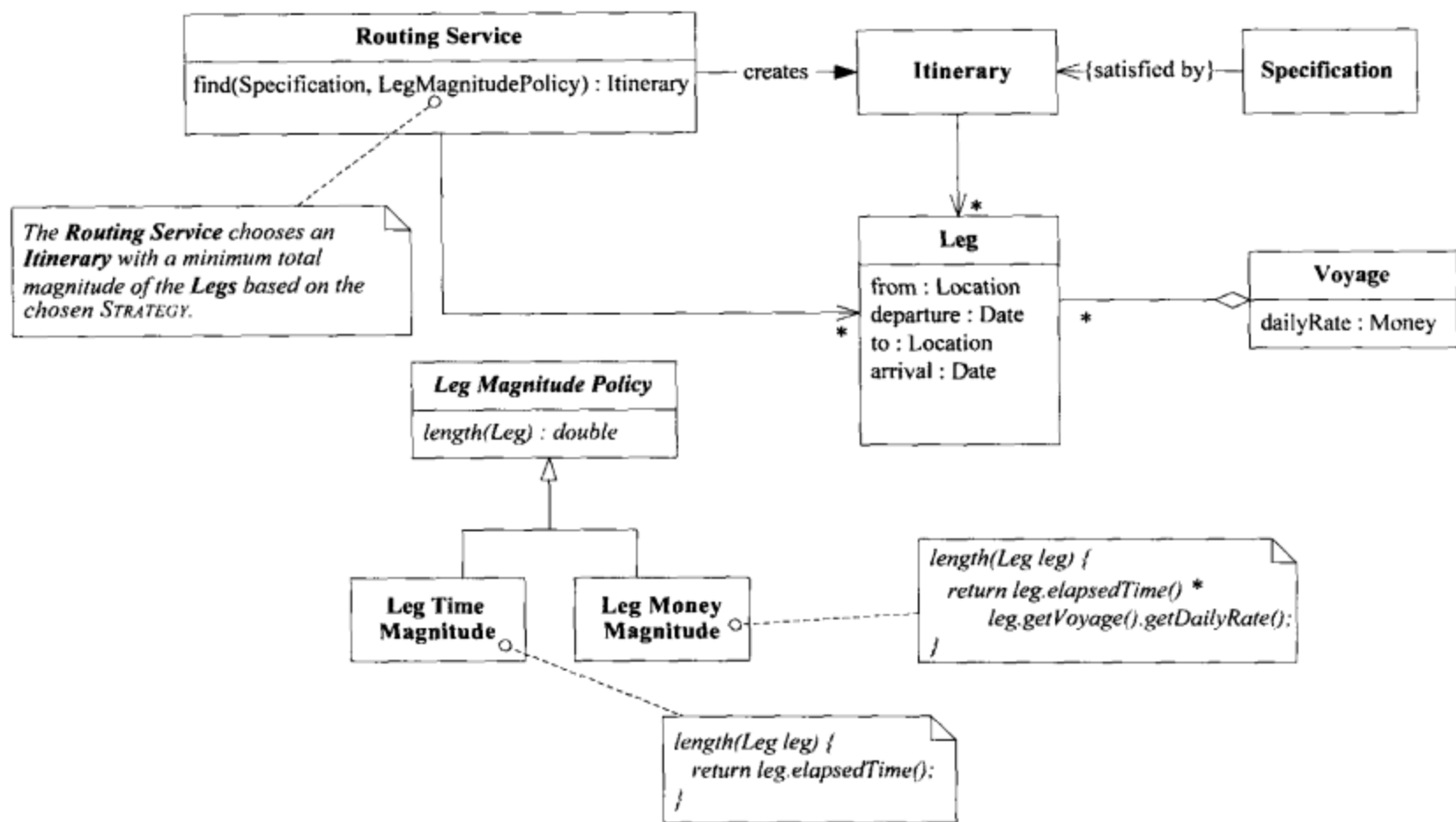
图12-2 通过STRATEGY (或者POLICY) 选择确定的选项 (STRATEGY是作为参数传入的)
