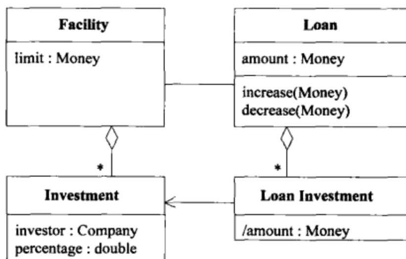
图8-1 假定放贷方所持股份固定的模型
