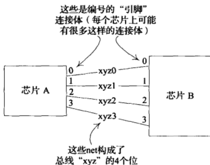
图3-2 net构成总线的示意图
