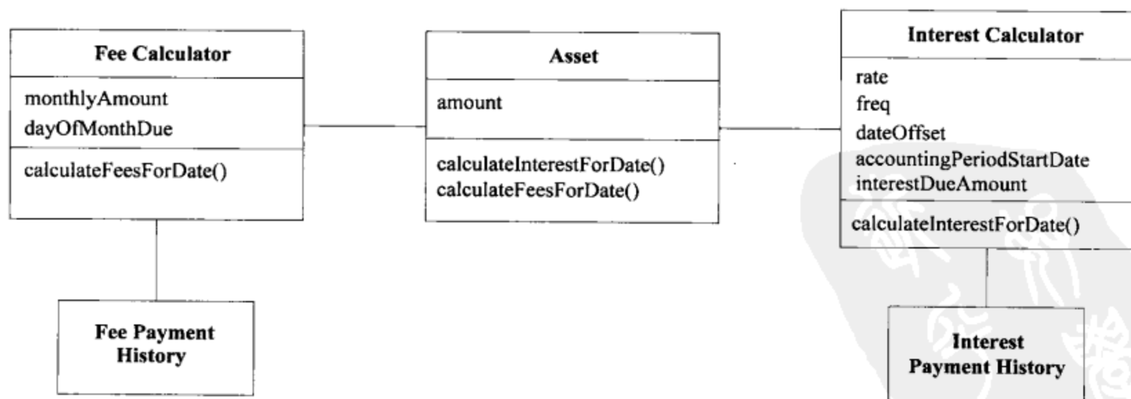
图11-1 初始的类图
