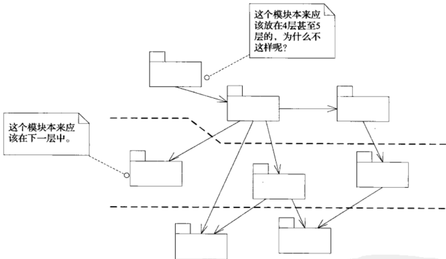
图 16-2 特定分层, 这些包描述了什么事情
