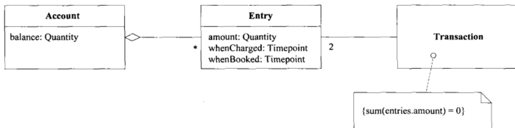
图11-3 一个交易模型
