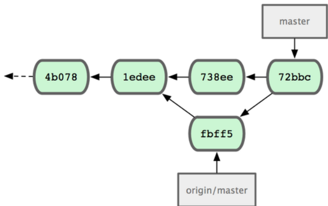
图 5.5: 合并 origin/master 后 John 的仓库历史
