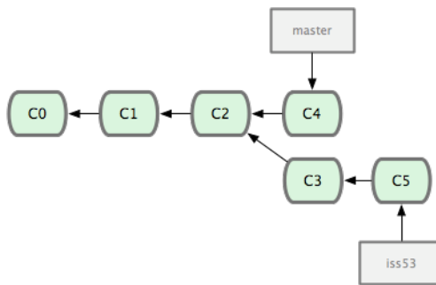
图 3.15: iss53 分支可以不受影响继续推进。
