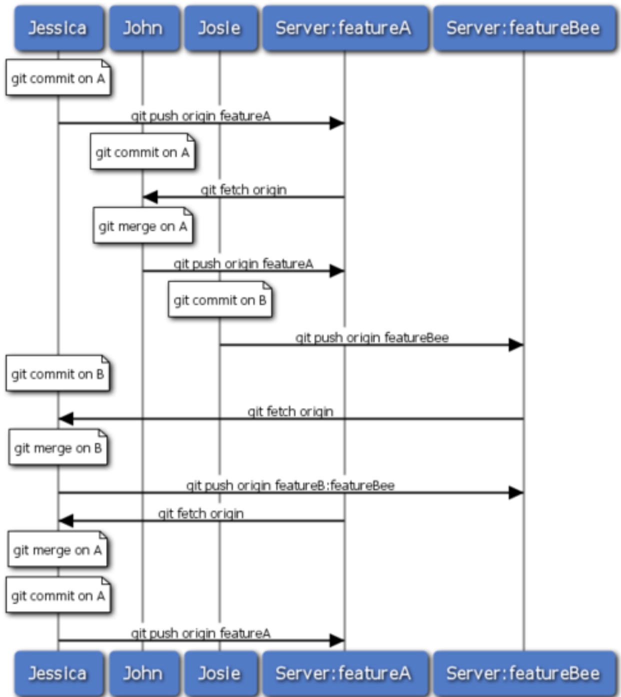
图 5.15: 团队间协作工作流程基本时序
