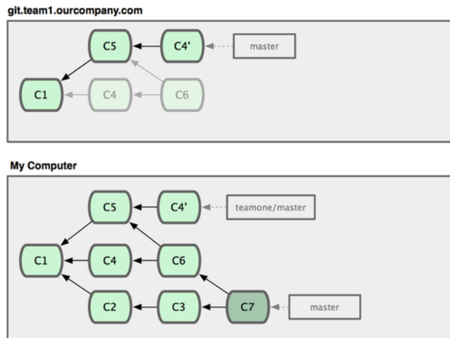
图 3.38: 有人推送了符合过的 C4'，丢弃了你作为开发基础的 C6。
