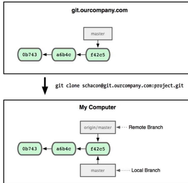
图 3.22: 一次 Git 克隆会建立你自己的本地分支 master 和远程分支 origin/master ，它们都指向
