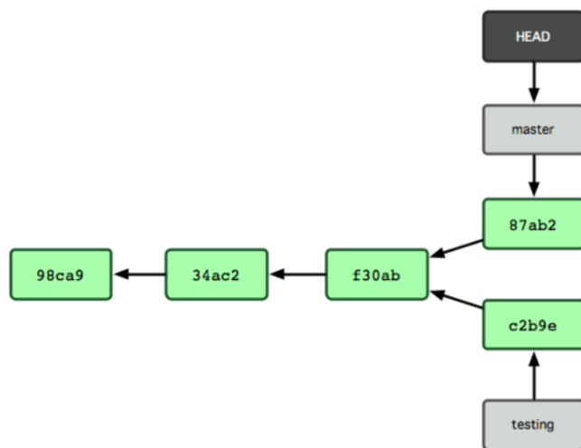
图 3.9：分叉了的分支历史
