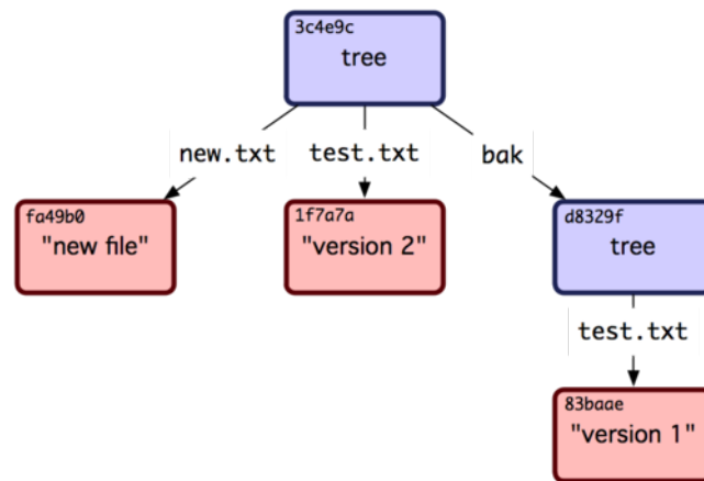
图 9.2: 当前 Git 数据的内容结构
