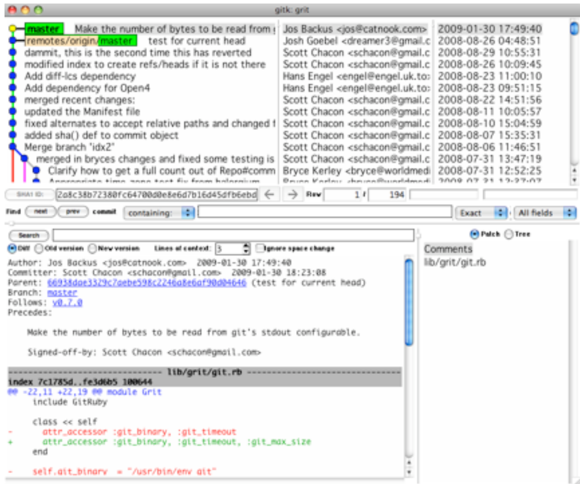
图 2.2: gitk 的图形界面
