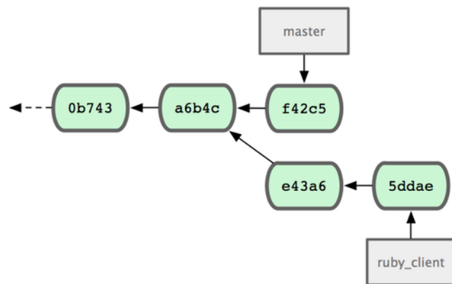
图 5.26: 挑拣 (cherry-pick) 之前的历史
