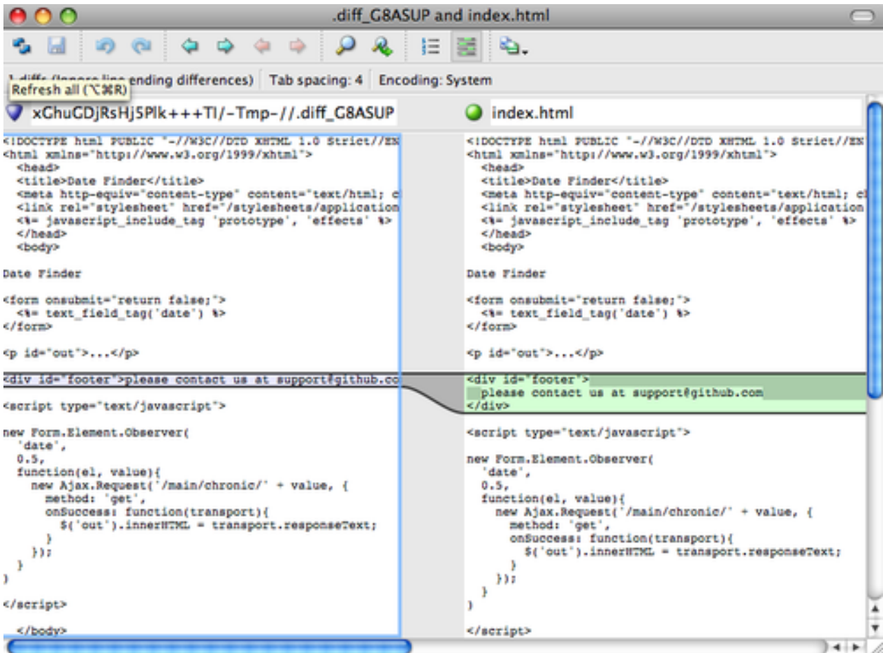
图 7.1: P4Merge。
