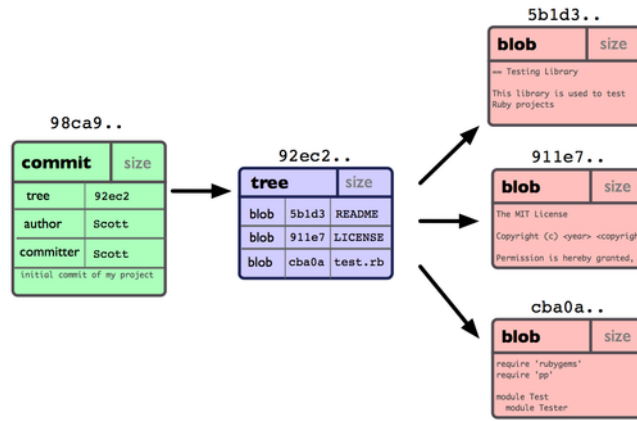
图 3.1: 一次提交后仓库里的数据
