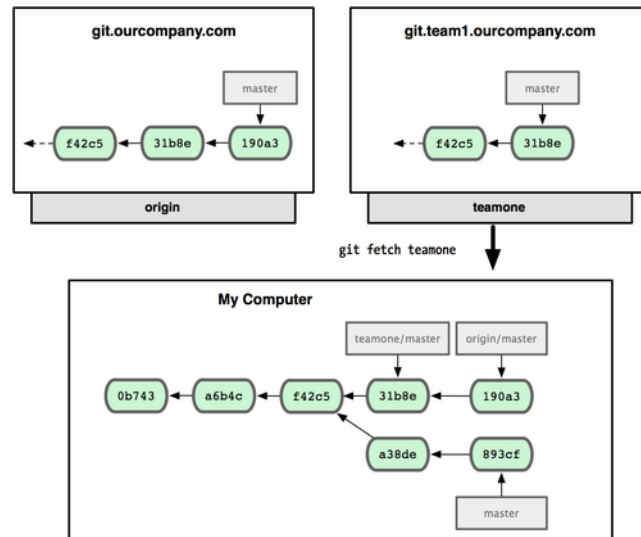
图 3.26: 你在本地有了一个指向 teamone 服务器上 master 分支的索引。
