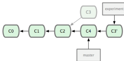
图 3.29: 把 C3 里产生的改变行合到 C4 中。
