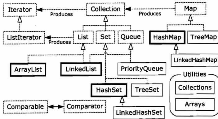
简单的容器分类
