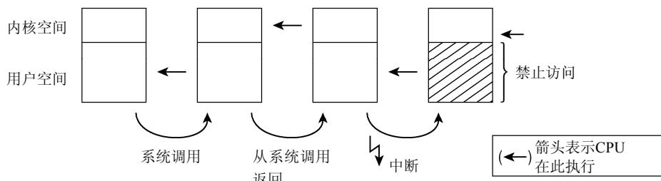
图1-5 在核心态和用户状态执行。CPU大多数时间都在执行用户空间中的代码。当应用程序执行系统调用时，则切换到核心态，内核将完成其请求。在此期间，内核可以访问虚拟地址空间的用户部分。在系统调用完成之后，CPU切换回用户状态。硬件中断也会使CPU切换到核心态，这种情况下内核不能访问用户空间
