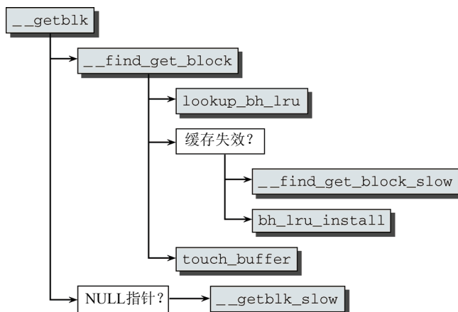
图16-9 __getblk的代码流程图
