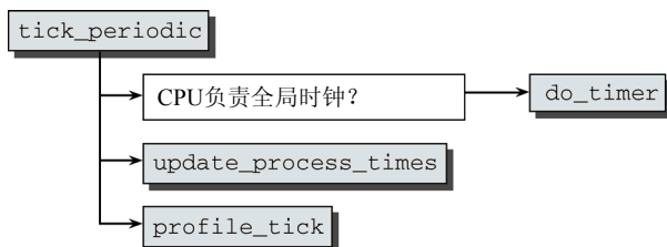
图15-11 tick_periodic的代码流程图
