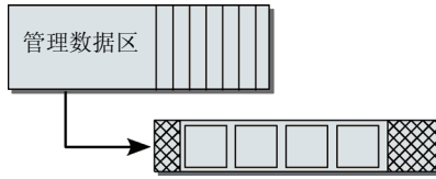
图3-48 slab首部位于slab外部的情况
