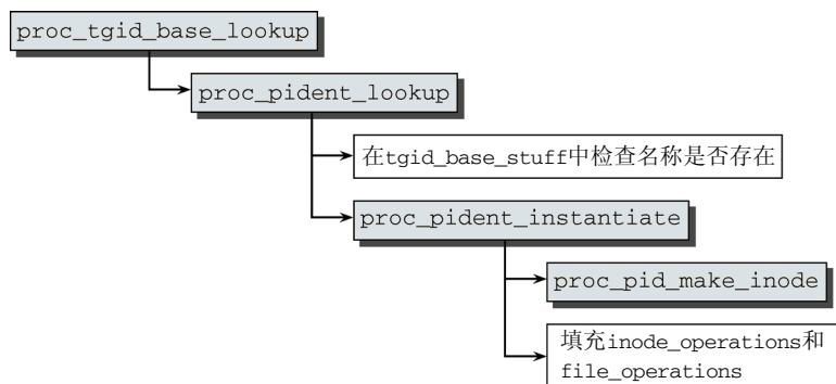
图10-5 proc_tgid_base_lookup 的代码流程图
