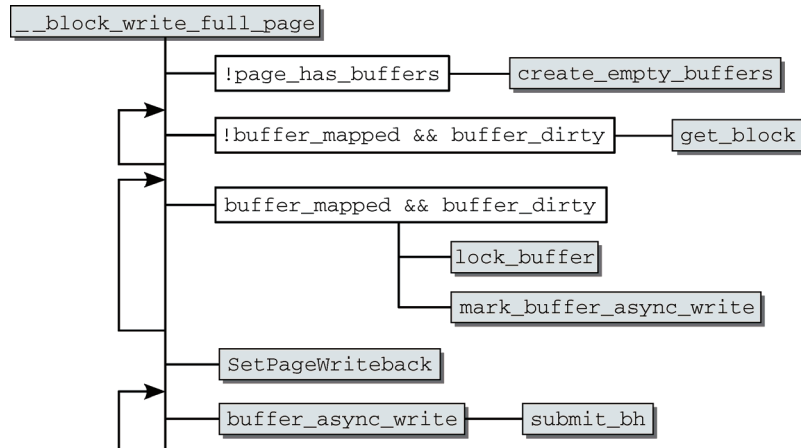
图16-8 __block_write_full_page的缓冲区相关操作的代码流程图
