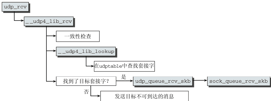
图12-23 udp_rcv的代码流程图
