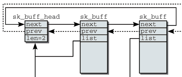
图12-8 通过双链表管理套接字缓冲区
