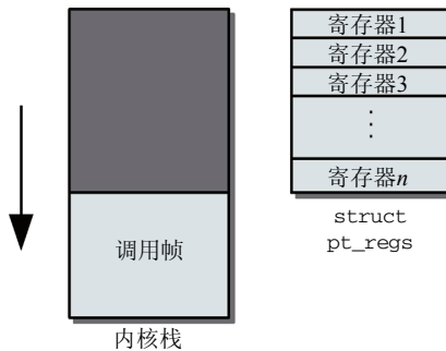
图14-8 进入核心态之后栈的布局
