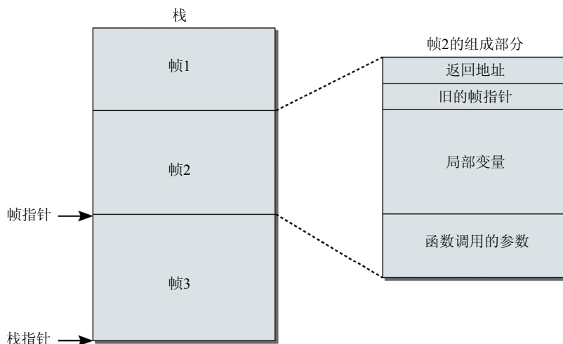
图C-1 栈上的各个活动记录
