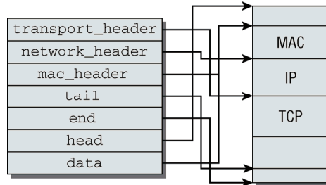
图12-6 套接字缓冲区和网络分组数据之间的关联
