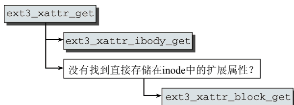
图11-5 ext3_xattr_get的代码流程图
