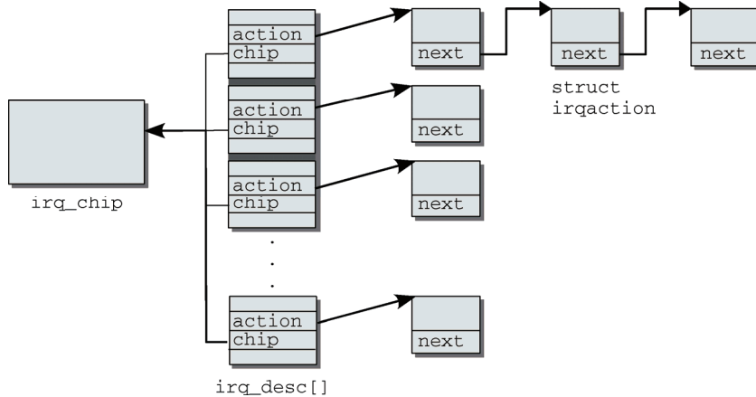
图14-4 IRQ管理涉及的各数据结构
