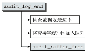
图19-6 audit_log_end 的代码流程图
