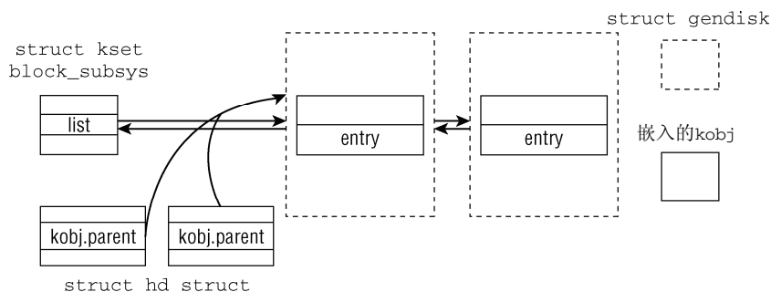
图6-11 通用硬盘gendisk与一般的内核对象框架的集成
