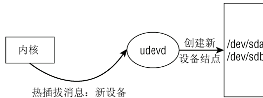
图6-3 使用udev从用户层管理设备结点
