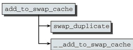
图18-9 add_to_swap_cache 的代码流程图
