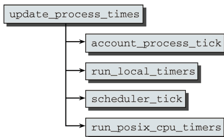
图15-23 update_process_times的代码流程图
