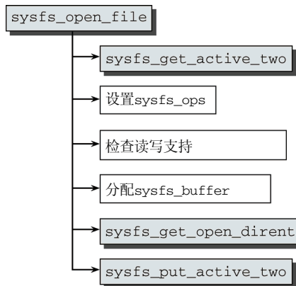
图10-13 sysfs_open_file 的代码流程图
