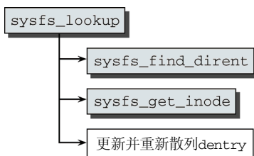
图10-16 sysfs_lookup 的代码流程图
