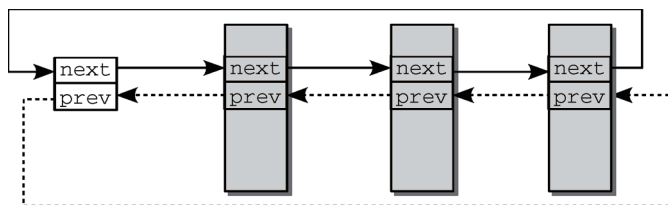
图1-11 标准双链表
