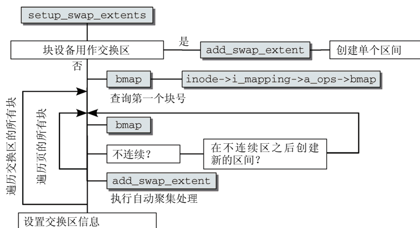
图18-3 setup_swap_extents的代码流程图
