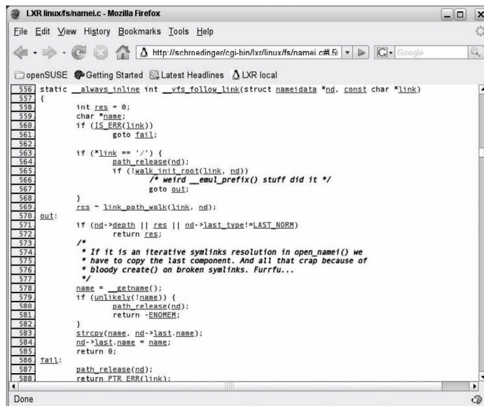
图B-4 通过LXR生成的超本来查看Linux源代码
