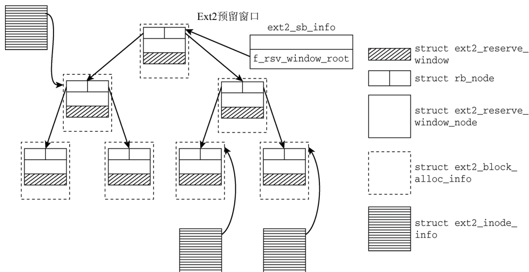
图9-7 预分配机制使用的数据结构
