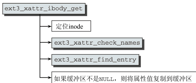
图11-6 ext3_xattr_ibody_get的代码流程图
