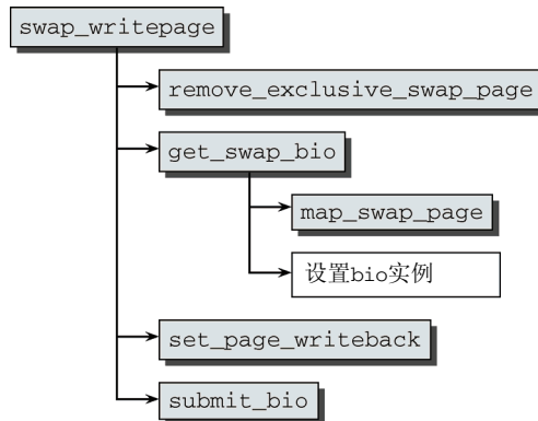
图18-10 swap_writepage的代码流程图
