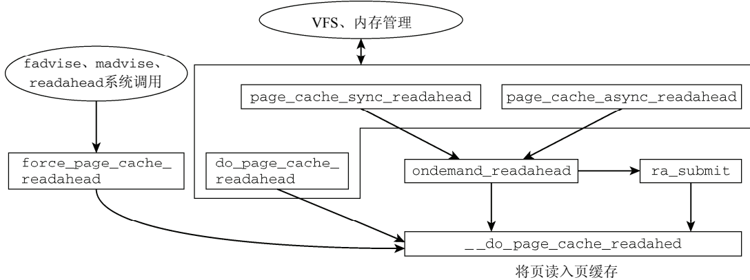
图16-5 用于实现预读的函数。请注意，图中虽然给出了各个函数之间的关联，但并不是一个正确的代码流程图
