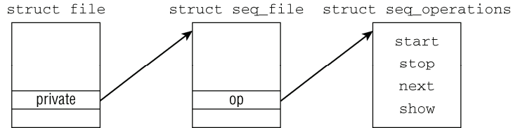
图10-8 顺序文件的数据结构
