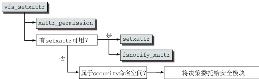
图11-3 vfs_setxattr的代码流程图
