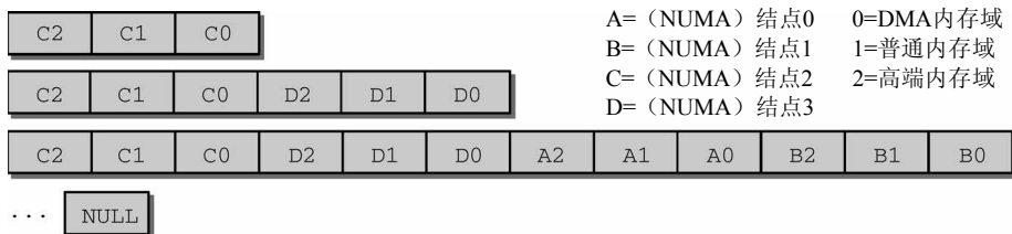
图3-9 连续填充备用列表
