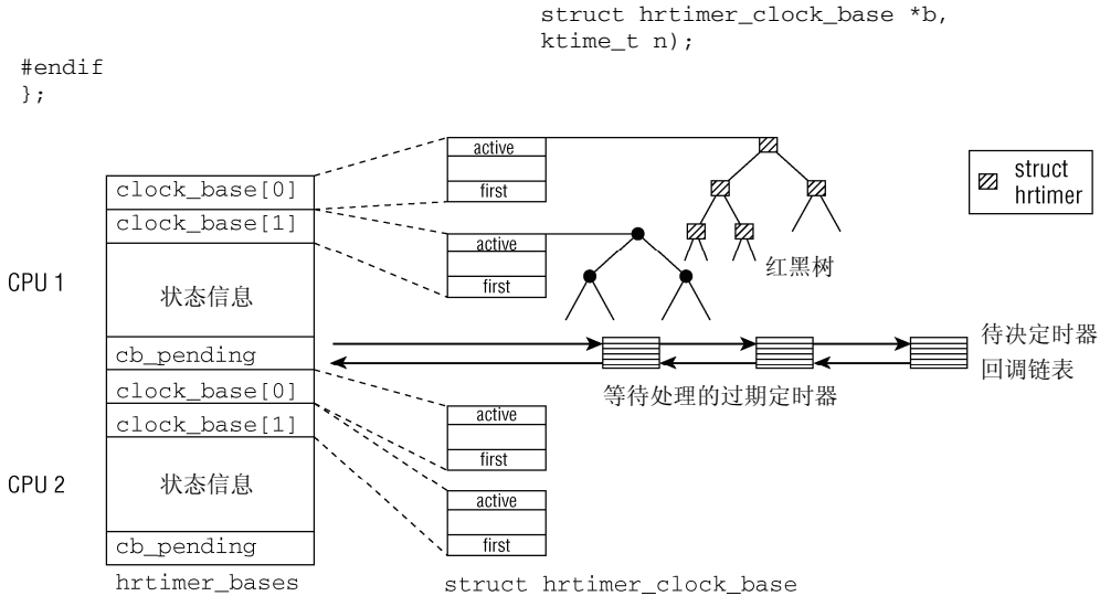
图15-12 用于实现高分辨率定时器的数据结构的概述
