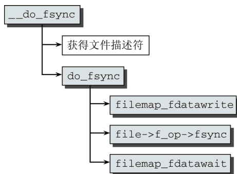
图17-12 __do_fsync 的代码流程图
