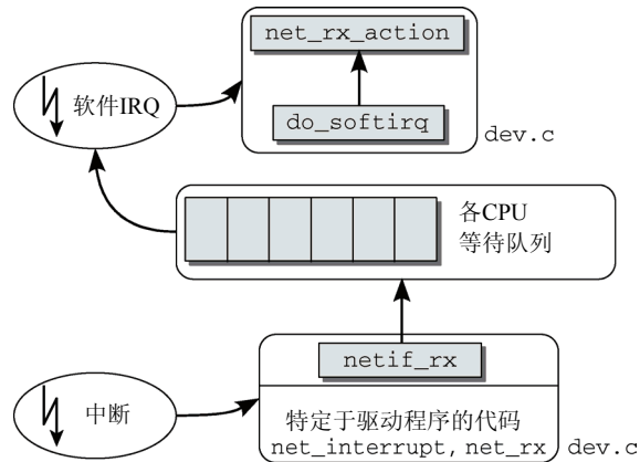
图12-10 接收到的分组穿过内核的路径
