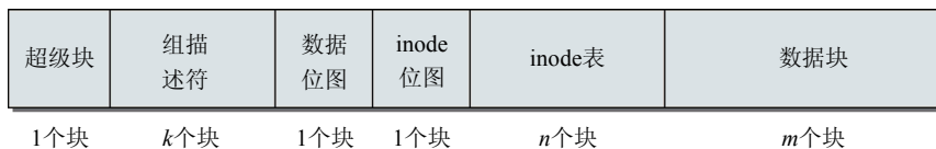
图9-2 Ext2文件系统的块组
