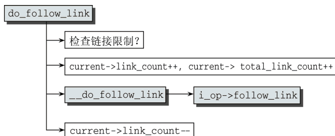
图8-10 do_follow_link的代码流程图
