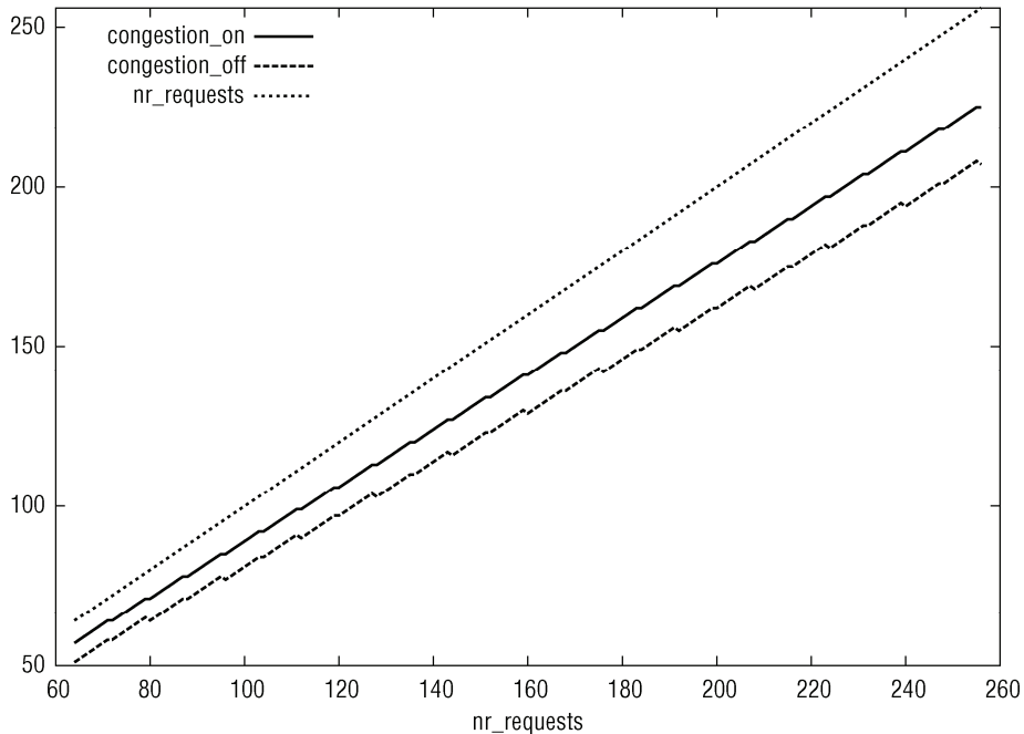
图17-9 拥塞现象出现和消失时，空闲请求数目的阈值。阈值显然总是小于队列中最大可容纳的请求数目
