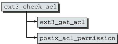
图11-12 ext3_check_acl 的代码流程图
