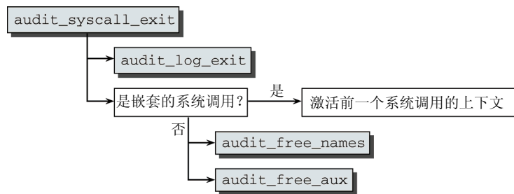
图19-9 audit_syscall_exit的代码流程图
