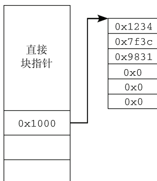
图9-11 ext2_get_branch 的返回值
