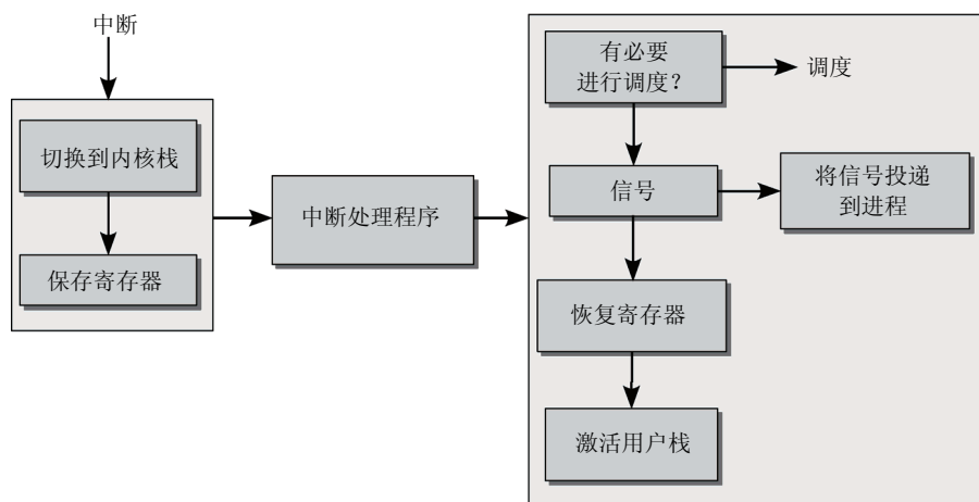
图14-2 中断的处理
