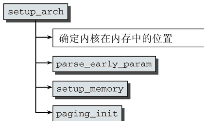
图D-2 IA-32系统上 setup_arch 的代码流程图
