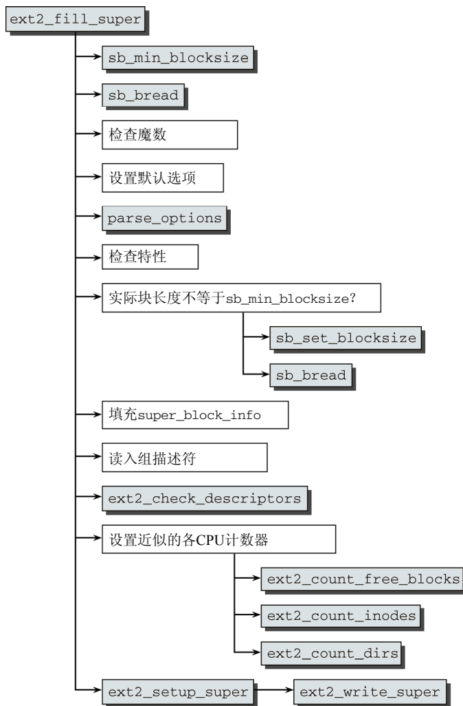
图9-8 ext2_fill_super 的代码流程图
