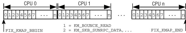
图3-42 利用固定映射来映射高端内存页
