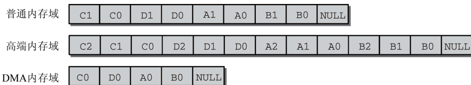
图3-10 完成的备用列表
