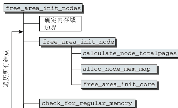
图3-28 free_area_init_nodes的代码流程图
