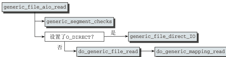
图8-13 generic_file_aio_read 的代码流程图
