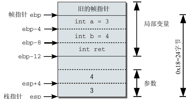
图C-2 调用add之前栈帧的状态
