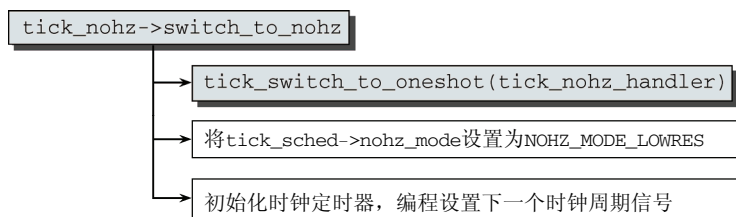
图15-19 tick_nohz_switch_to_nohz 的代码流程图
