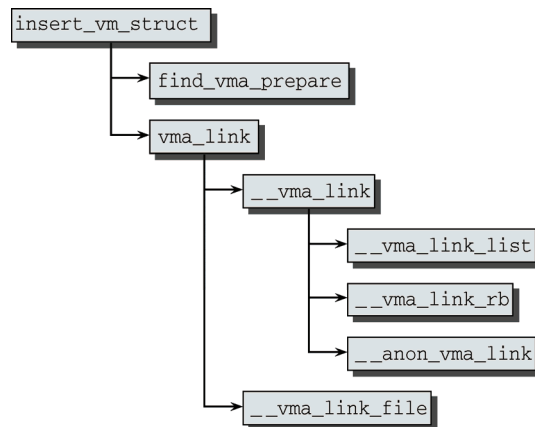
图4-11 insert_vm_struct 的代码流程图
