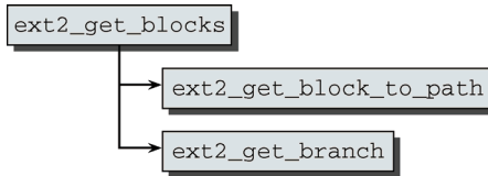
图9-9 ext2_get_block的代码流程图（读取一块）
