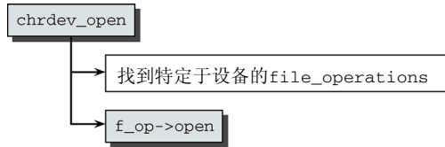
图6-6 chrdev_open的代码流程图
