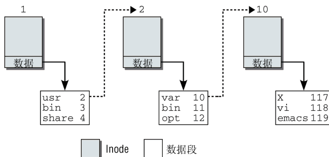
图8-2 查找/usr/bin/emacs的操作
