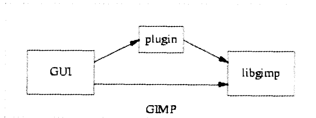
图 4.2 载入插件的 GIMP 中调用和被调用关系图
