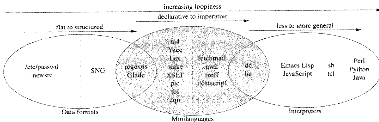
图 8.1 语言分类
