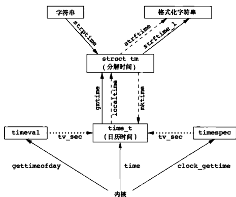
图 6-9 各个时间函数之间的关系
