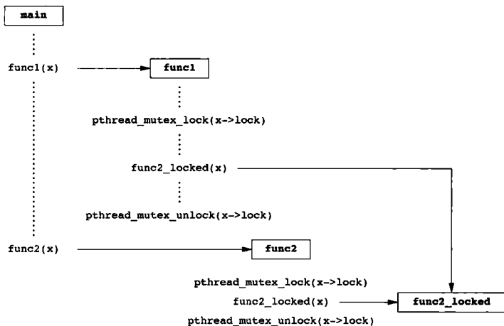
图 12-7 避免使用递归锁的一种可能情况
