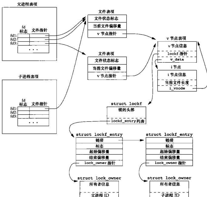
图 14-8 关于记录锁的 FreeBSD 数据结构
