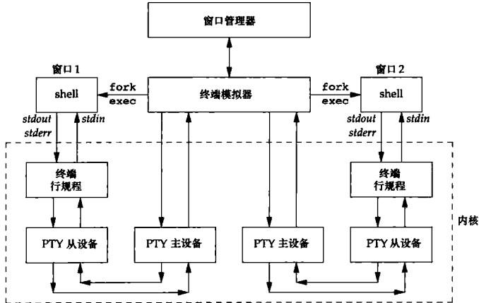
图 19-4 窗口系统的进程安排
