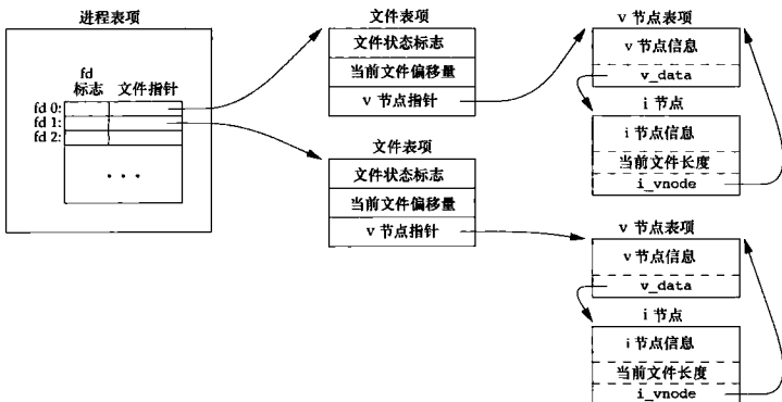
图 3-7 打开文件的内核数据结构
