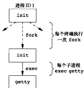
图 9-1 为允许终端登录, init 调用的进程
