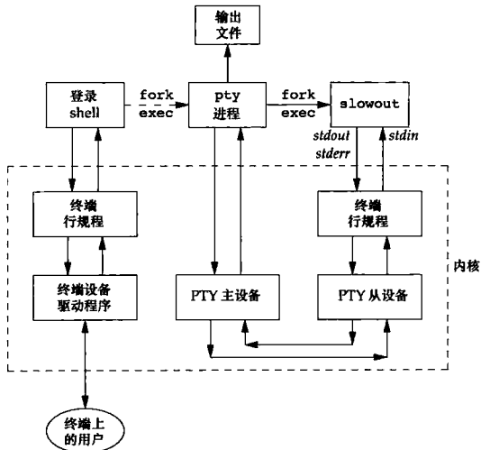
图 19-7 使用伪终端运行一个缓慢输出的程序
