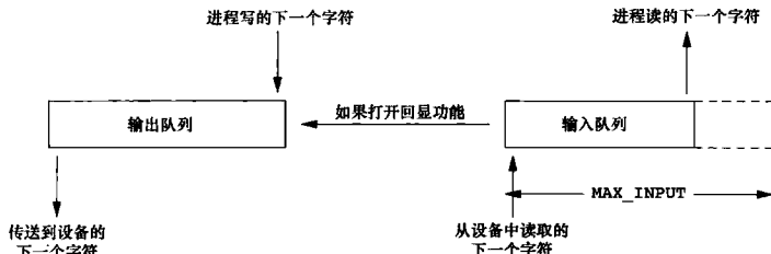
图 18-1 终端设备的输入、输出队列的逻辑结构
