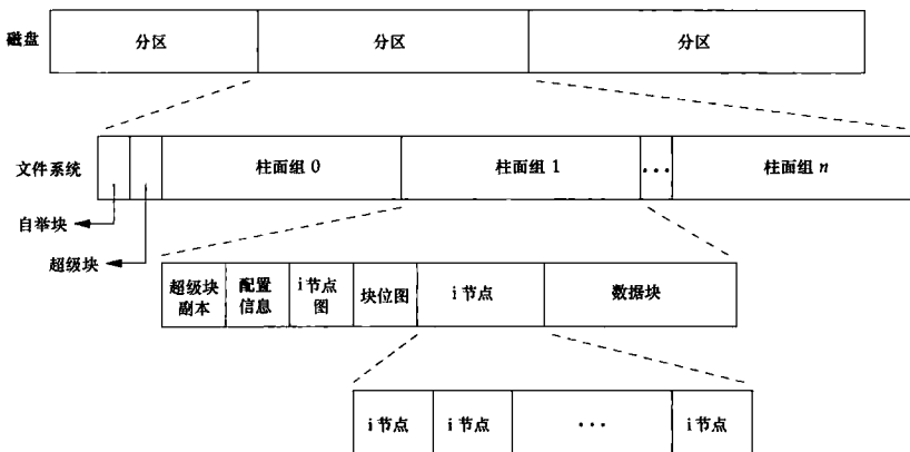
图 4-13 磁盘、分区和文件系统
