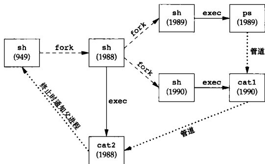
图 9-10 Bourne shell 执行程序 ps | cat1 | cat2 时的进程
