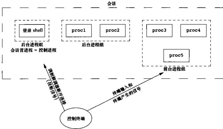
图 9-7 进程组、会话和控制终端
