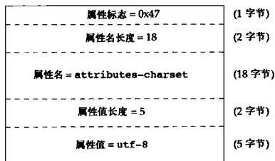
图 21-4 IPP 属性编码样例
