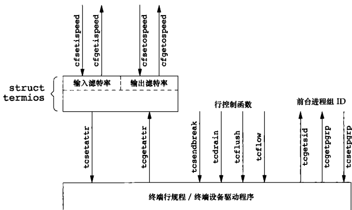
图 18-8 与终端有关的各函数之间的关系
