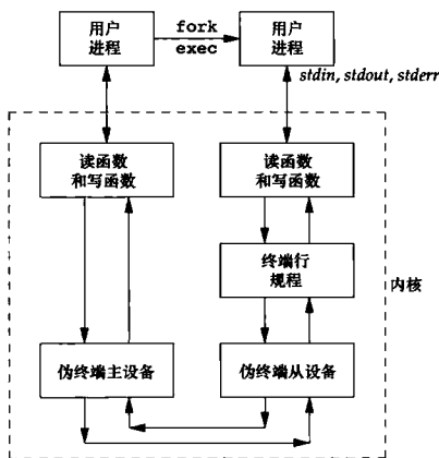
图 19-1 使用伪终端的相关进程的典型结构
