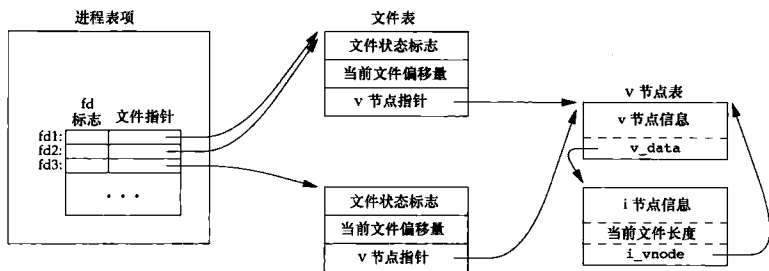
图 C-2 open 和 dup 的结果
