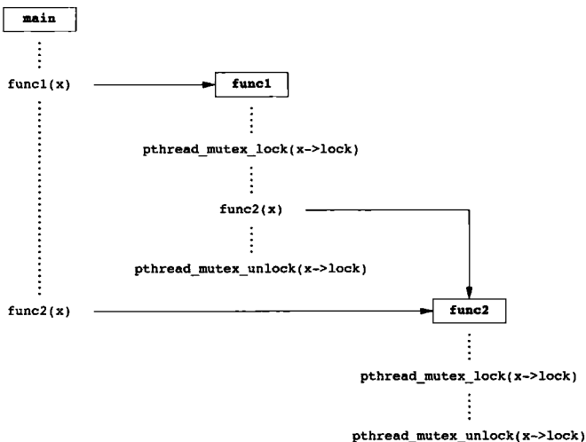
图 12-6 使用递归锁的一种可能情况
