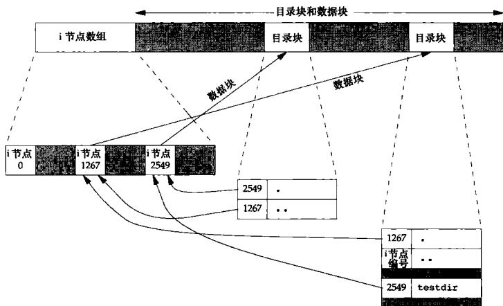
图 4-15 创建了目录 testdir 后的文件系统实例
