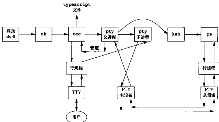
图 19-14 script shell 脚本的进程安排
