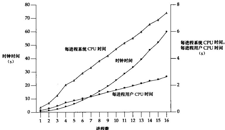
图 20-9 图 20-8 中使用建议性细粒度锁的数据
