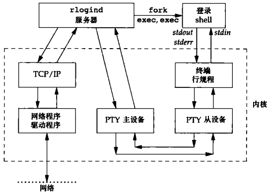
图 19-3 rlogind 服务器的进程安排
