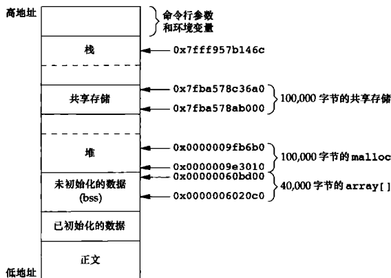
图 15-32 在基于 Intel 的 Linux 系统上的存储区布局
