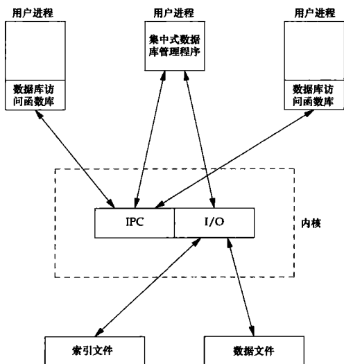
图 20-4 集中式数据库访问
