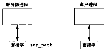
图 17-6 connect 之前的客户端套接字和服务端套接字
