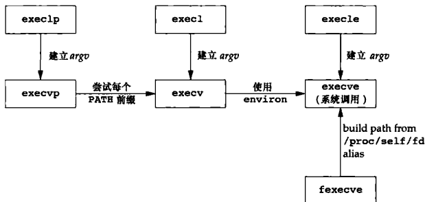
图 8-15 7 个 exec 函数之间的关系
