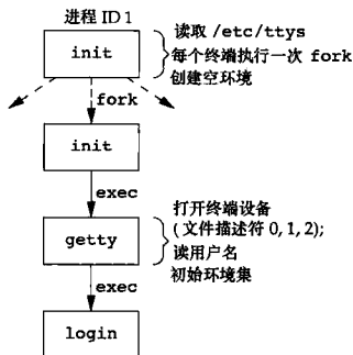
图 9-2 login 调用后进程的状态
