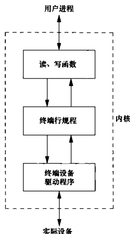
图 18-2 终端行规程
