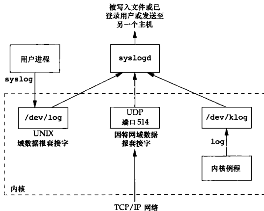
图 13-2 BSD 的 syslog 设施
