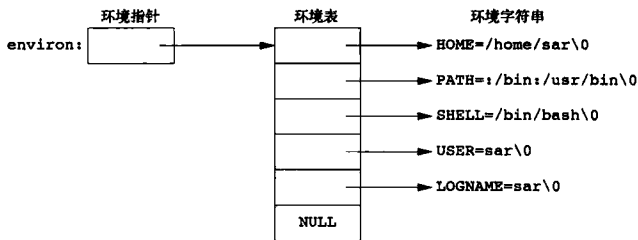
图 7-5 由 5 个字符串组成的环境
