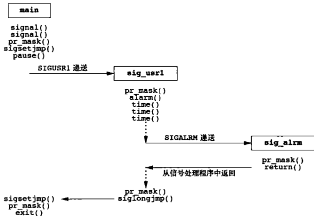
图 10-21 处理两个信号的实例程序的时间顺序
