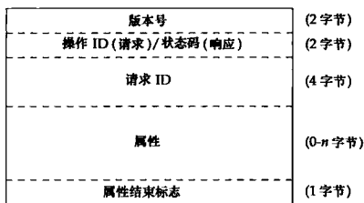
图 21-3 IPP 首部结构
