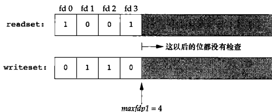
图 14-16 select 的样本描述符集
