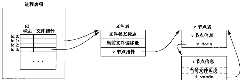
图 3-9 dup(1) 后的内核数据结构
