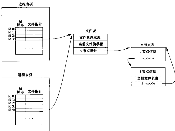
图 17-11 从顶部进程传送一个打开文件至底部进程
