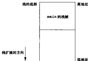
图 7-12 在调用 longjmp 后的栈帧
