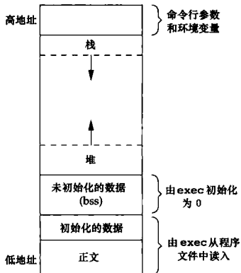
图 7-6 典型的存储空间安排
