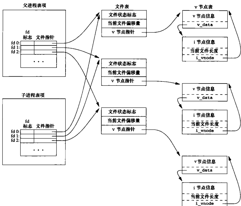
图 8-2 fork 之后父进程和子进程之间对打开文件的共享
