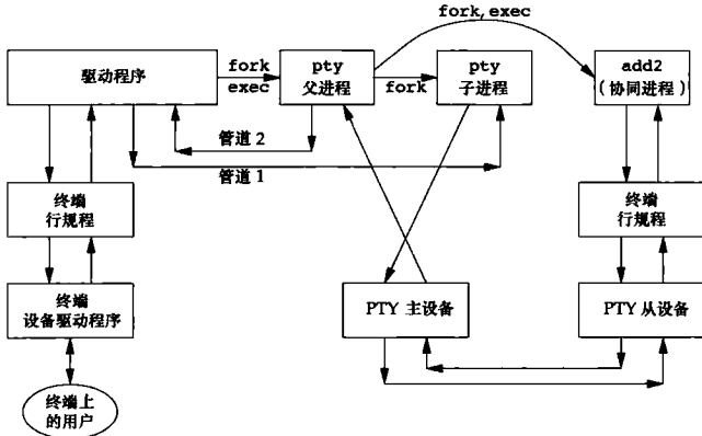
图 19-15 运行一个协同进程，以伪终端作为其输入和输出
