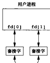
图 17-1 套接字对
