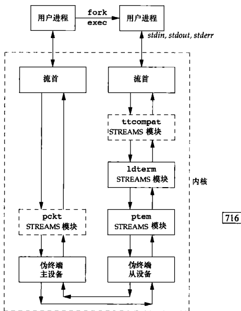
图 19-2 Solaris 中的伪终端安排
