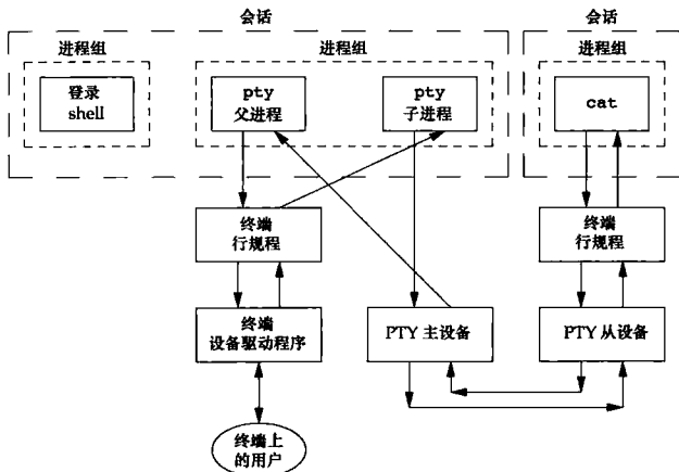
图 19-13 pty cat 的进程组和会话
