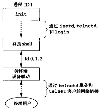
图 9-5 网络登录完成各种设置后的进程安排
