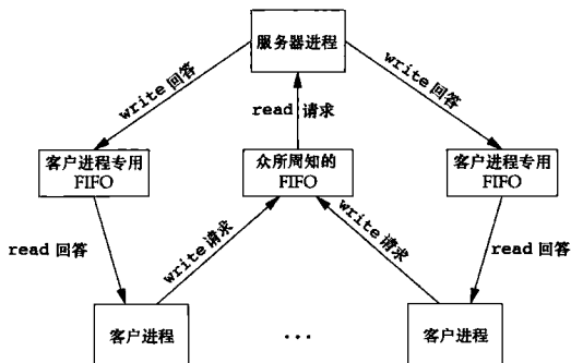
图 15-23 用 FIFO 进行客户进程-服务器进程通信
