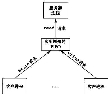
图 15-22 客户进程用 FIFO 向服务器进程发送请求
