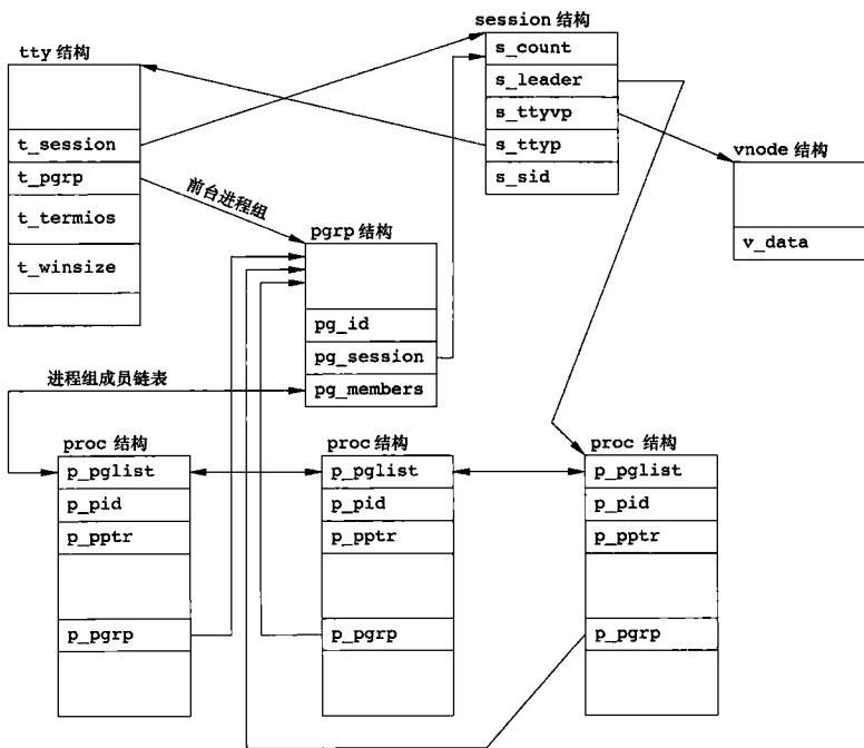
图 9-13 会话和进程组的 FreeBSD 实现
