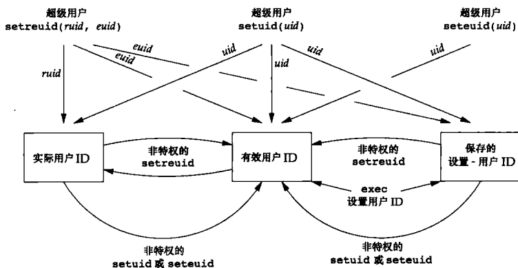
图 8-19 设置不同用户 ID 的各函数
