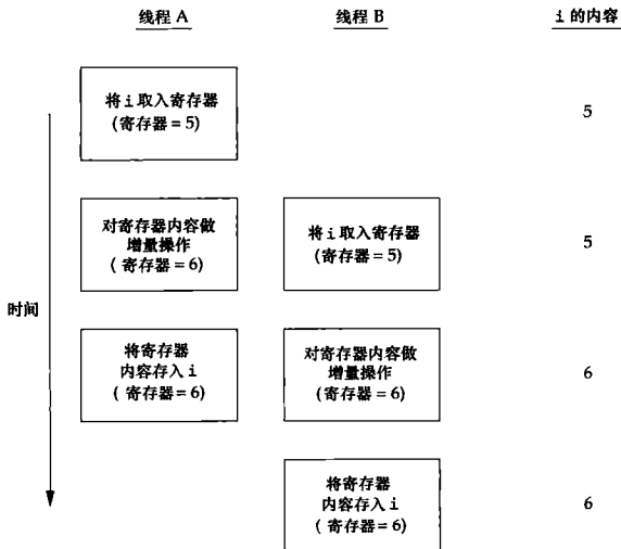
图 11-9 两个非同步的线程对同一个变量做增量操作
