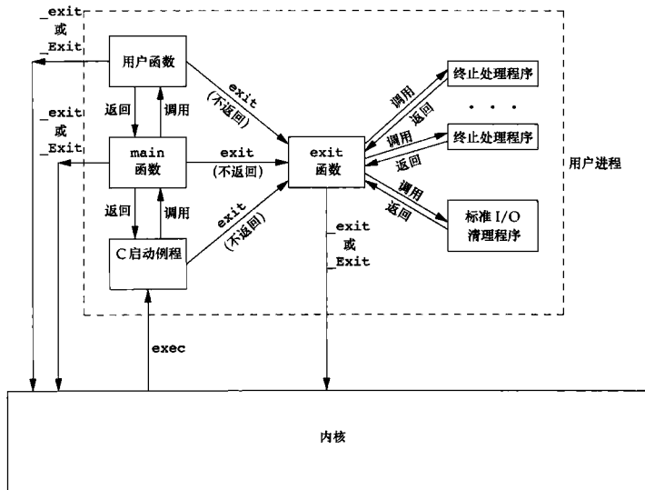
图 7-2 一个 C 程序是如何启动和终止的
