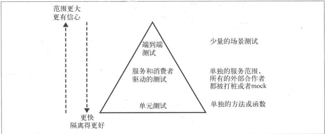
图 7-10: 把消费者契约的测试集成到测试金字塔
