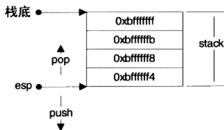
图 10-3 程序栈实例
