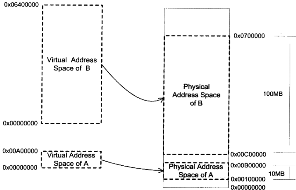
图 1-5 段映射机制
