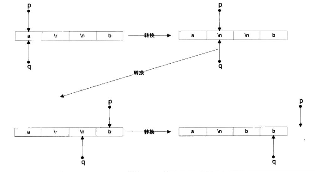
图 11-14 换行符转换
