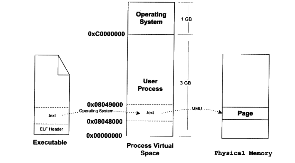
图 6-6 页错误
