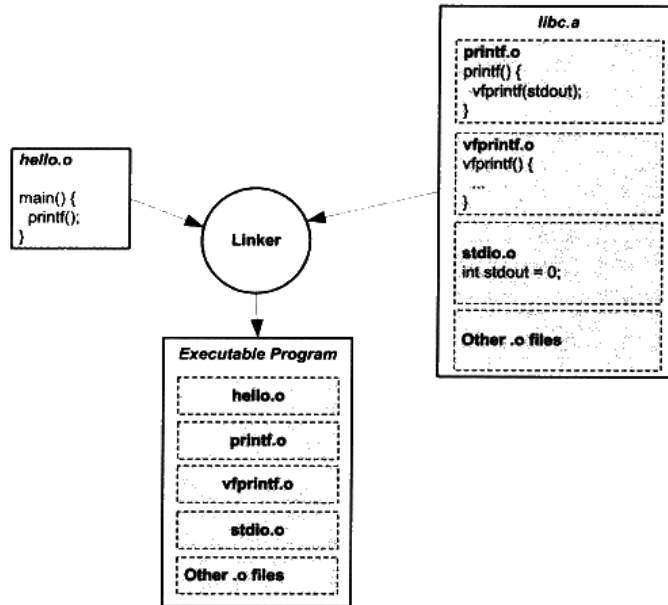
图 4-6 静态库链接
