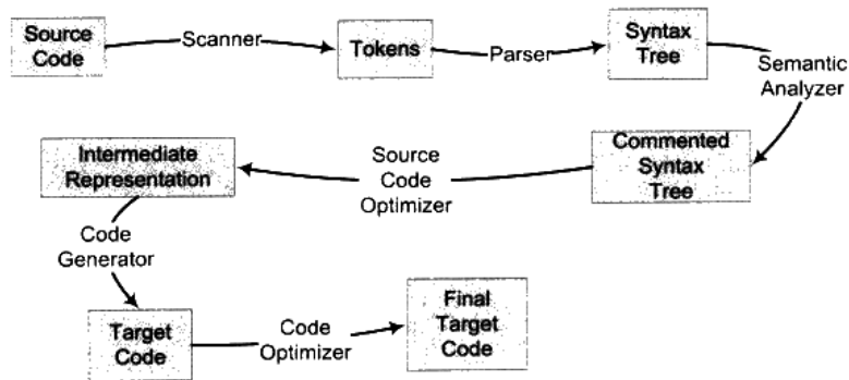
图 2-2 编译过程
