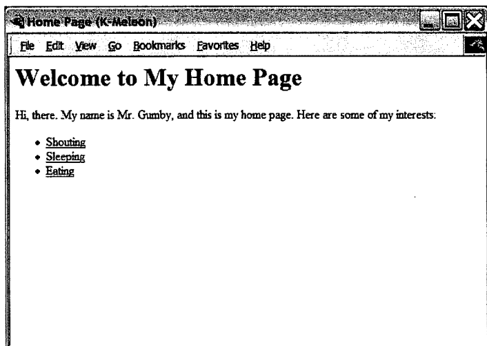
图22-1 生成的网页
