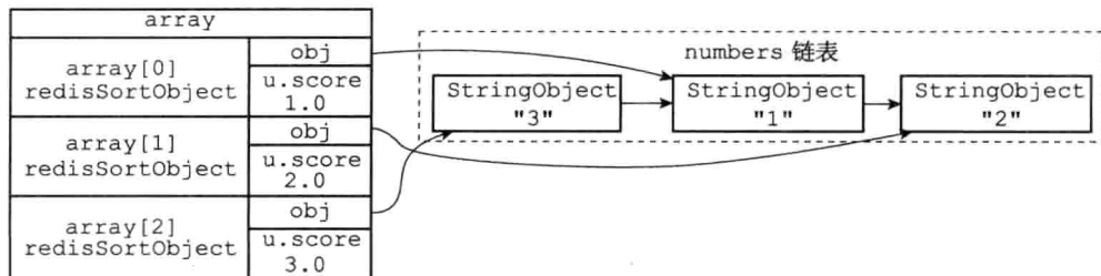
图 21-7 执行升序排序的数组
