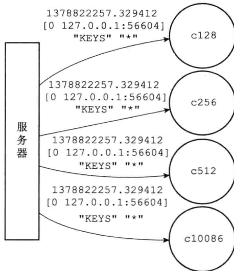
图 24-4 服务器将信息发送给各个监视器
