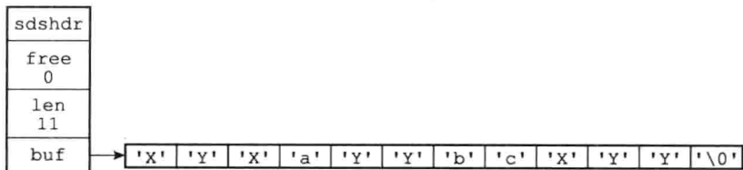
图 2-14 执行 sdstrim 之前的 SDS
