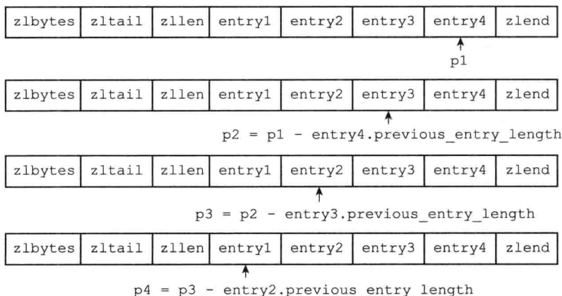
图 7-8 一个从表尾向表头遍历的例子
