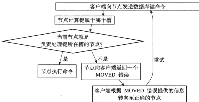
图 17-18 判断客户端是否需要转向的流程
