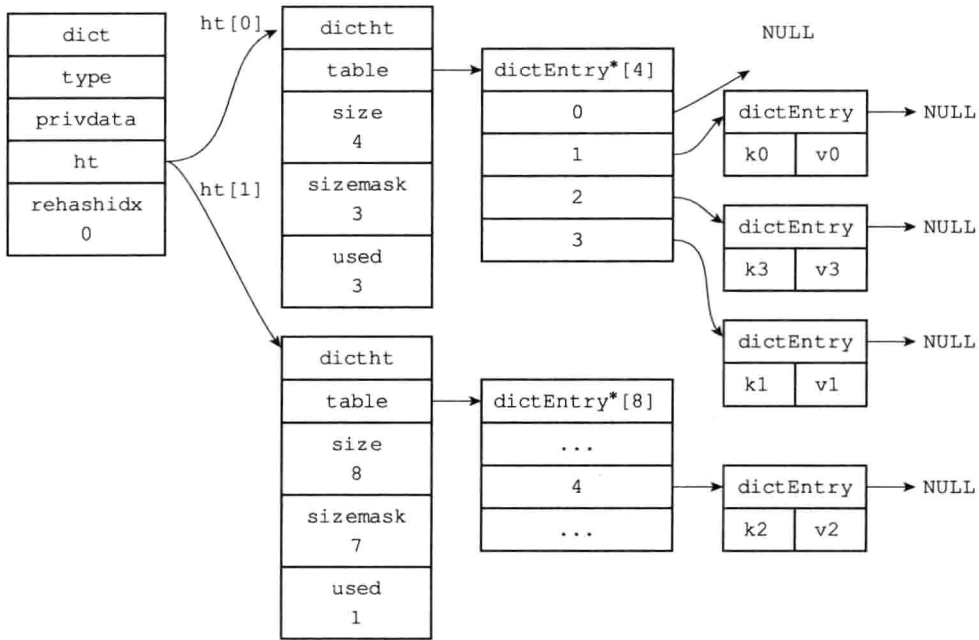
图 4-13 rehash 索引 0 上的键值对
