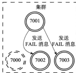
图 17-43 节点 7001 向集群广播 FAIL 消息
