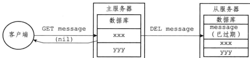
图 9-19 主从服务器删除过期键 (3)
