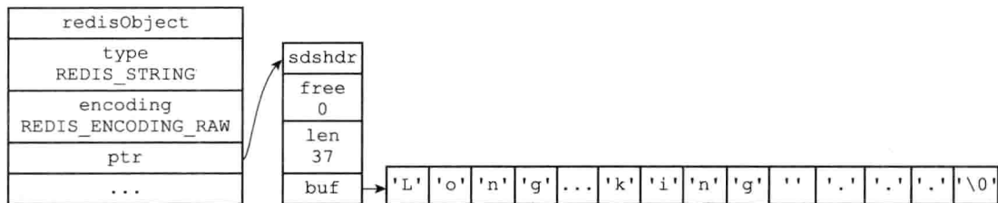
图 8-2 raw 编码的字符串对象
