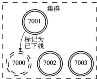
图 17-42 节点 7001 将节点 7000 标记为已下线
