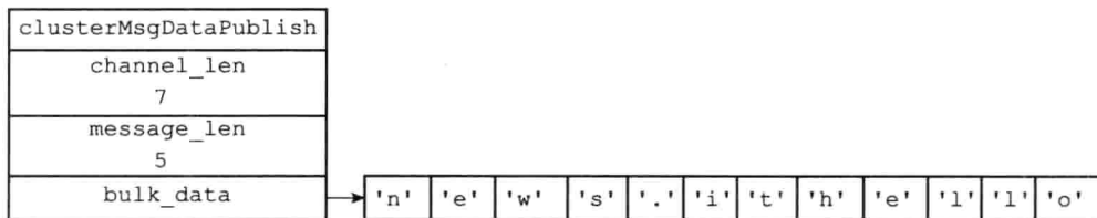
图 17-46 clusterMsgDataPublish 结构示例
