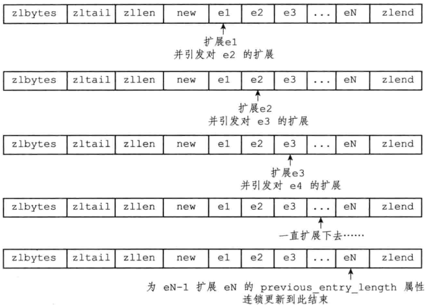
图 7-13 连锁更新过程
