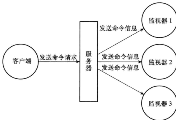
图 24-1 命令的接收和信息的发送
