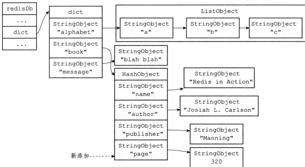
图 9-8 使用 HSET 更新 book 键
