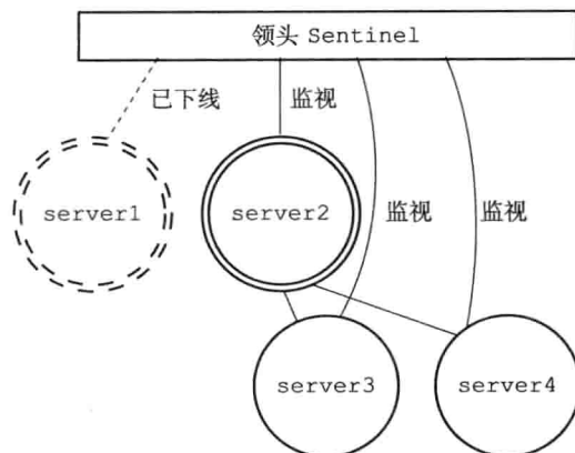
图 16-25 server3 和 server4 成为 server2 的从服务器
