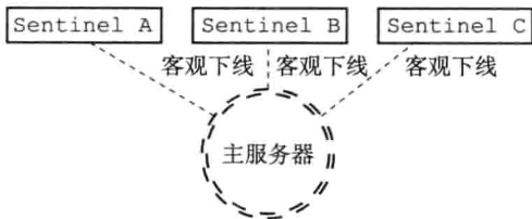
图 16-20 三个 Sentinel 都发现主服务器已经进入了客观下线状态
