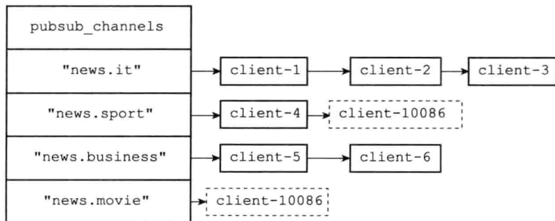
图 18-8 执行 UNSUBSCRIBE 之前的 pubsub_channels 字典
