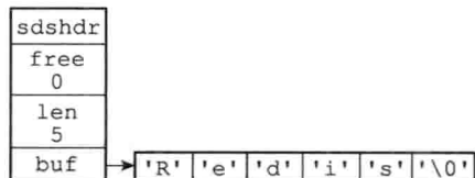
图 2-11 执行 sdscat 之前的 SDS
