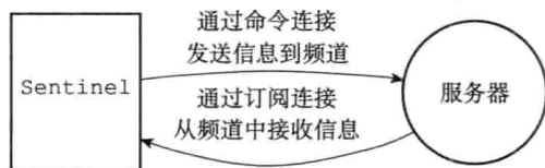
图 16-13 Sentinel 同时向服务器发送和接收信息
