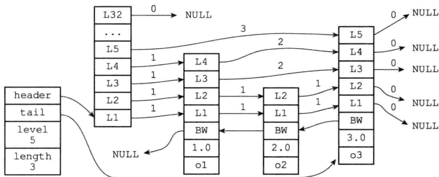
图 5-9 带有 zskiplist 结构的跳跃表
