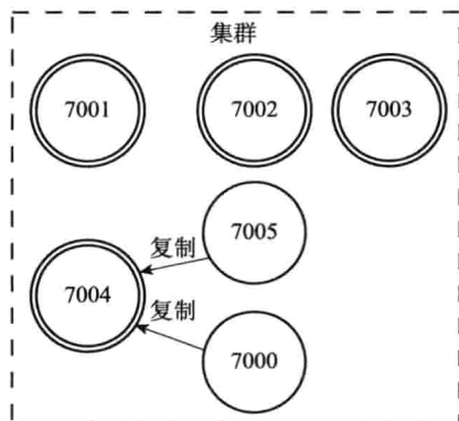
图 17-34 重新上线的节点 7000 成为节点 7004 的从节点
