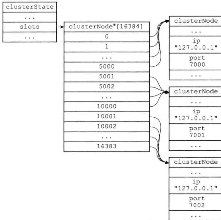
图 17-14 clusterState 结构的 slots 数组
