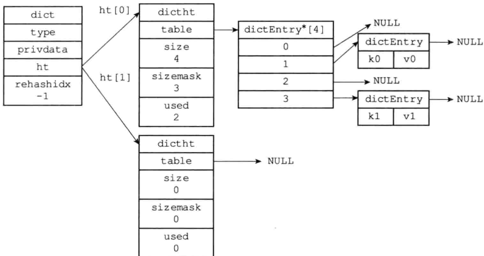
图 4-3 普通状态下的字典
