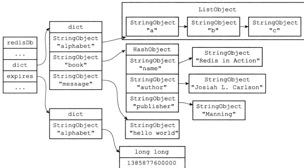
图 9-14 执行 PERSIST 之后的数据库
