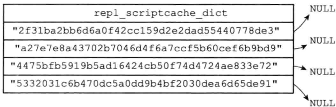
图 20-14 执行 EVALSHA 命令之后的 repl_scriptcache_dict 字典
