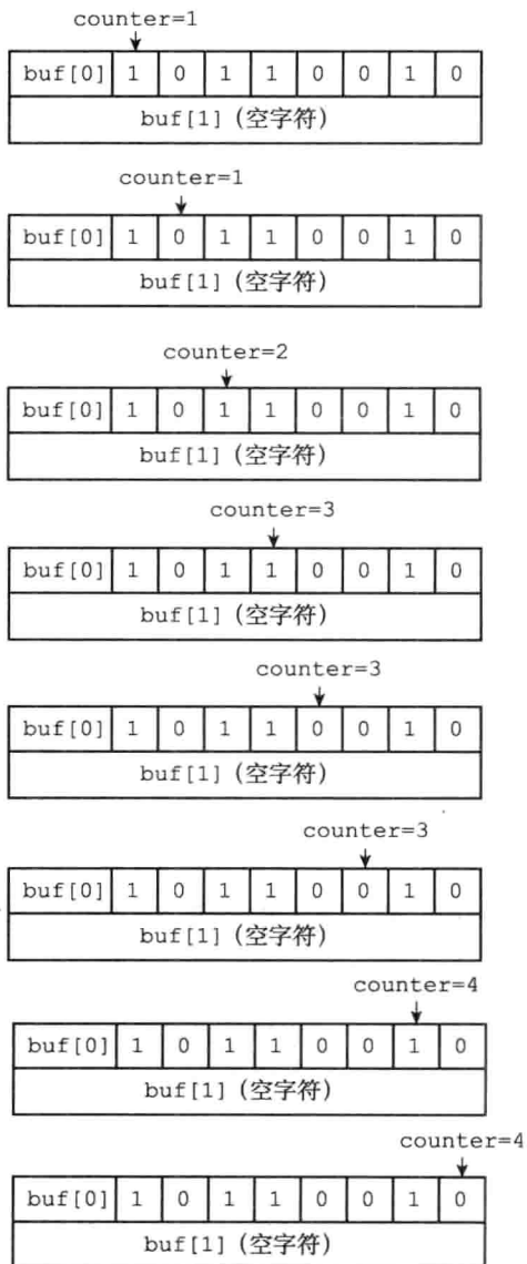
图 22-17 遍历算法的运行过程
