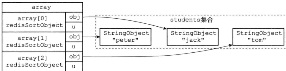
图 21-18 排序之后的数组
