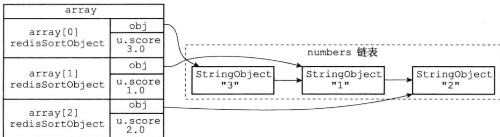
图 21-3 设置数组项的 u.score 属性
