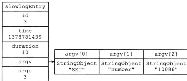
图 23-1 slowlogEntry 结构示例
