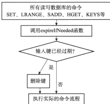
图 9-15 命令调用 expireIfNeeded 来删除过期键
