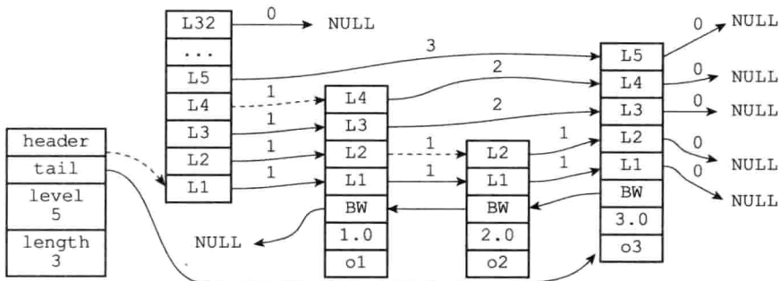
图 5-5 另一个计算节点排位的例子
