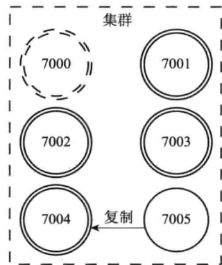
图 17-33 节点 7004 成为新的主节点
