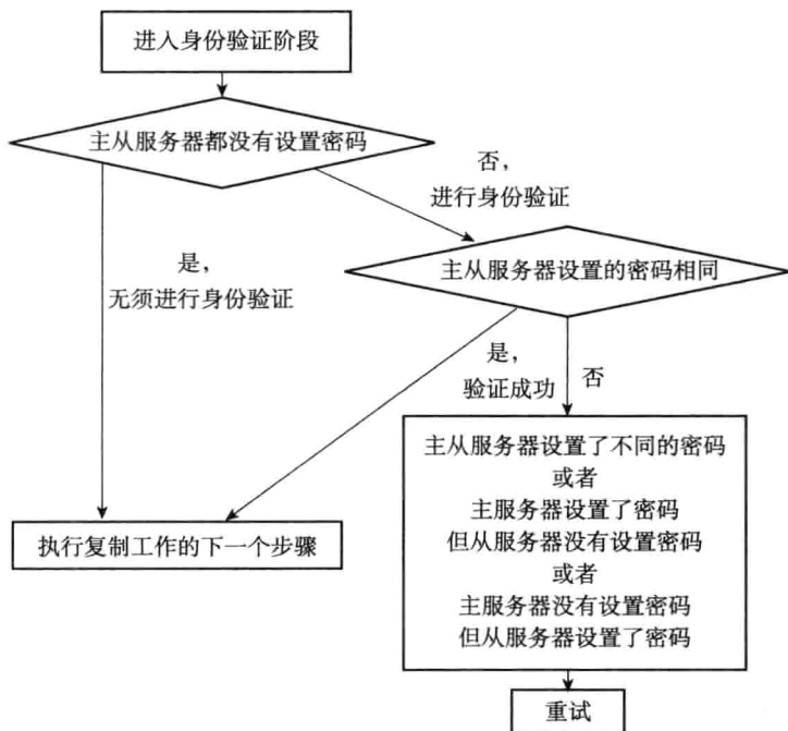
图 15-19 从服务器在身份验证阶段可能遇到的情况
