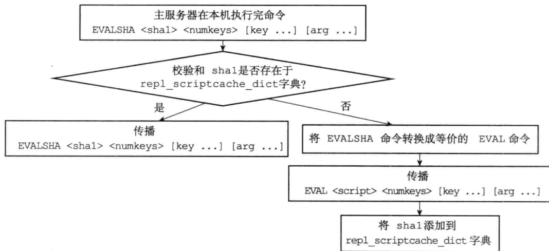
图 20-12 主服务器判断传播 EVAL 还是 EVALSHA 的过程
