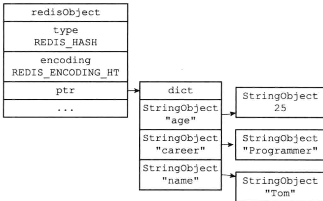
图 8-11 hashtable 编码的 profile 哈希对象
