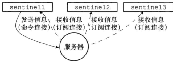
图 16-14 向服务器发送信息
