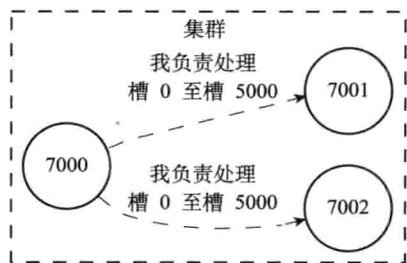
图 17-11 7000 告知 7001 和 7002 自己负责处理的槽
