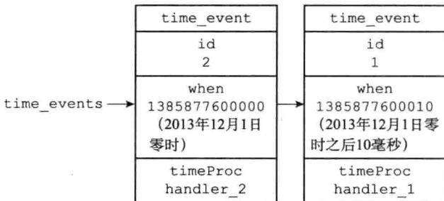
图 12-9 用链表连接起来的两个时间事件
