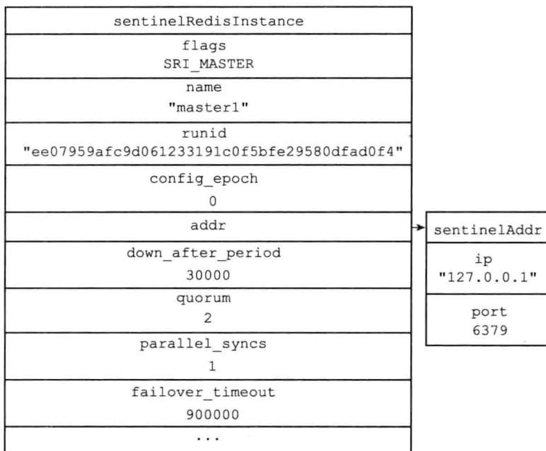
图 16-5 master1 的实例结构
