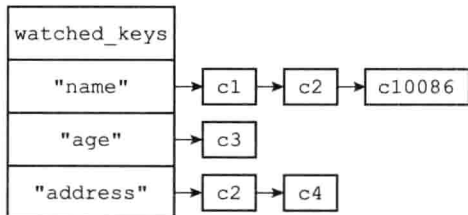
图 19-8 执行 WATCH 命令之后的 watched_keys 字典
