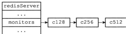
图 24-2 客户端 c10086 执行 MONITOR 命令之前的 monitors 链表
