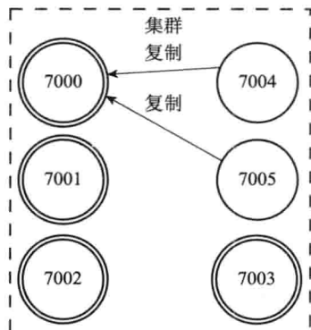
图 17-32 设置节点 7004 和节点 7005 成为节点 7000 的从节点
