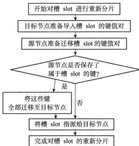
图 17-25 对槽 slot 进行重新分片的过程
