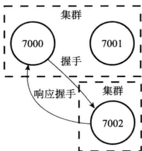
图 17-4 节点 7000 与节点 7002 进行握手
