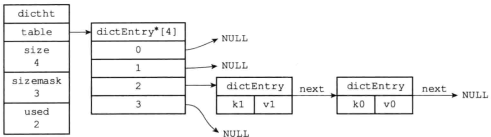
图 4-2 连接在一起的键 k1 和键 k0
