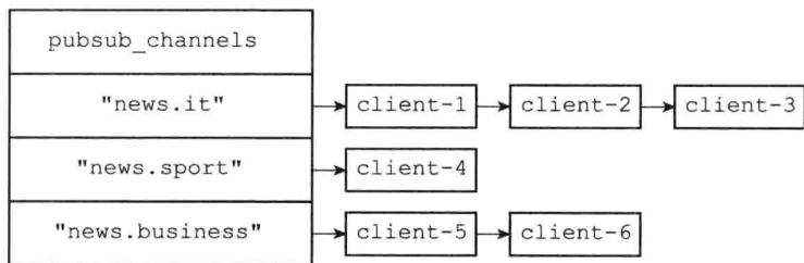
图 18-6 一个 pubsub_channels 字典示例
