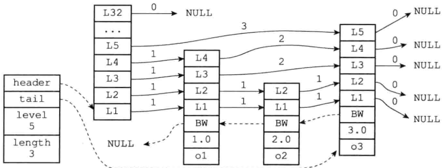
图 5-6 从表尾向表头方向遍历跳跃表
