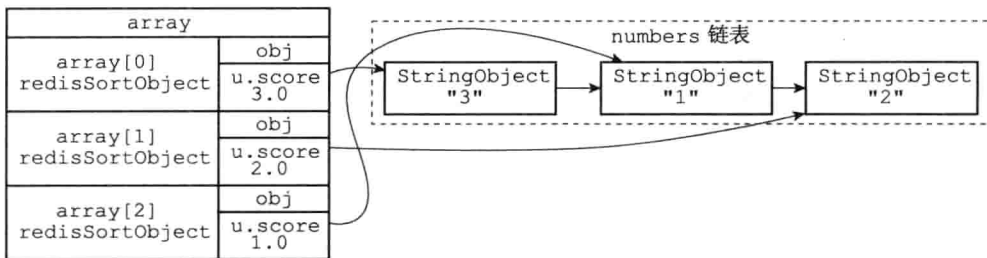
图 21-8 执行降序排序的数组
