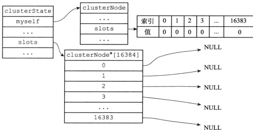
图 17-16 节点的 clusterState 结构
