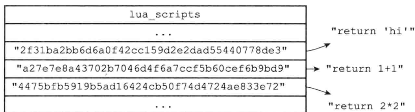
图 20-4 lua_scripts 字典示例
