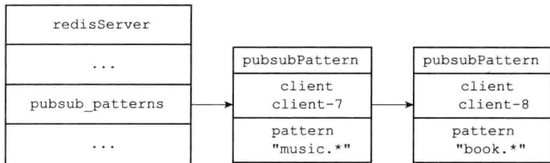
图 18-15 执行 PUNSUBSCRIBE 命令之后的 pubsub_patterns 链表
