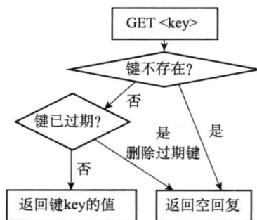
图 9-16 GET 命令的执行过程
