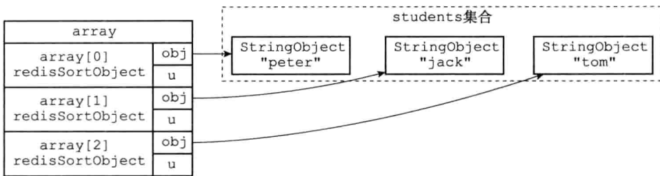
图 21-17 排序之前的数组
