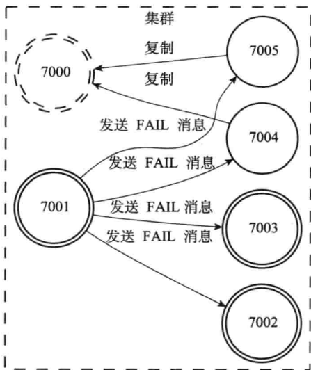
图 17-39 节点 7001 向集群广播 FAIL 消息
