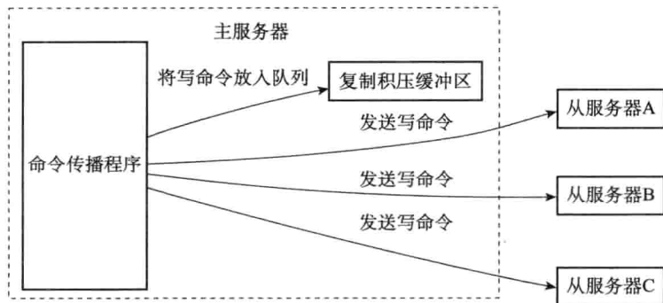
图 15-10 主服务器向复制积压缓冲区和所有从服务器传播写命令数据
