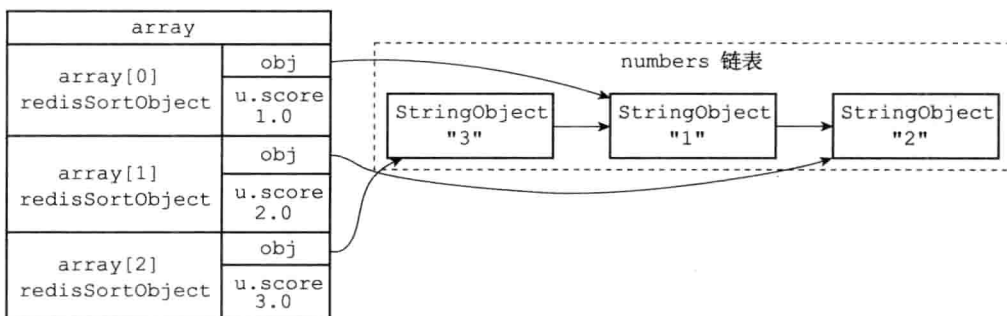
图 21-4 排序后的数组
