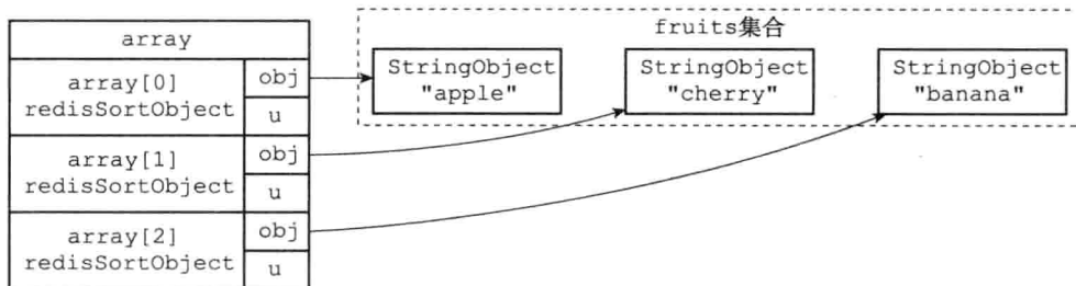
图 21-12 将 obj 指针指向集合的各个元素
