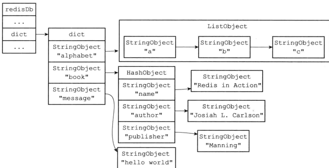
图 9-4 数据库键空间例子
