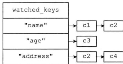
图 19-3 一个 watched_keys 字典
