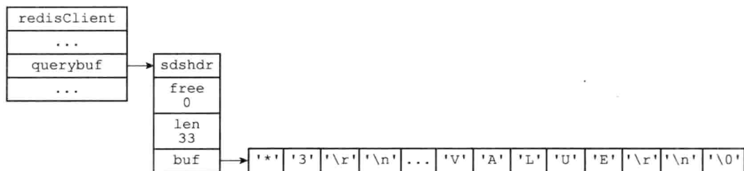
图 14-2 客户端状态中的命令请求
