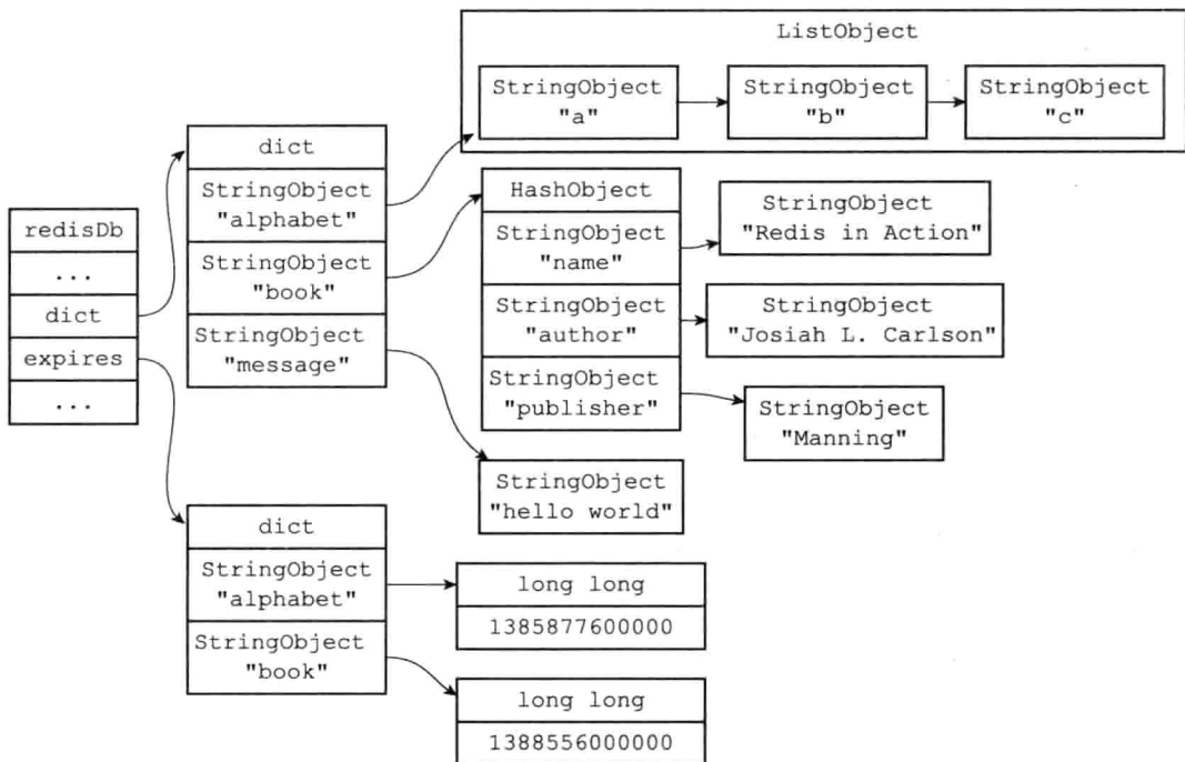
图 9-12 带有过期字典的数据库例子
