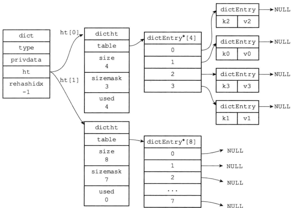
图 4-12 准备开始 rehash
