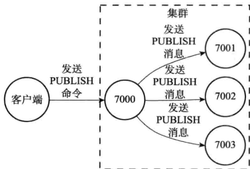
图 17-45 接收到 PUBLISH 命令的节点 7000 向集群广播 PUBLISH 消息
