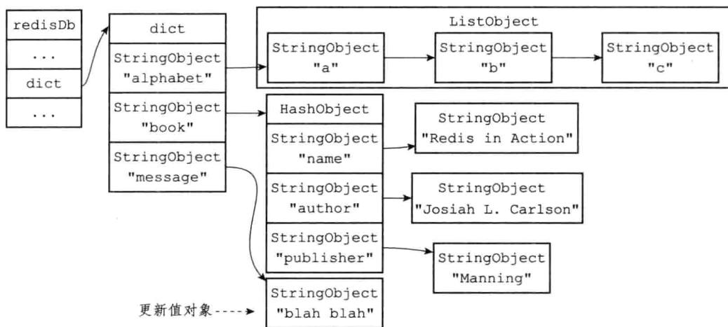
图 9-7 使用 SET 命令更新 message 键
