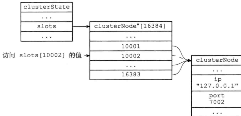
图 17-15 访问 slots[10002] 的值
