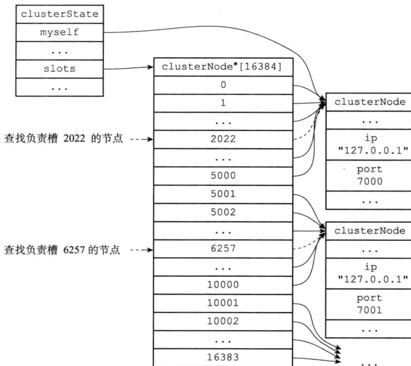
图 17-19 节点 7000 的 clusterState 结构
