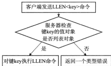
图 8-18 LLEN 命令执行时的类型检查过程
