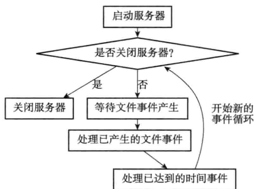
图 12-10 事件处理角度下的服务器运行流程
