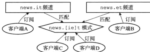
图 18-3 频道和模式的订阅状态
