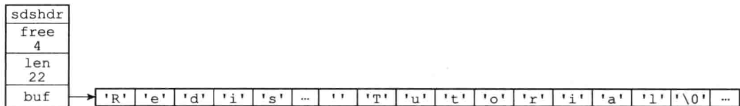
图 2-13 再次执行 sdscat 之后的 SDS
