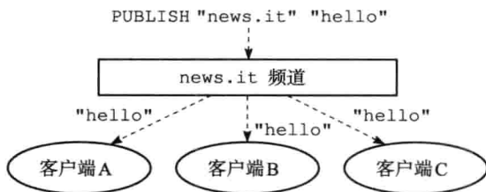
图 18-2 向 news.it 频道发送消息
