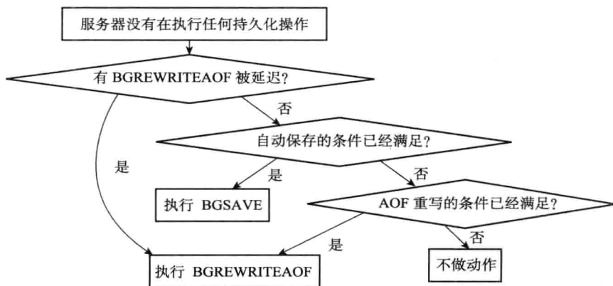
图 14-9 判断是否需要执行持久化操作
