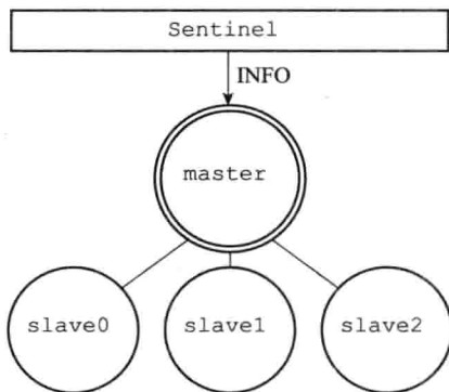
图 16-9 Sentinel 向带有三个从服务器的主服务器发送 INFO 命令
