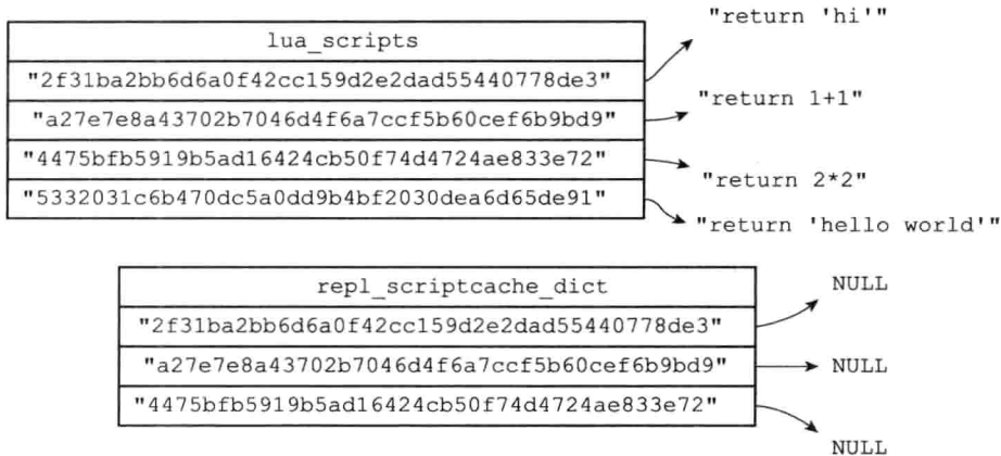
图 20-13 执行 EVALSHA 命令之前的 lua_scripts 字典和 repl_scriptcache_dict 字典
