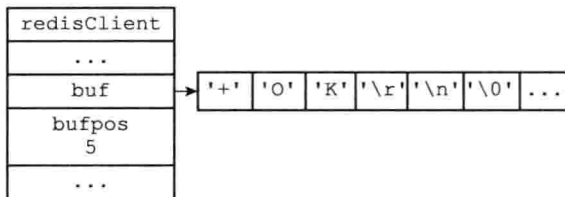
图 13-8 固定大小缓冲区示例
