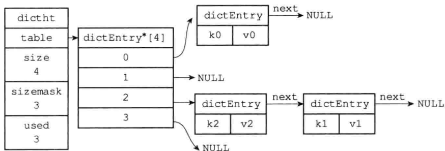
图 4-7 使用链表解决 k2 和 k1 的冲突
