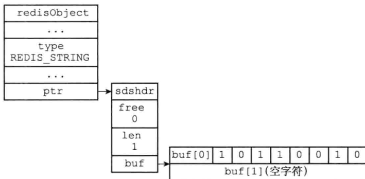
图 22-2 一字节长的位数组的 SDS 表示
