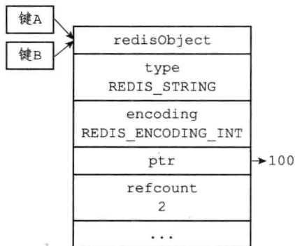
图 8-21 被共享的字符串对象
