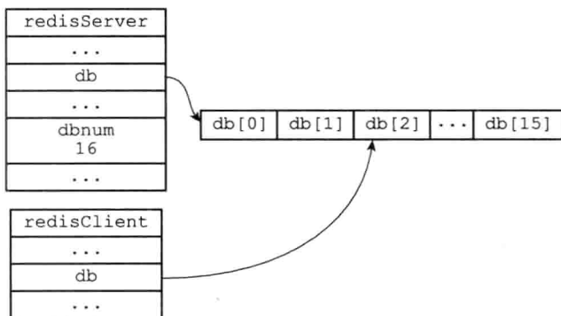
图 9-3 客户端的目标数据库为 2 号数据库
