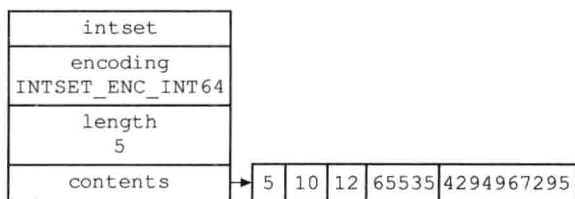
图 6-11 数组编码为 INTSET_ENC_INT64 的整数集合
