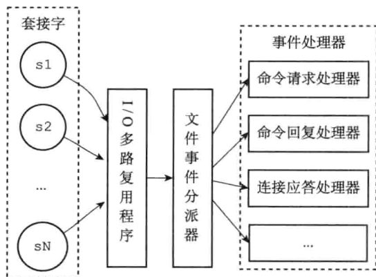
图 12-1 文件事件处理器的四个组成部分
