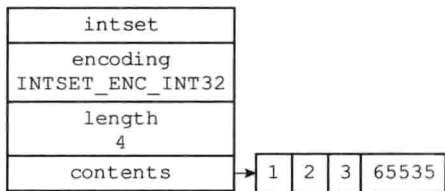
图 6-10 完成添加操作之后的整数集合
