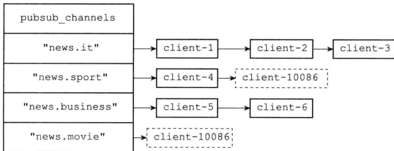
图 18-7 执行 SUBSCRIBE 之后的 pubsub_channels 字典
