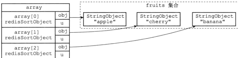
图 21-5 将 obj 指针指向集合的各个元素
