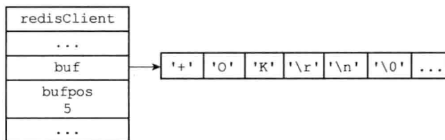
图 14-7 保存了命令回复的客户端状态
