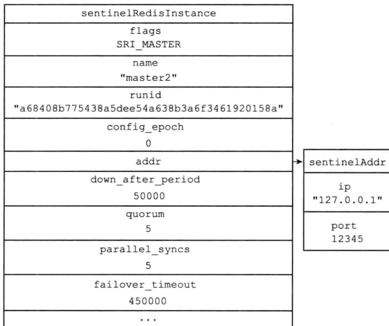
图 16-6 master2 的实例结构
