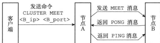
图 17-8 节点的握手过程
