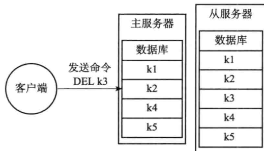
图 15-4 处于不一致状态的主从服务器
