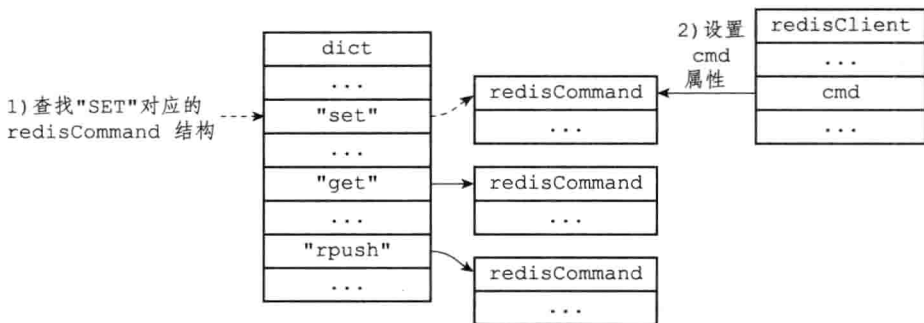
图 13-7 查找命令并设置 cmd 属性
