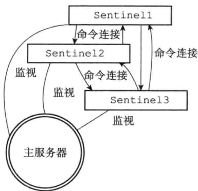
图 16-16 各个 Sentinel 之间的网络连接
