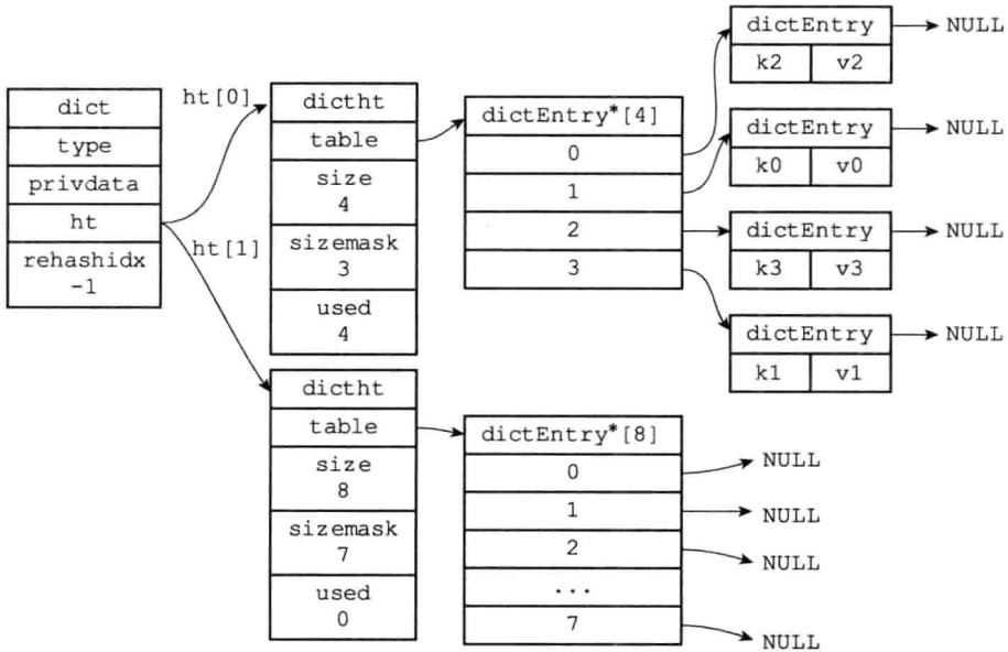
图 4-9 为字典的 ht[1] 哈希表分配空间
