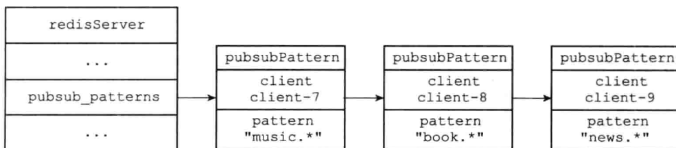
图 18-14 执行 PUNSUBSCRIBE 命令之前的 pubsub_patterns 链表
