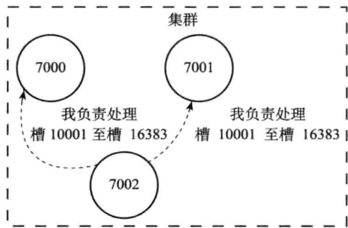
图 17-13 7002 告知 7000 和 7001 自己负责处理的槽
