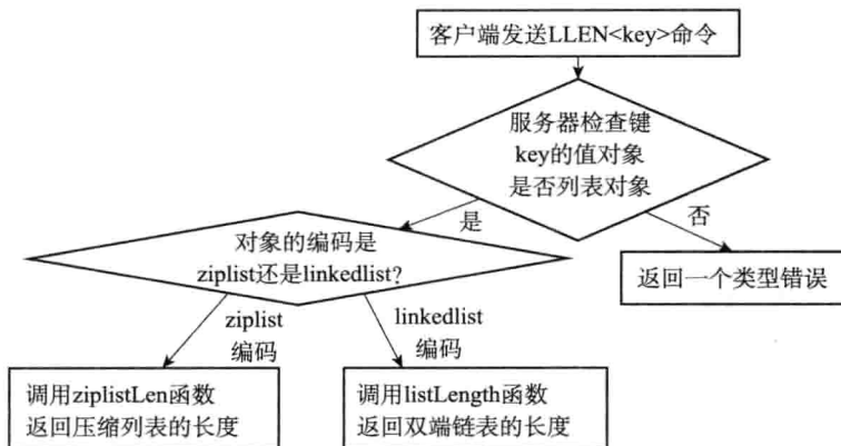
图 8-19 LLEN 命令的执行过程
