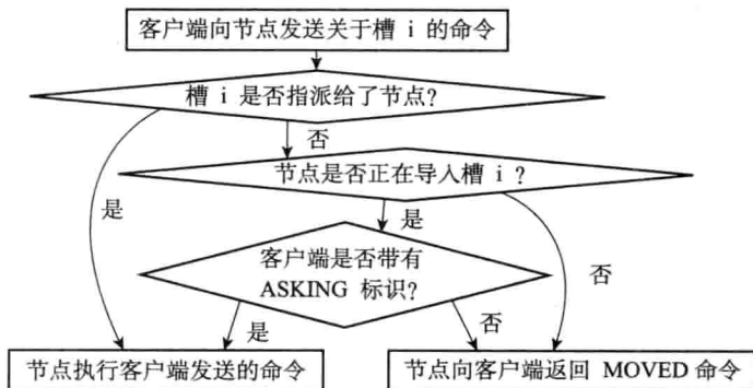
图 17-31 节点判断是否执行客户端命令的过程
