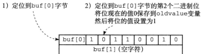
图 22-6 SETBIT 命令的执行过程
