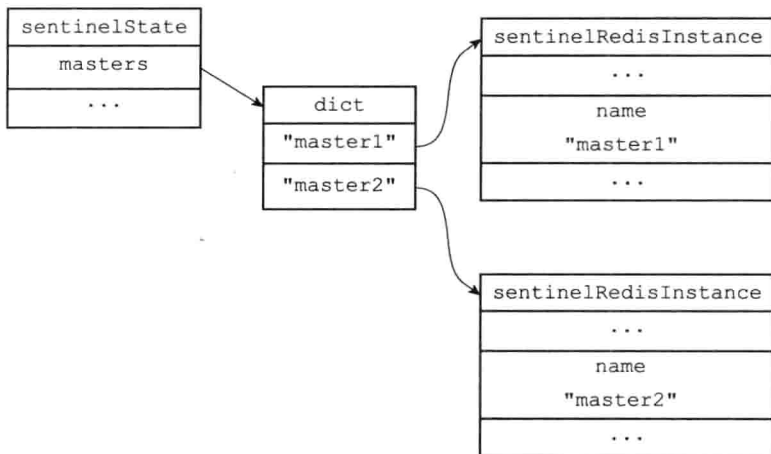
图 16-7 Sentinel 状态以及 masters 字典
