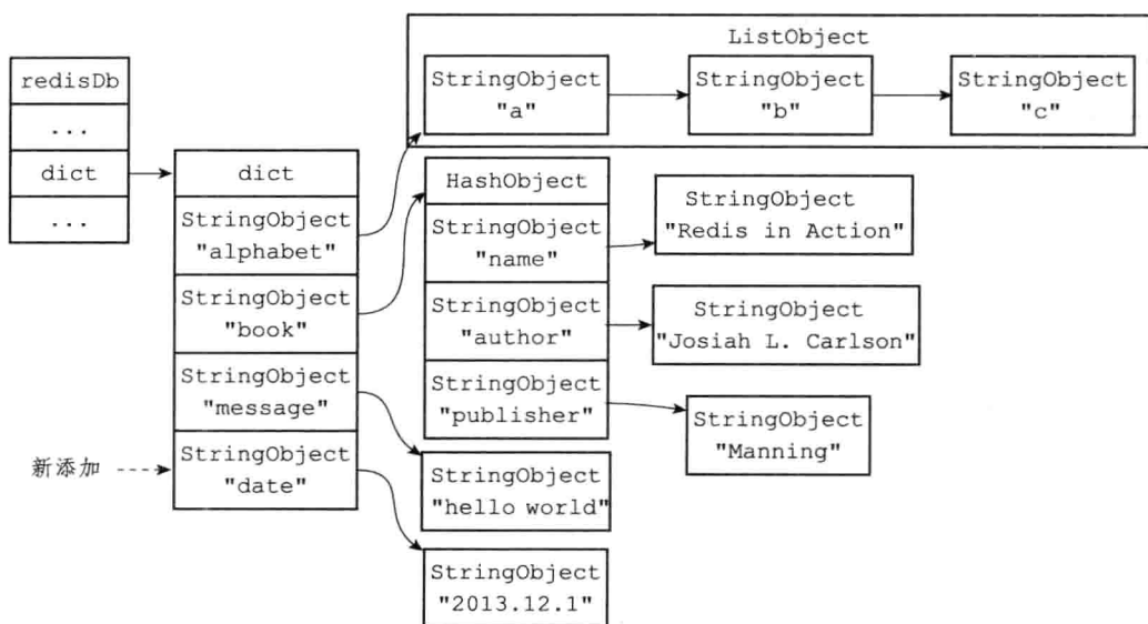
图 9-5 添加 date 键之后的键空间
