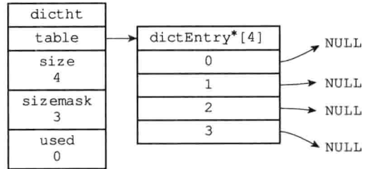
图 4-1 一个空的哈希表
