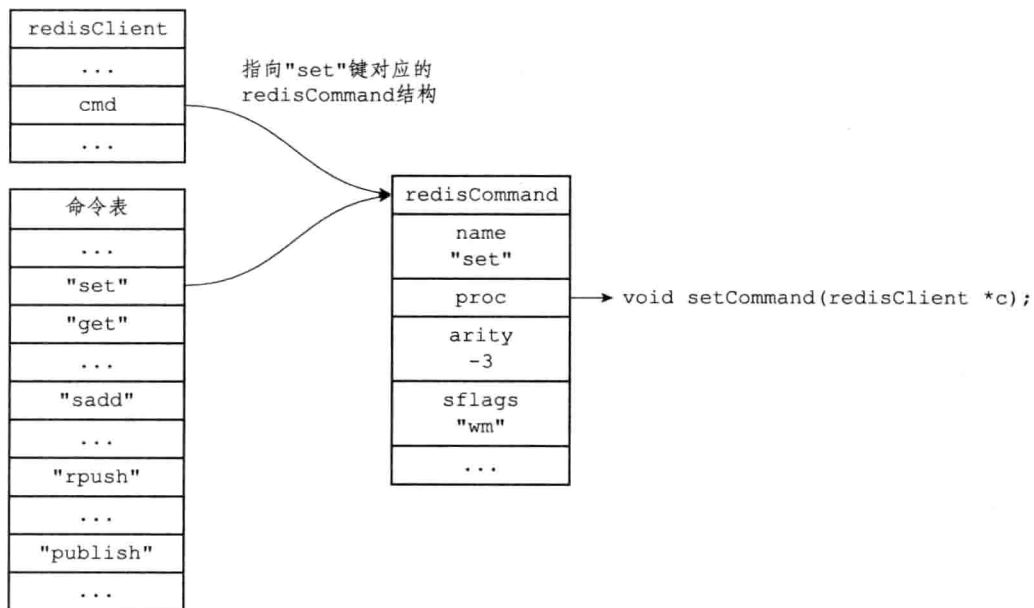
图 14-5 设置客户端状态的 cmd 指针
