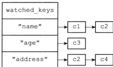
图 19-7 执行 WATCH 命令之前的 watched_keys 字典
