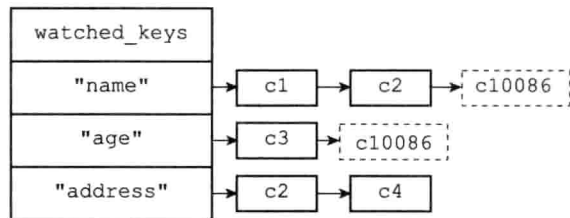
图 19-4 执行 WATCH 命令之后的 watched_keys 字典
