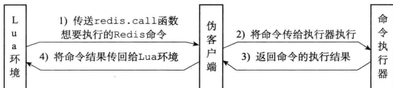
图 20-2 Lua 脚本执行 Redis 命令时的通信步骤
