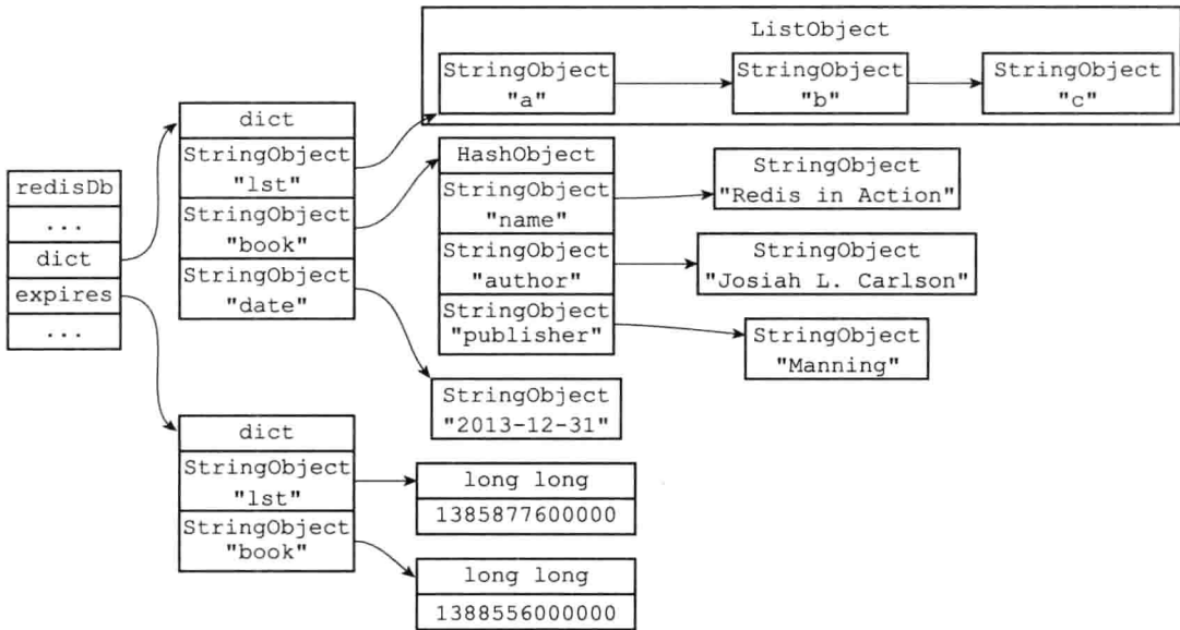
图 17-22 节点 7000 的数据库
