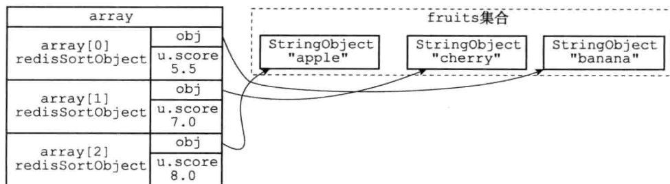
图 21-11 根据 u.score 属性进行排序之后的数组
