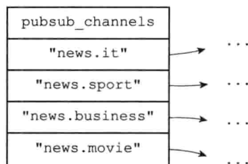
图 18-18 pubsub_channels 字典示例
