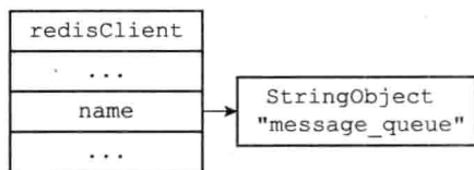
图 13-3 name 属性示例
