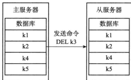
图 15-5 主服务器向从服务器发送命令
