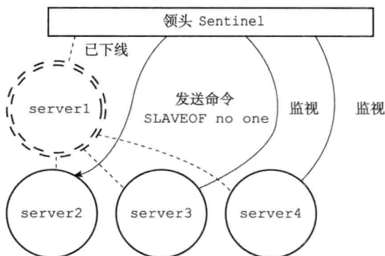
图 16-22 将 server2 升级为主服务器
