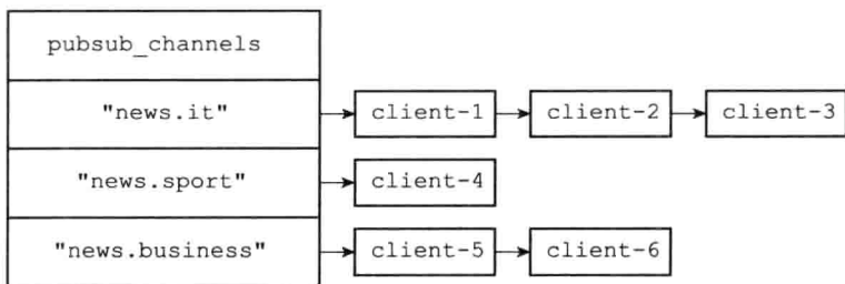
图 18-9 执行 UNSUBSCRIBE 之后的 pubsub_channels 字典
