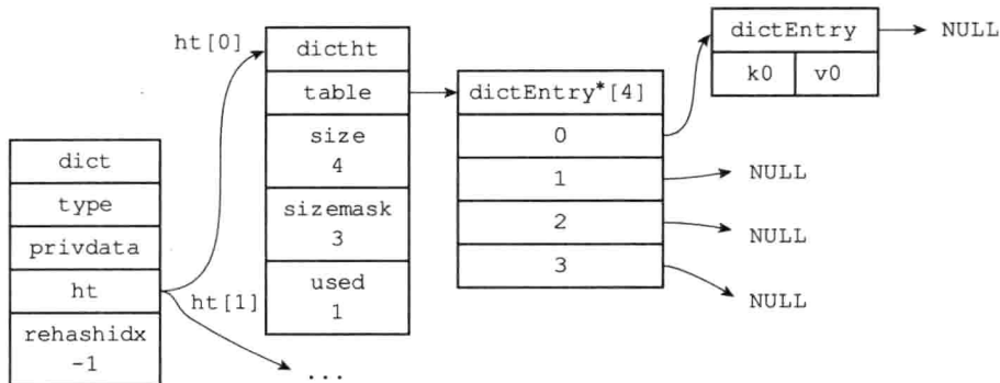
图 4-5 添加键值对 k_0 和 v_0 之后的字典
