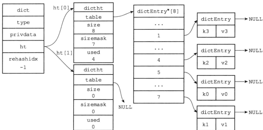
图 4-17 rehash 执行完毕
