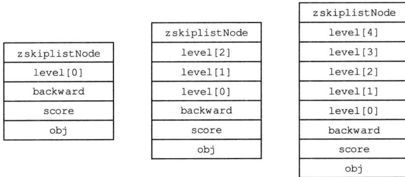
图 5-2 带有不同层高的节点
