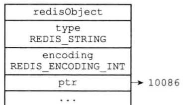
图 8-1 int 编码的字符串对象
