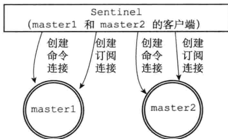
图 16-8 Sentinel 向主服务器创建网络连接
