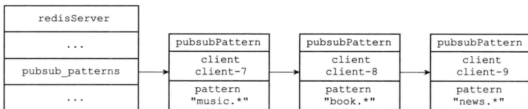
图 18-11 pubsub_patterns 链表示例
