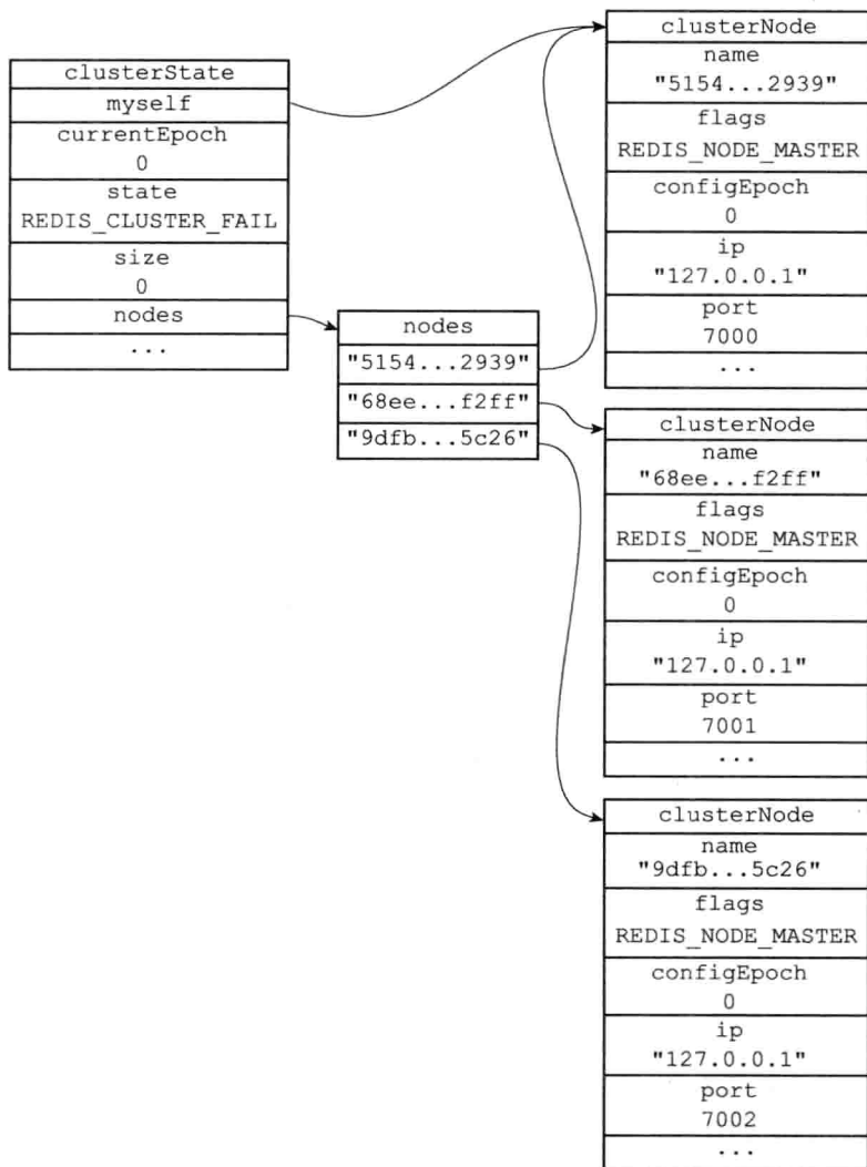
图 17-7 节点 7000 创建的 clusterState 结构
