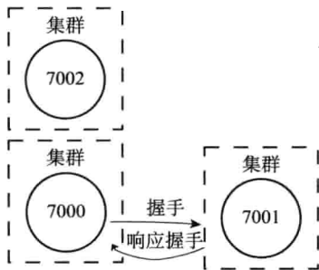
图 17-2 节点 7000 和 7001 进行握手
