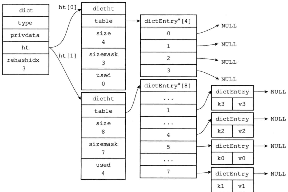
图 4-16 rehash 索引 3 上的键值对
