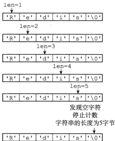
图 2-4 计算 C 字符串长度的过程
