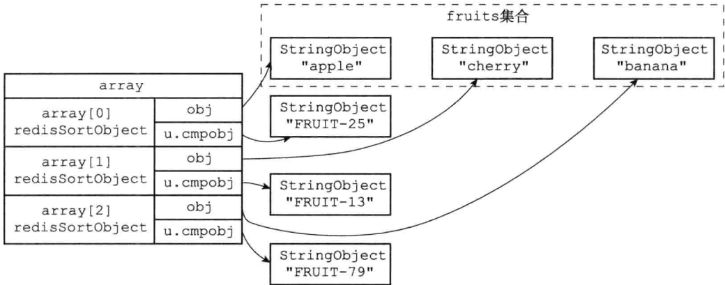
图 21-13 将 u.cmpobj 指针指向权重键
