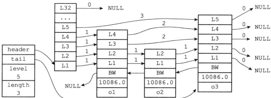
图 5-7 三个带有相同分值的跳跃表节点
