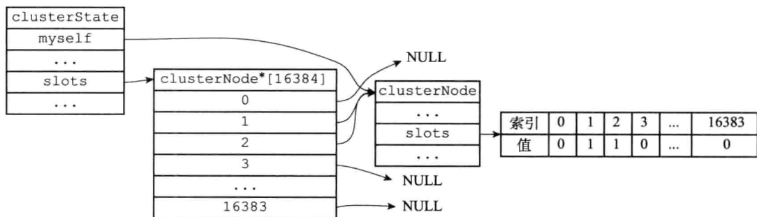
图 17-17 执行 CLUSTER ADDSLOTS 命令之后的 clusterState 结构
