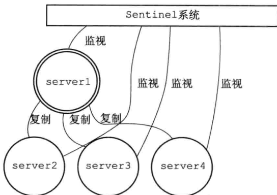
图 16-1 服务器与 Sentinel 系统
