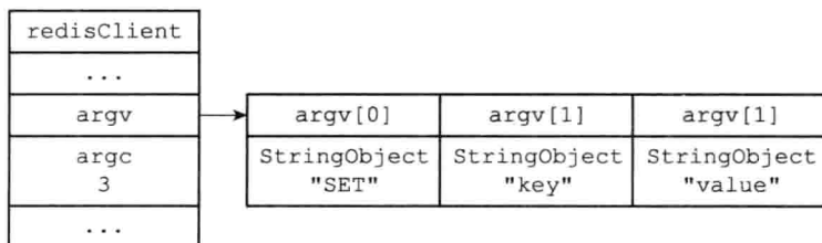
图 13-5 argv 属性和 argc 属性示例
