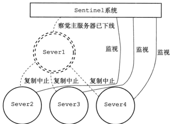
图 16-2 主服务器下线
