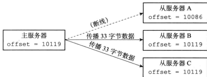
图 15-9 因为断线而处于不一致状态的从服务器 A
