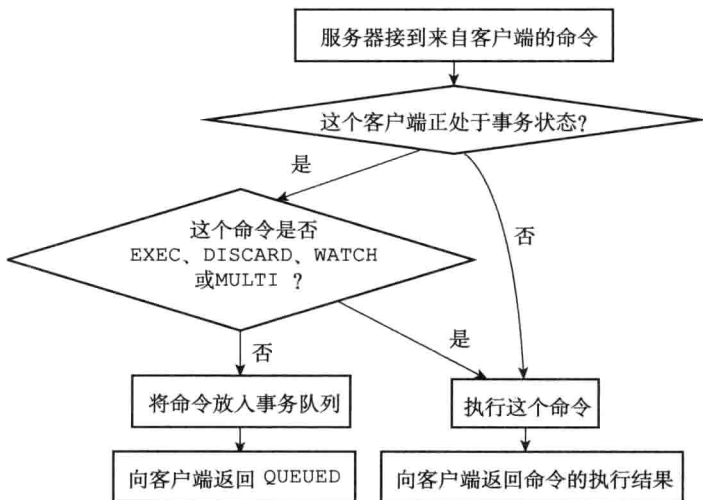
图 19-1 服务器判断命令是该入队还是该执行的过程
