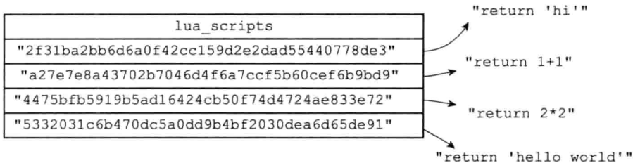
图 20-11 lua_scripts 字典
