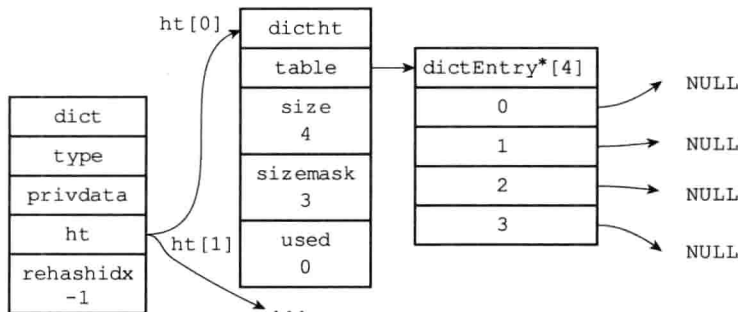
图 4-4 空字典
