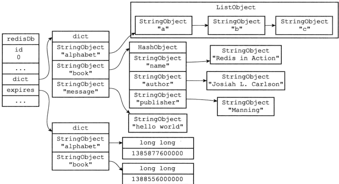
图 11-3 一个数据库
