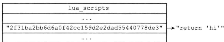
图 20-7 lua_scripts 字典
