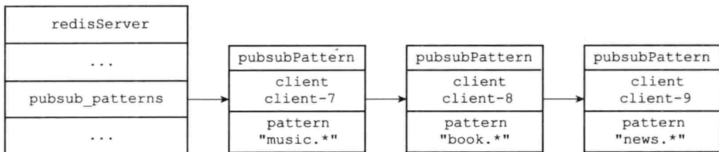
图 18-20 pubsub_patterns 链表
