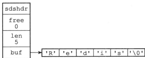
图 2-1 SDS 示例
