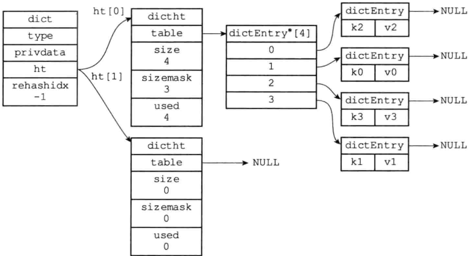
图 4-8 执行 rehash 之前的字典
