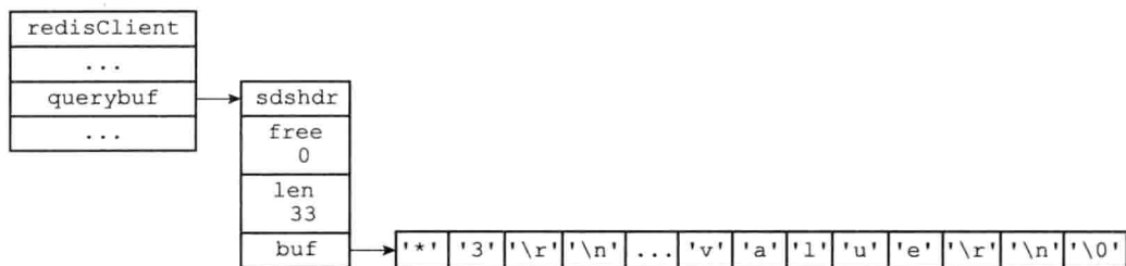
图 13-4 querybuf 属性示例
