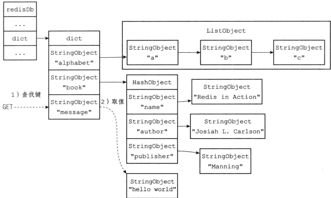
图 9-9 使用 GET 命令取值的过程
