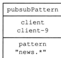
图 18-10 pubsubPattern 结构示例
