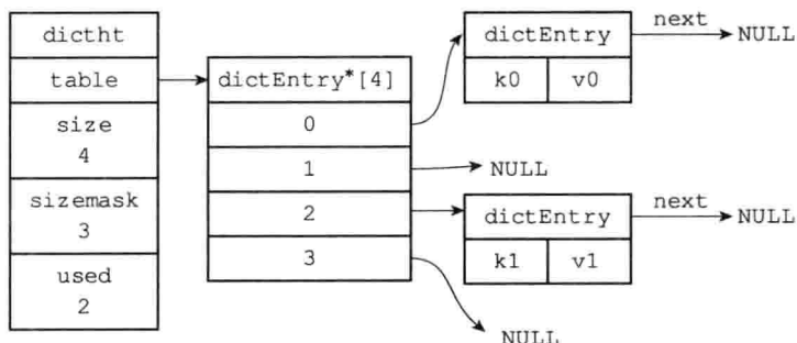
图 4-6 一个包含两个键值对的哈希表
