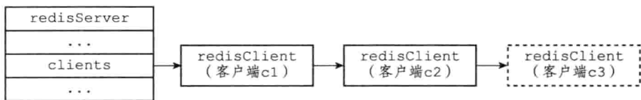
图 13-12 服务器状态结构的 clients 链表
