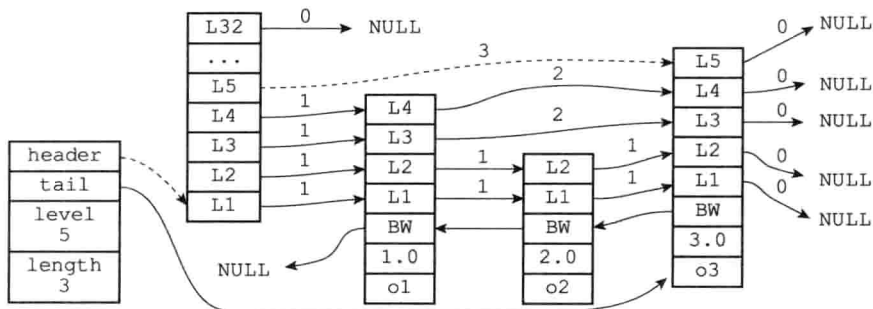
图 5-4 计算节点的排位
