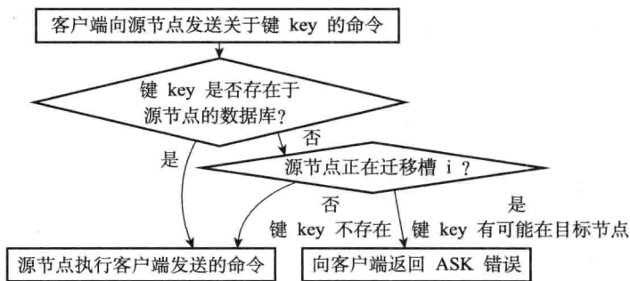
图 17-26 判断是否发送 ASK 错误的过程
