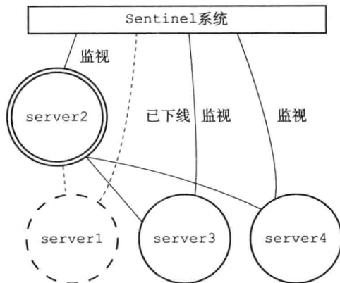
图 16-26 server1 被设置为新主服务器的从服务器
