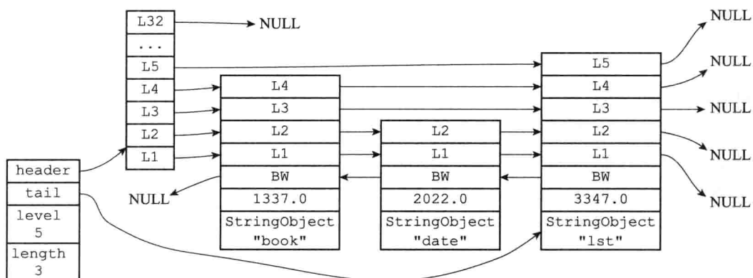
图 17-23 节点 7000 的 slots_to_keys 跳跃表
