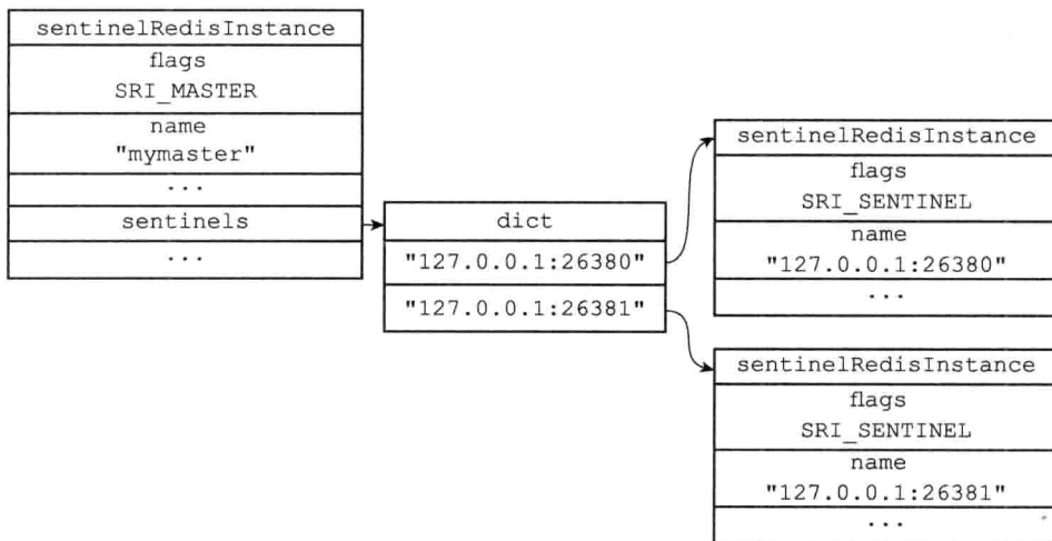
图 16-15 主服务器实例结构中的 sentinels 字典
