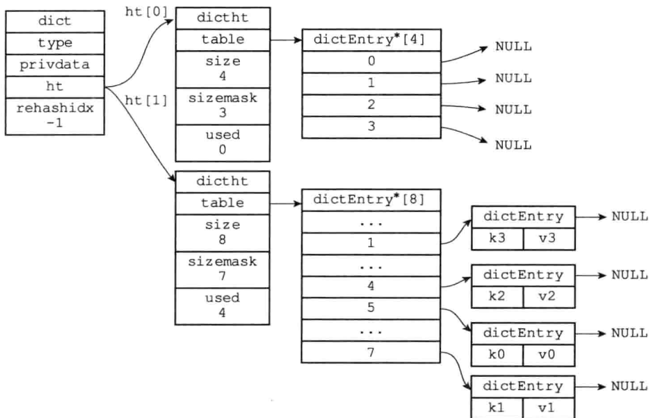
图 4-10 ht[0] 的所有键值对都已经被迁移到 ht[1]
