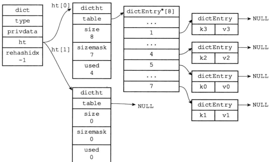
图 4-11 完成 rehash 之后的字典
