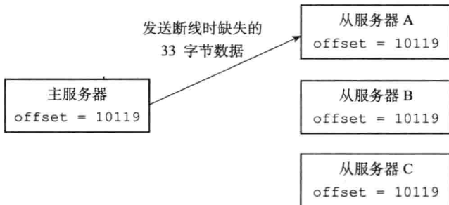
图 15-11 主服务器向从服务器发送缺失的数据
