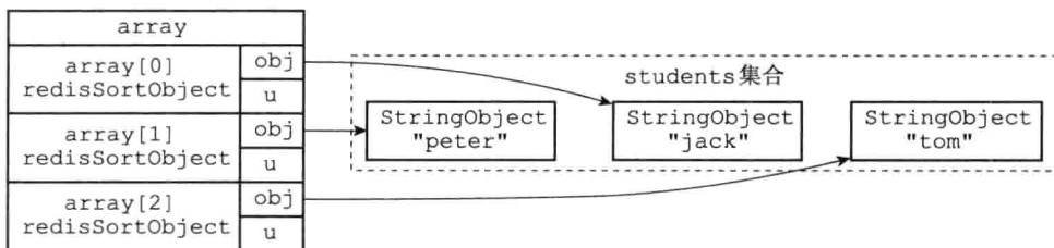
图 21-19 排序之后的数组
