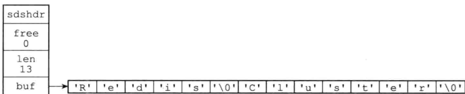
图 2-18 保存了特殊数据格式的 SDS
