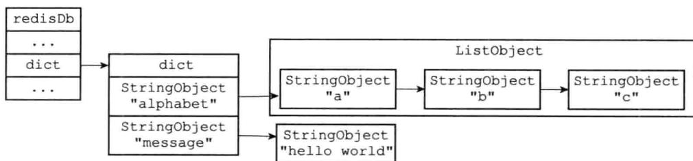
图 9-6 删除 book 键之后的键空间
