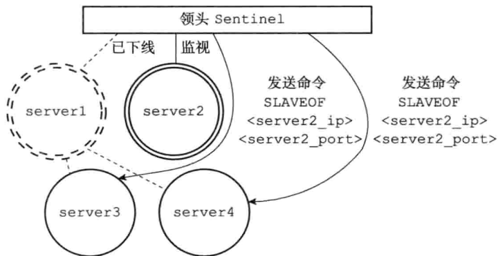
图 16-24 让从服务器复制新的主服务器
