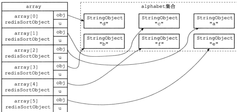
图 21-15 将 obj 指针指向集合的各个元素
