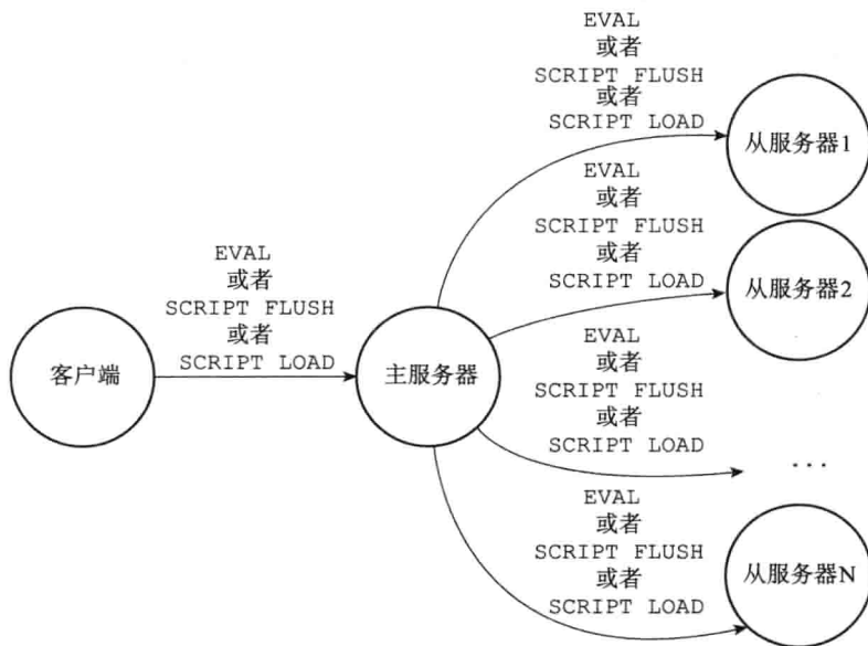
图 20-9 将脚本命令传播给从服务器
