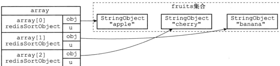
图 21-6 按集合元素进行排序后的数组
