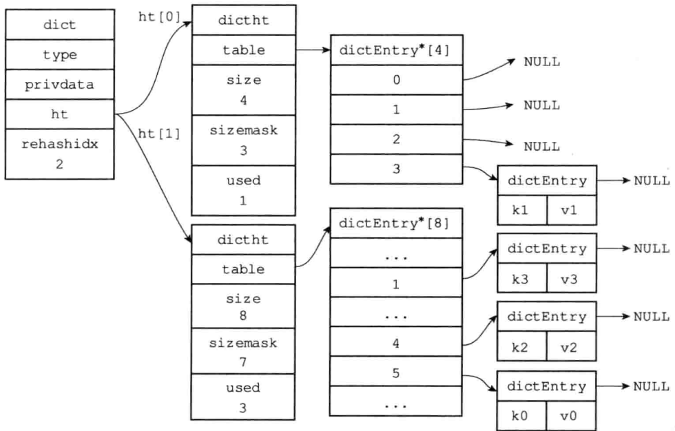
图 4-15 rehash 索引 2 上的键值对
