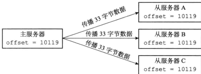
图 15-8 更新偏移量之后的主从服务器
