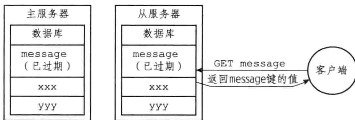
图 9-18 主从服务器删除过期键 (2)
