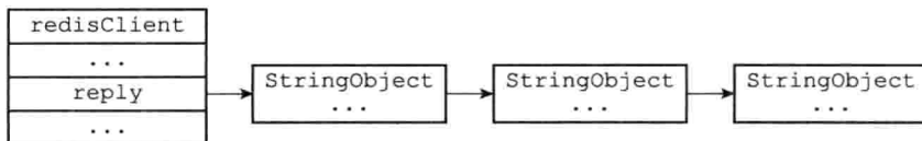
图 13-9 可变大小缓冲区示例
