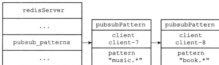
图 18-12 执行 PSUBSCRIBE 命令之前的 pubsub_patterns 链表
