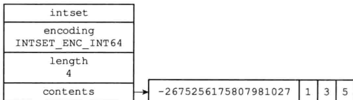
图 6-2 一个包含四个 int64_t 类型整数的整数集合
