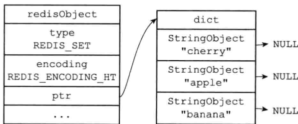
图 8-13 hashtable 编码的 fruits 集合对象
