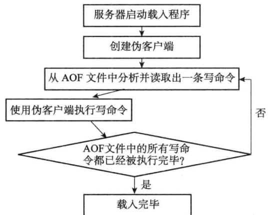
图 11-2 AOF 文件载入过程
