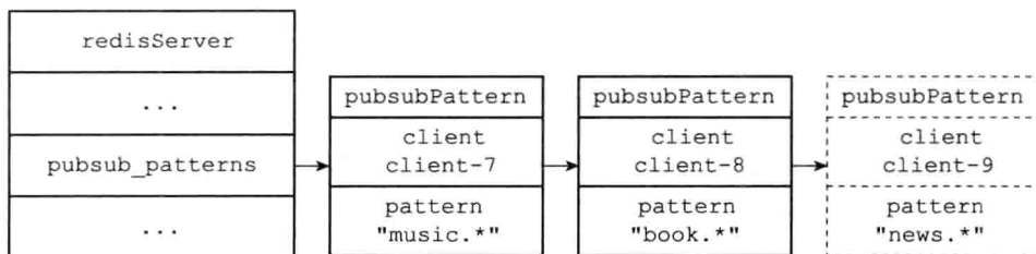
图 18-13 执行 PSUBSCRIBE 命令之后的 pubsub_patterns 链表
