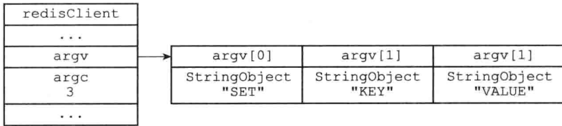
图 14-3 客户端状态的 argv 属性和 argc 属性
