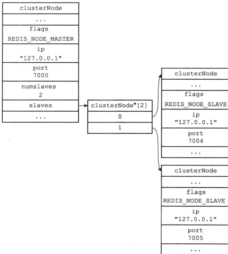
图 17-36 集群中的各个节点为节点 7000 创建的 clusterNode 结构
