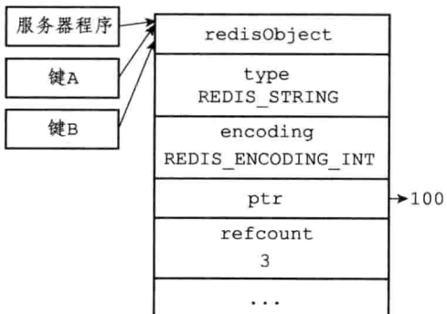
图 8-23 引用数为 3 的共享对象
