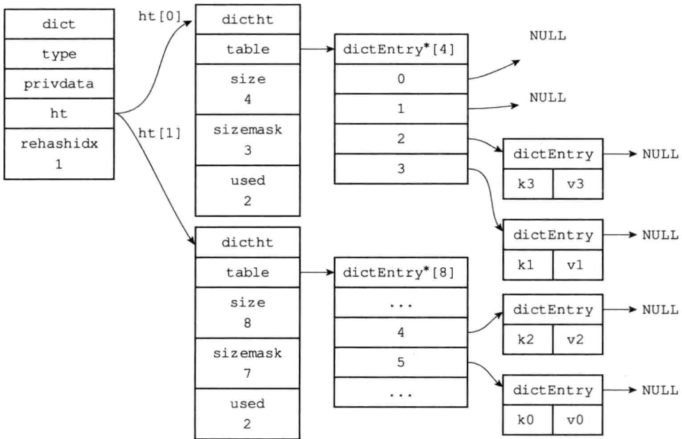
图 4-14 rehash 索引 1 上的键值对
