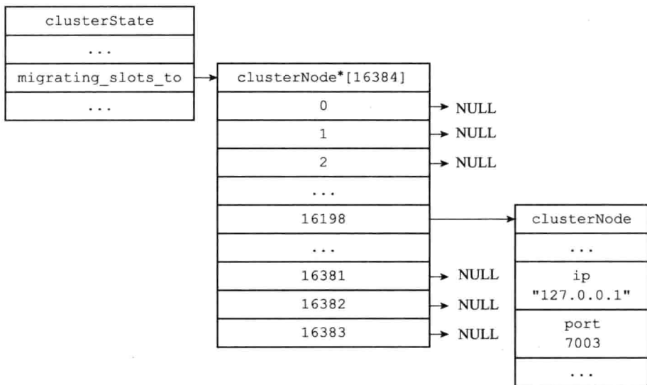
图 17-28 节点 7002 的 migrating_slots_to 数组
