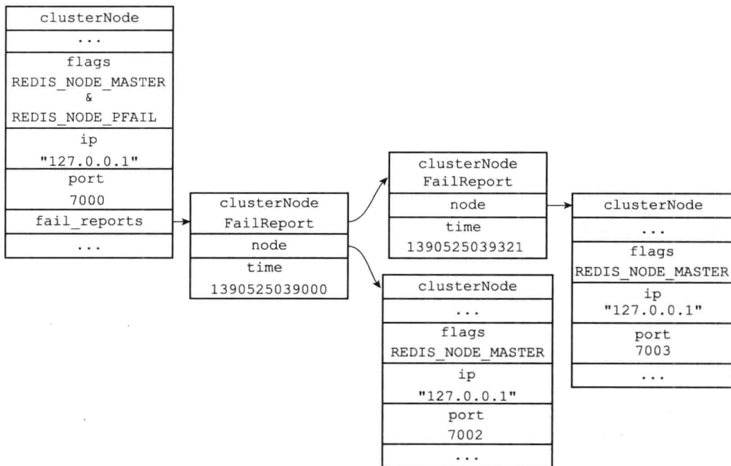
图 17-38 节点 7000 的下线报告
