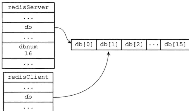
图 9-2 客户端的目标数据库为 1 号数据库
