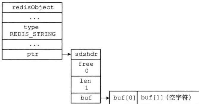
图 22-1 SDS 表示的位数组
