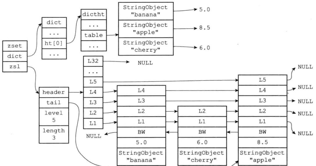
图 8-16 skiplist 编码的有序集合对象
