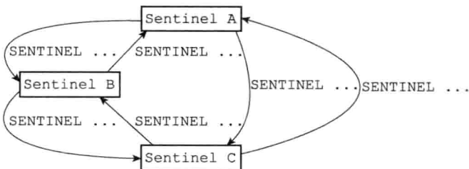
图 16-21 Sentinel 再次向其他 Sentinel 发送命令
