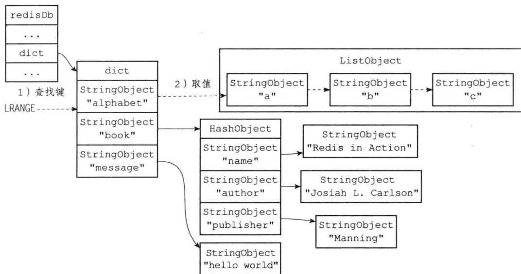
图 9-10 使用 LRANGE 命令取值的过程
