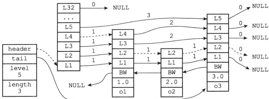
图 5-3 遍历整个跳跃表
