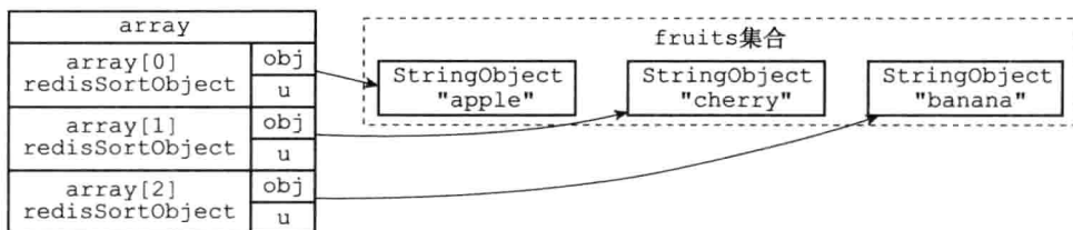
图 21-9 将 obj 指针指向集合的各个元素
