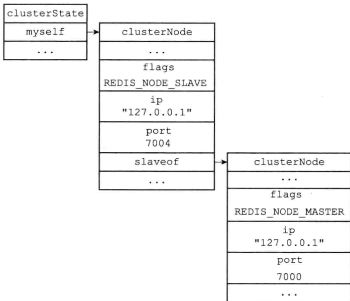
图 17-35 节点 7004 的 clusterState 结构
