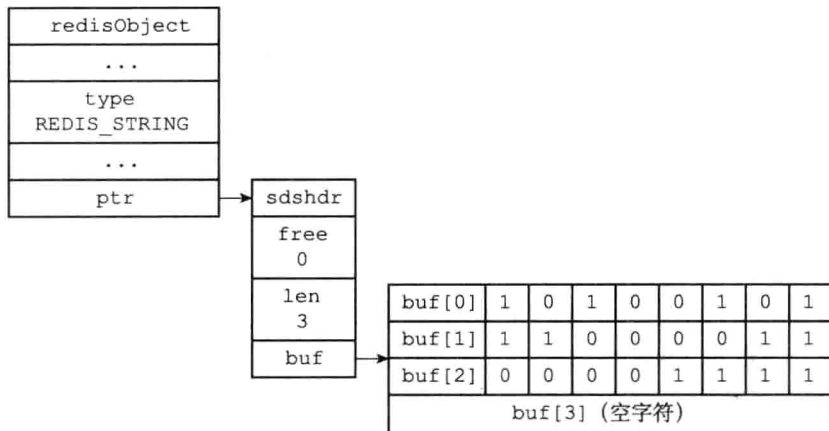
图 22-3 三字节长的位数组的 SDS 表示
