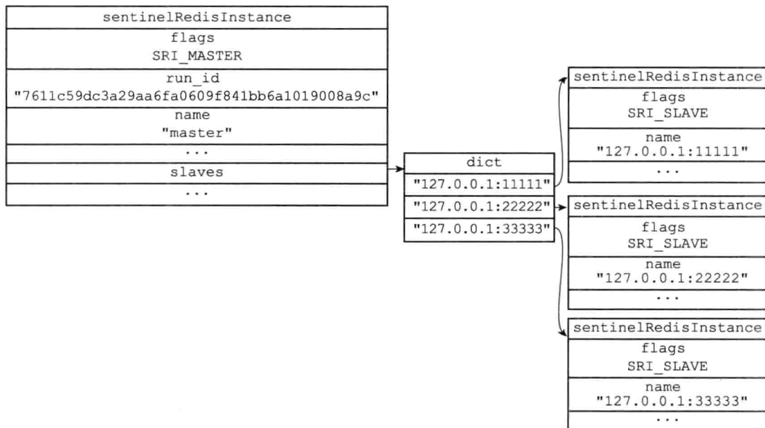
图 16-10 主服务器和它的三个从服务器
