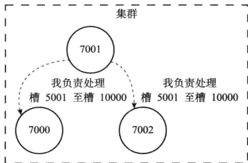
图 17-12 7001 告知 7000 和 7002 自己负责处理的槽
