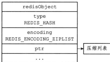
图 8-9 ziplist 编码的 profile 哈希对象
