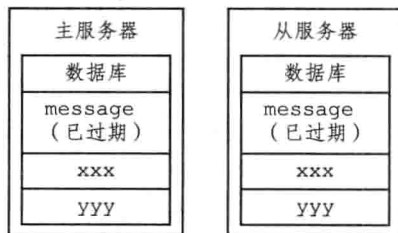
图 9-17 主从服务器删除过期键（1）
