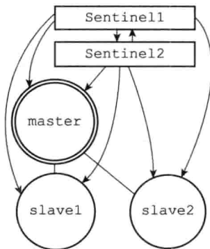
图 16-17 Sentinel 向实例发送 PING 命令
