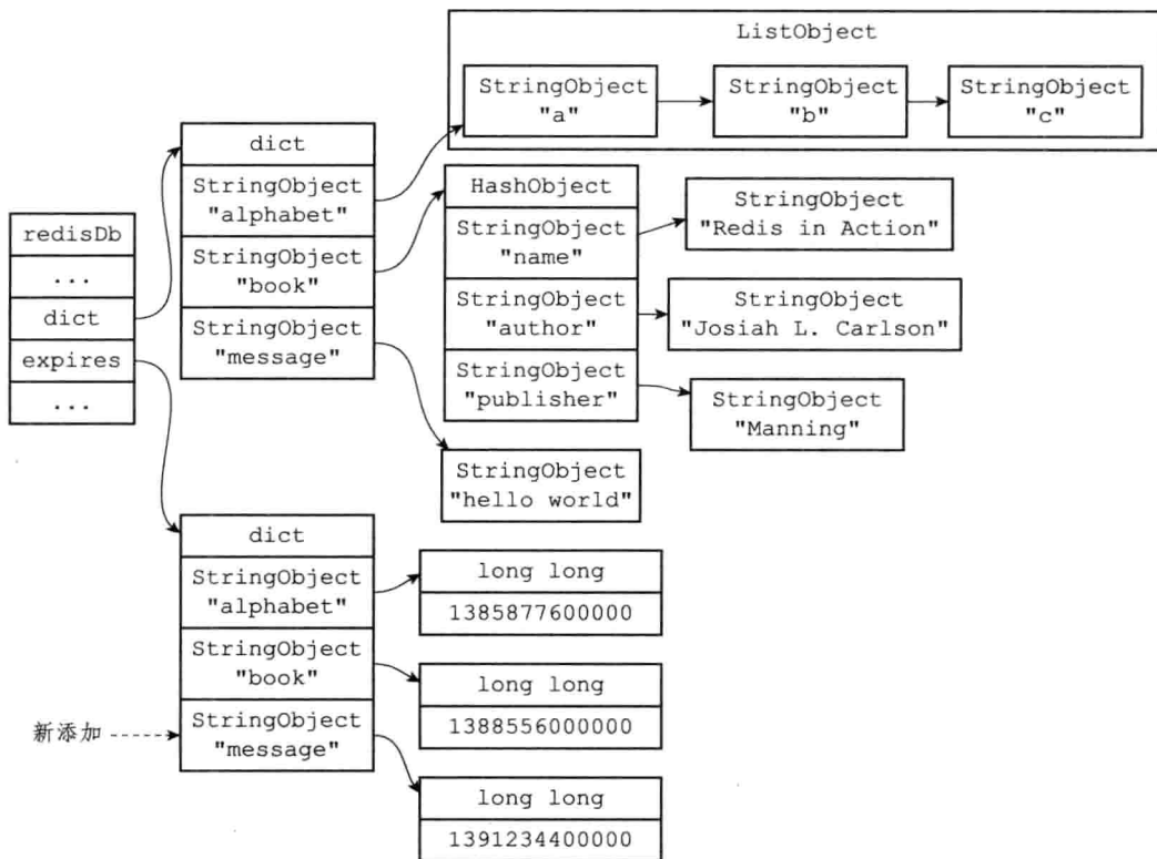
图 9-13 执行 PEXPIREAT 命令之后的数据库
