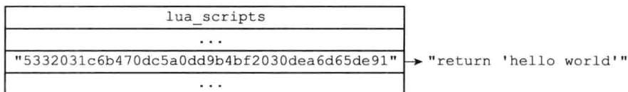
图 20-5 添加新键值对之后的 lua_scripts 字典
