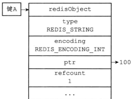
图 8-20 未被共享的字符串对象
