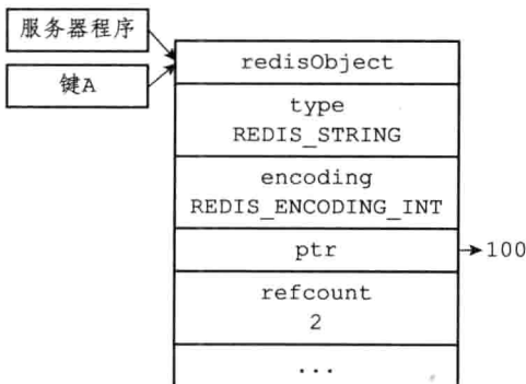
图 8-22 引用数为 2 的共享对象
