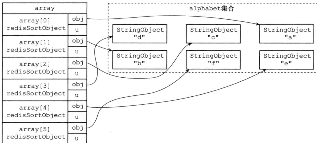
图 21-16 排序后的数组
