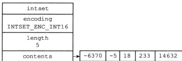
图 6-1 一个包含五个 int16_t 类型整数的整数集合
