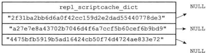
图 20-10 一个 repl_scriptcache_dict 字典示例
