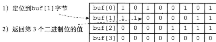
图 22-5 查找并返回 offset 为 10 的二进制位的过程
