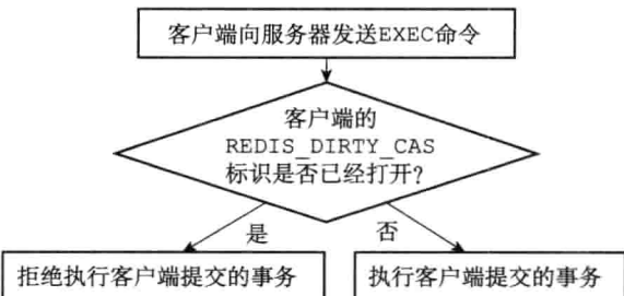
图 19-6 服务器判断是否执行事务的过程
