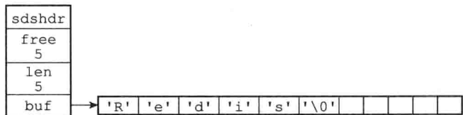
图 2-2 带有未使用空间的 SDS 示例
