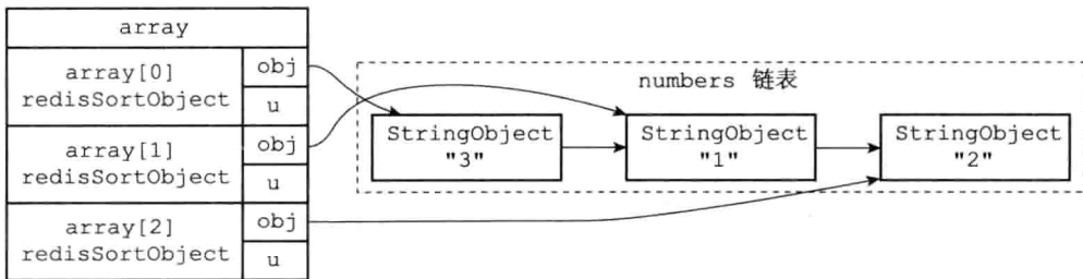
图 21-2 将 obj 指针指向列表的各个项
