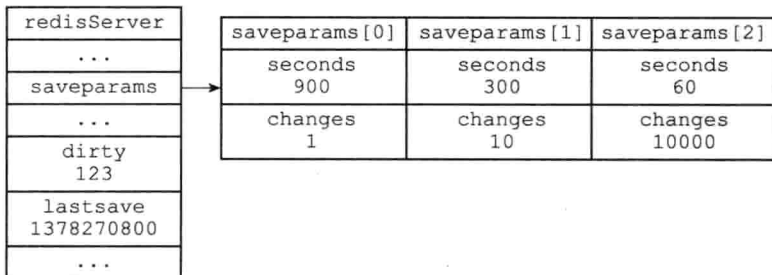
图 10-8 服务器状态
