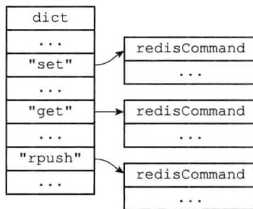
图 13-6 命令表
