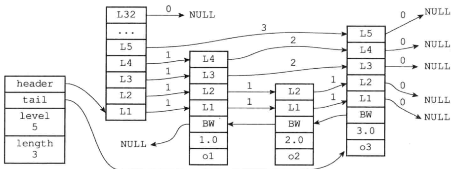
图 5-1 一个跳跃表
