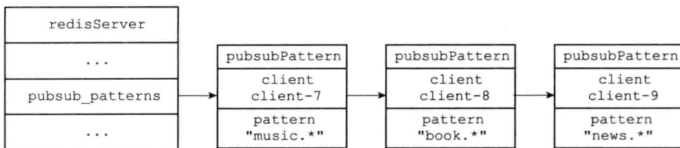
图 18-17 pubsub_patterns 链表
