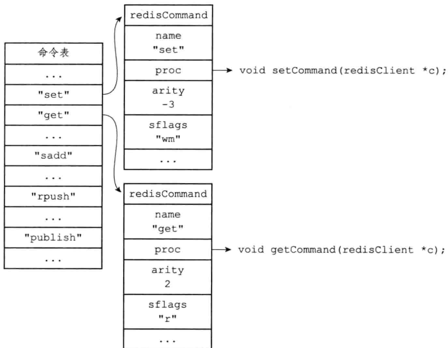
图 14-4 命令表
