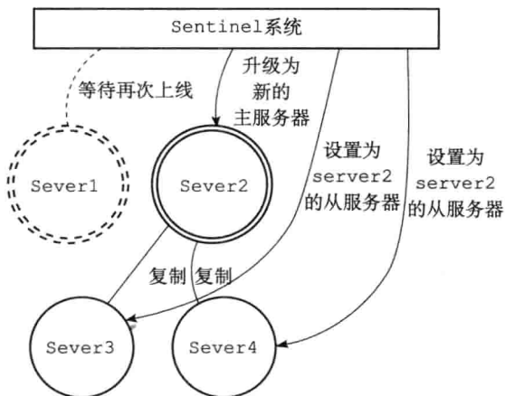
图 16-3 故障转移
