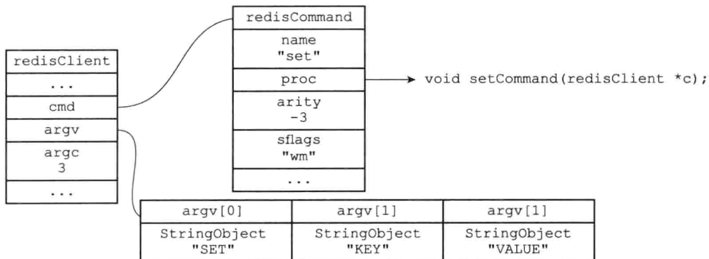
图 14-6 客户端状态
