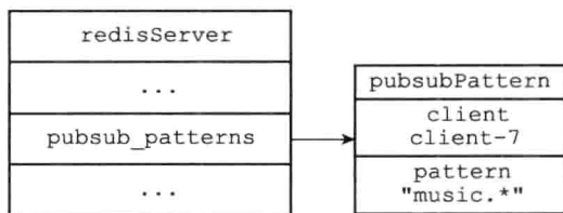
图 18-21 pubsub_patterns 链表
