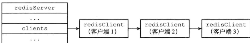
图 13-2 clients 链表
