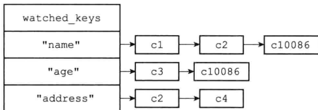
图 19-5 watched_keys 字典
