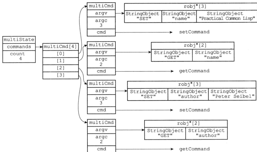
图 19-2 事务状态
