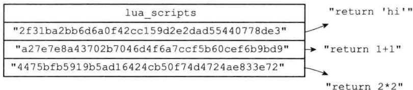
图 20-6 lua_scripts 字典
