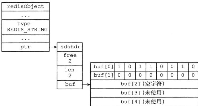
图 22-8 扩展空间之后的位数组
