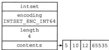
图 6-12 删除 4 294 967 295 的整数集合
