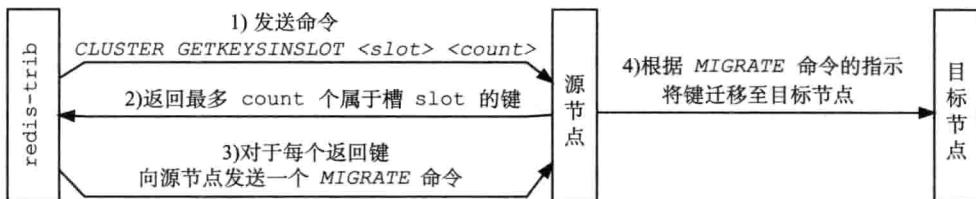
图 17-24 迁移键的过程
