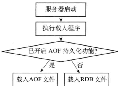
图 10-4 服务器载入文件时的判断流程
