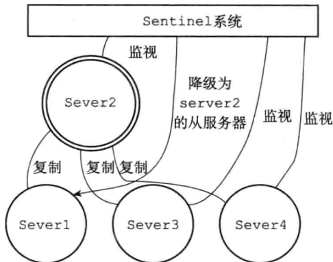
图 16-4 原来的主服务器被降级为从服务器
