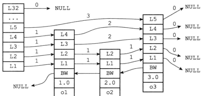
图 5-8 由多个跳跃节点组成的跳跃表
