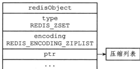
图 8-14 ziplist 编码的有序集合对象
