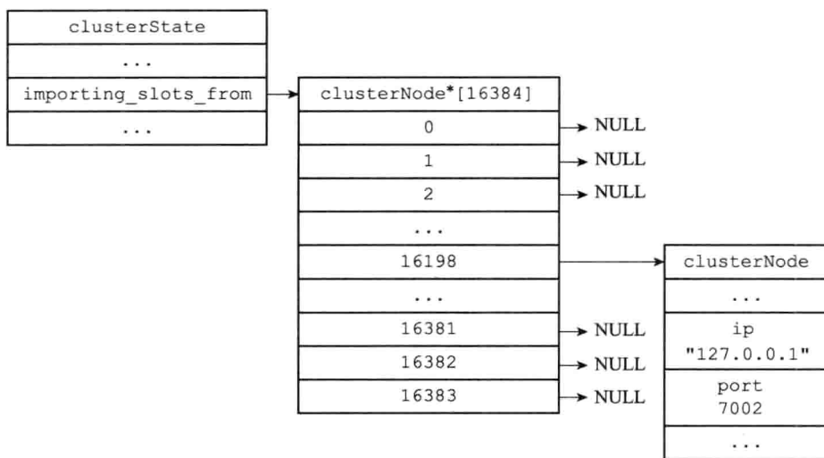
图 17-27 节点 7003 的 importing_slots_from 数组
