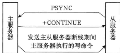
图 15-6 主从服务器执行部分重同步的过程
