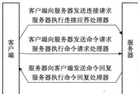
图 12-7 客户端和服务器的通信过程
