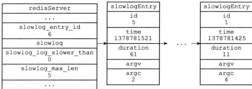
图 23-2 redisServer 结构示例
