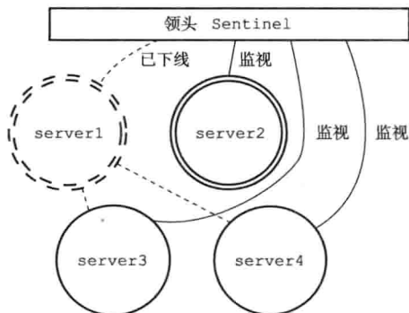
图 16-23 server2 成功升级为主服务器
